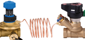
DPCV: ASV-PV+ASV-BD
