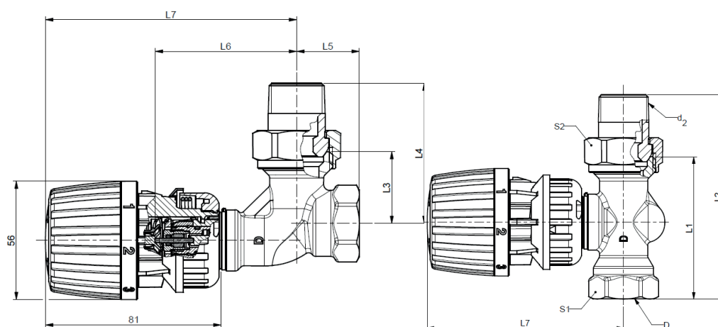
RA-DV Droit et équerre / tête RA 2990 sensor
