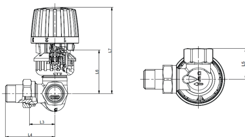
RA-DV versione a squadra/ diritta+ sensore RA 2990
