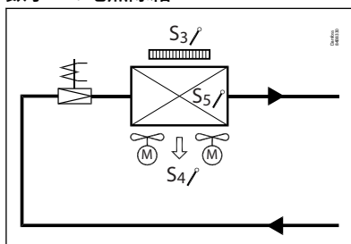
数字 14: 电热除霜
