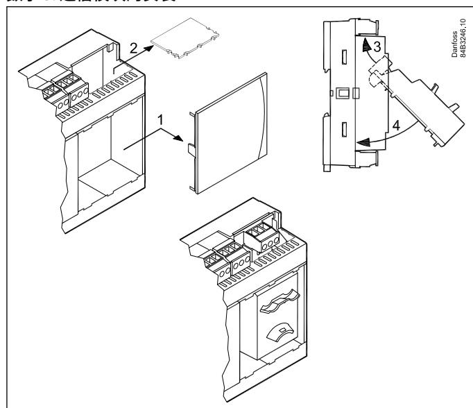
数字 3: 通信模块的安装
