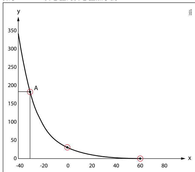
数字 13: NTC 传感器的传感器点示例
