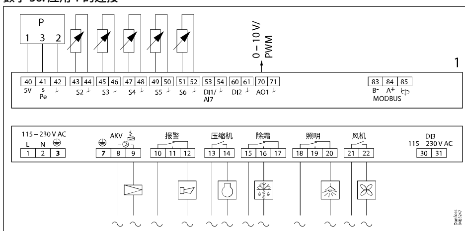
数字 37: 应用 2 的连接
