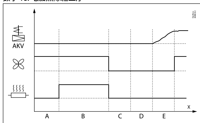
数字 18: 电加热除霜工序
