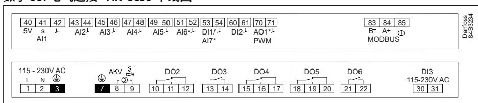
数字 35: 电气连接 - AK-CC55 单线圈
