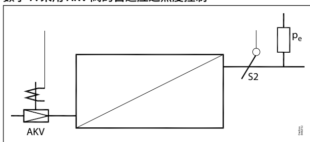
数字 7: 采用 AKV 阀的自适应过热度控制
