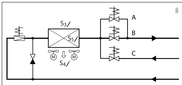
数字 15: 热气除霜
