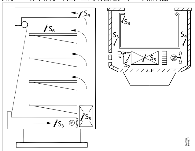
数字 32: 带一个蒸发器的背对背机柜
