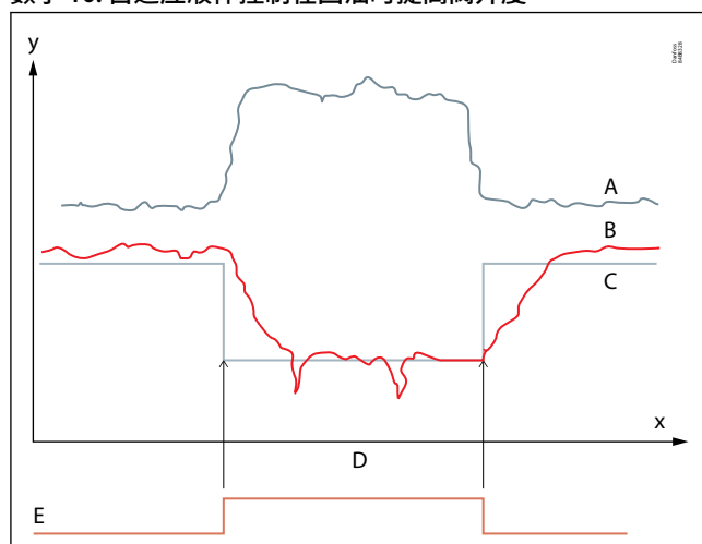
数字 10: 自适应液体控制在回油时提高阀开度
