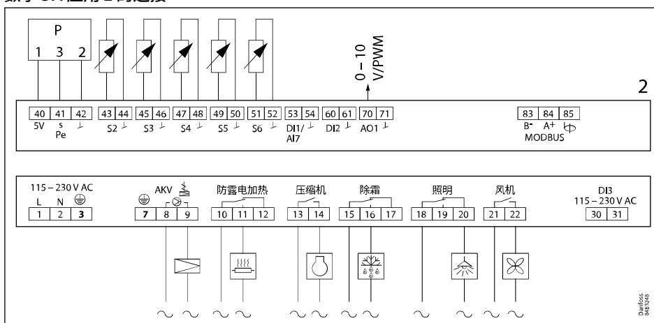
数字 37: 应用 2 的连接
