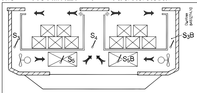
数字 33: 带两个蒸发器和一个 AKV 阀门的背对背机柜
