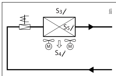
数字 16: 自然除霜
