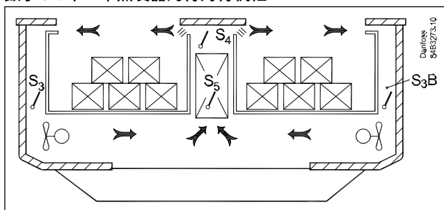
数字 32: 带一个蒸发器的背对背机柜
