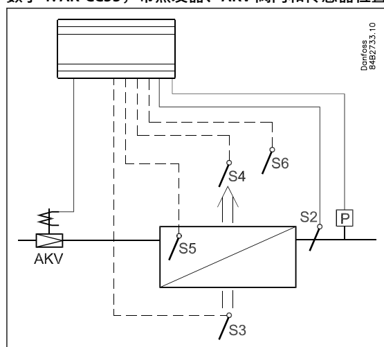
数字 1: AK-CC55，带蒸发器、AKV 阀门和传感器位置
