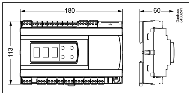
数字 60: AK-CC55 单线圈 UI
