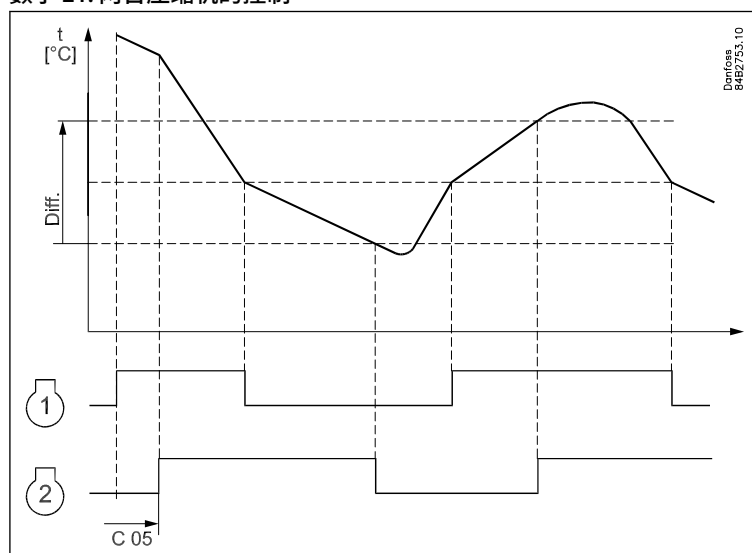
数字 21: 两台压缩机的控制
