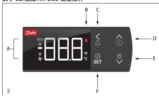
数字 52: 通过 AK-UI55 设定操作
