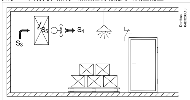
数字 34: 具有门和照明、加热控制功能的冷藏室配置
