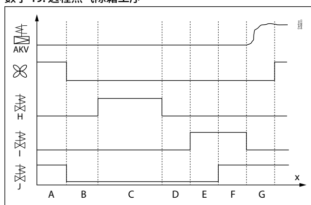
数字 19: 远程热气除霜工序
