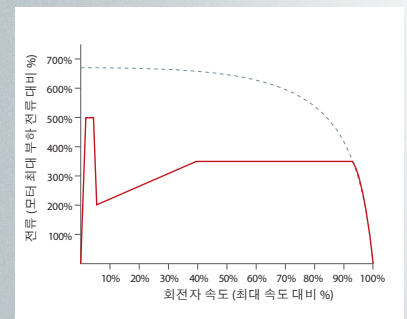
일정 전류/전류 가감속 - 킥스타트와 함께 이 그래프에 표시됨
