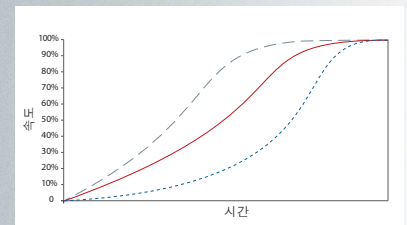
3가지의 적응형 가속 제어(AAC) 기동 프로파일 - 초기 가속, 일정 가속 및 지연 가속
