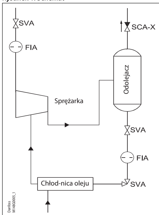
Rysunek 1: Schemat
