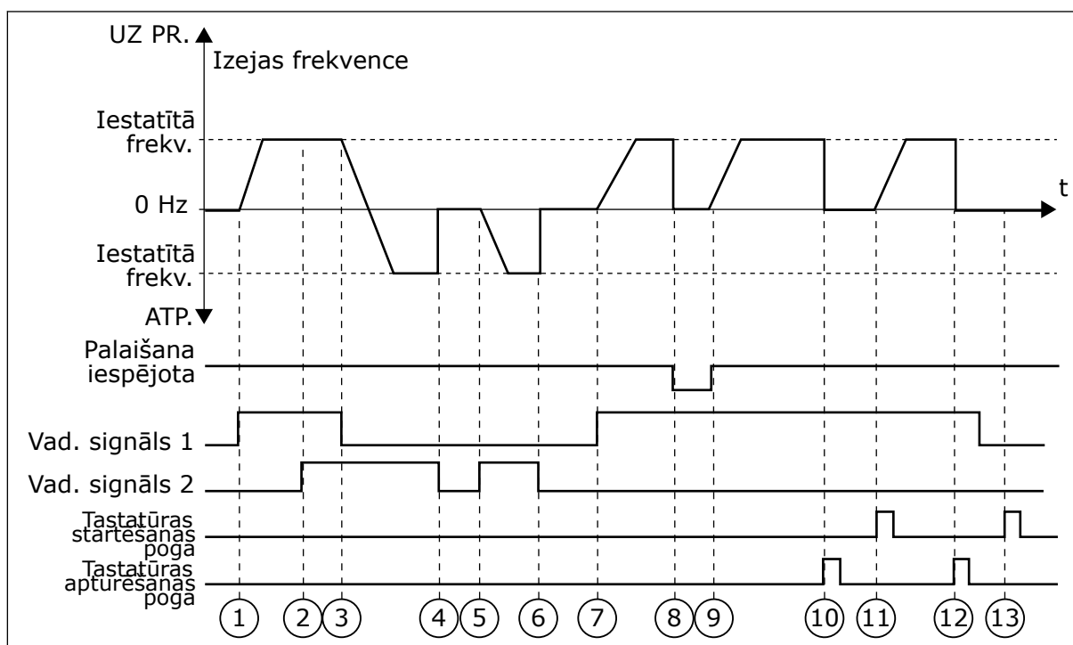
Att. 15: I/I A sākšanas/apturēšanas loģika = 0
