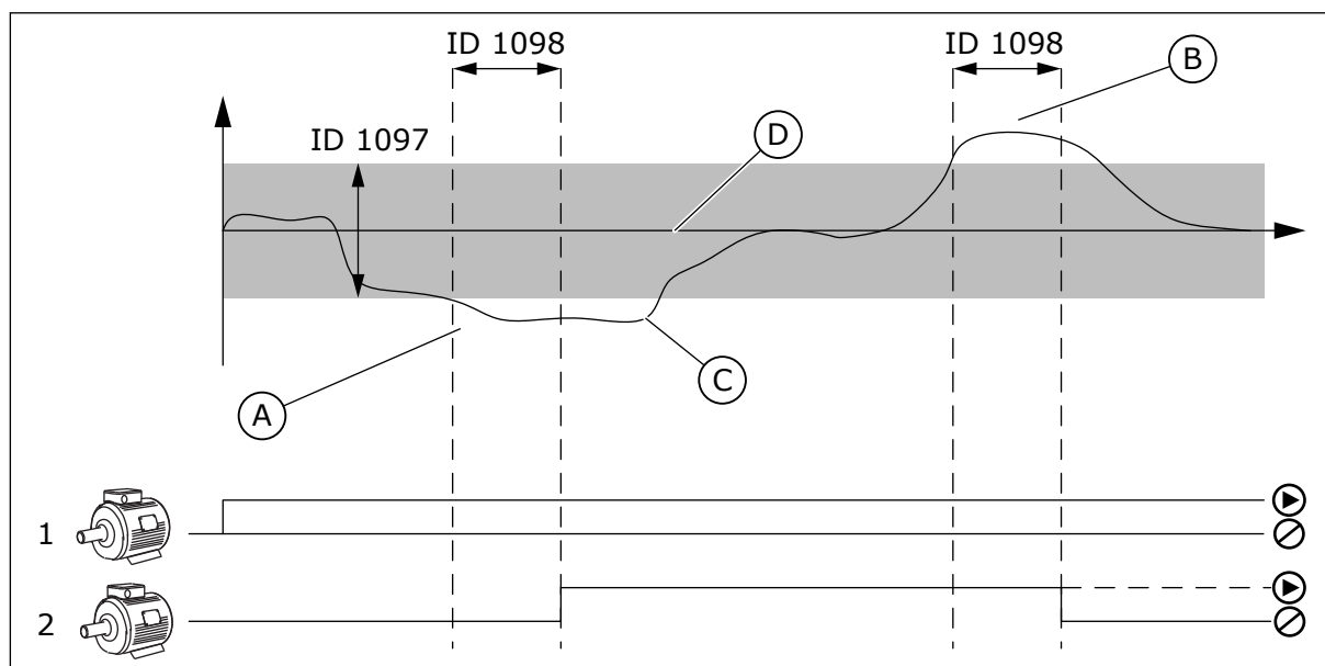
Att. 50: Papildu sūkņu sāksana vai apturēšana (P3.14.8 = joslas platums, P3.14.9 = joslas platuma aizkave)
