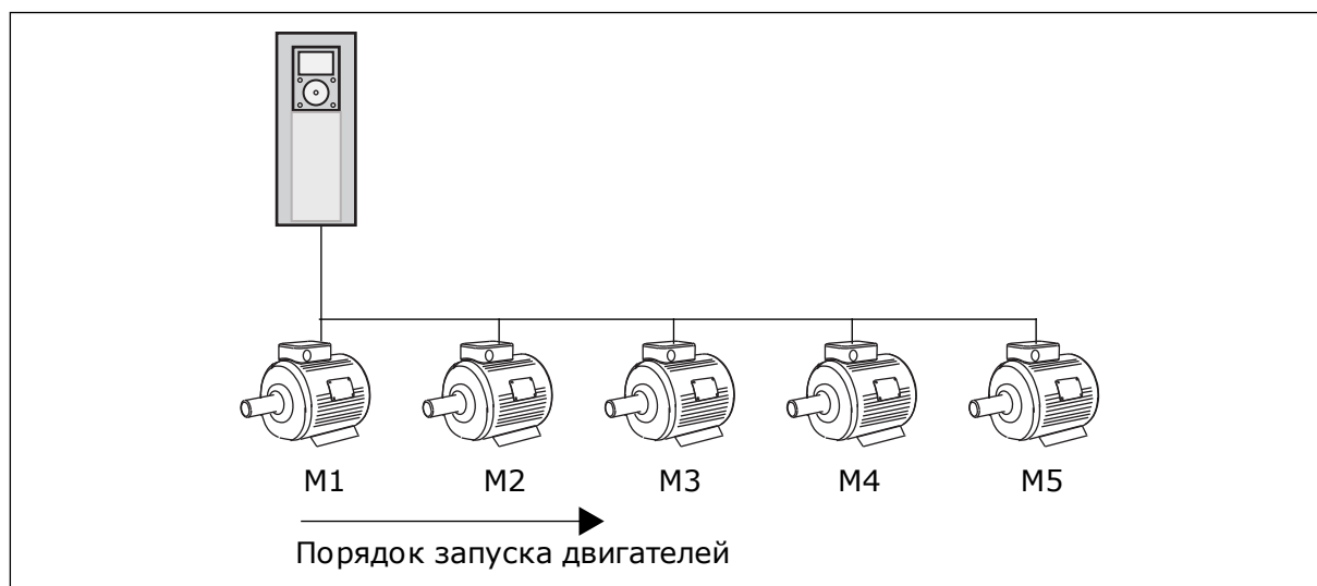
Рис. 45: Логика блокировки 1
