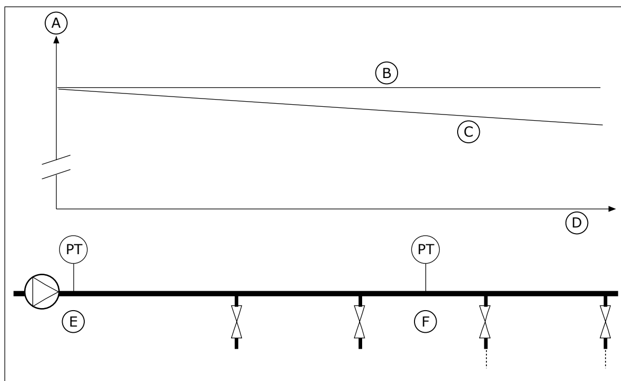
图 42: 压力传感器的位置
