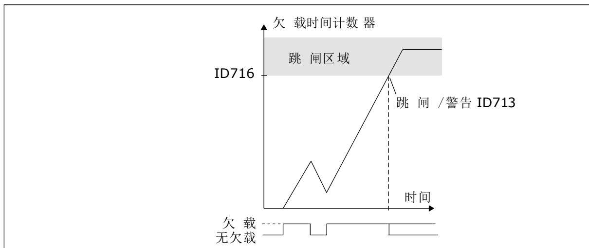
图 32: 欠载时间计数器功能
