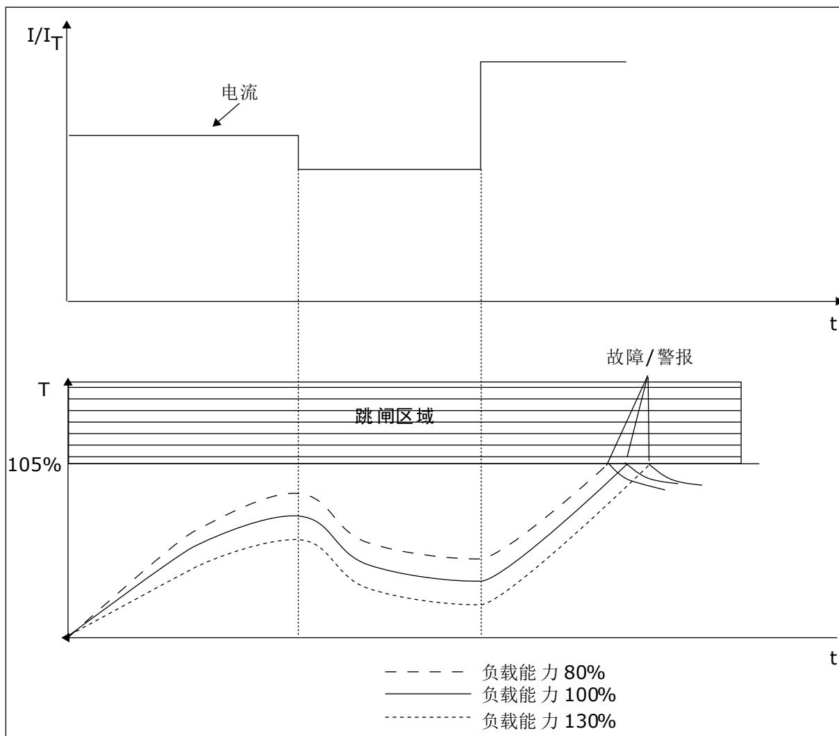
图 29: 电机温度的计算
