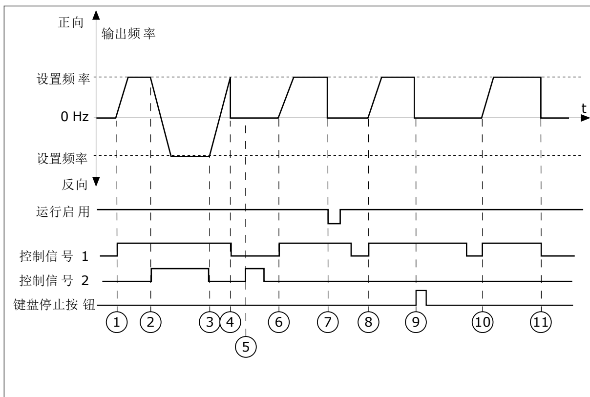
图 19: I/O A 启动/停止逻辑 = 4
