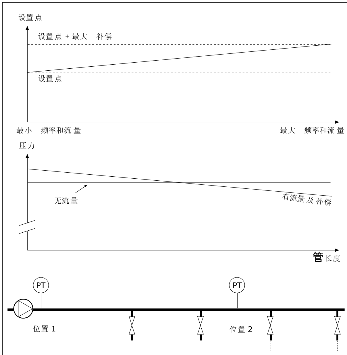
图 43: 压力损失补偿的启用设置点 1
