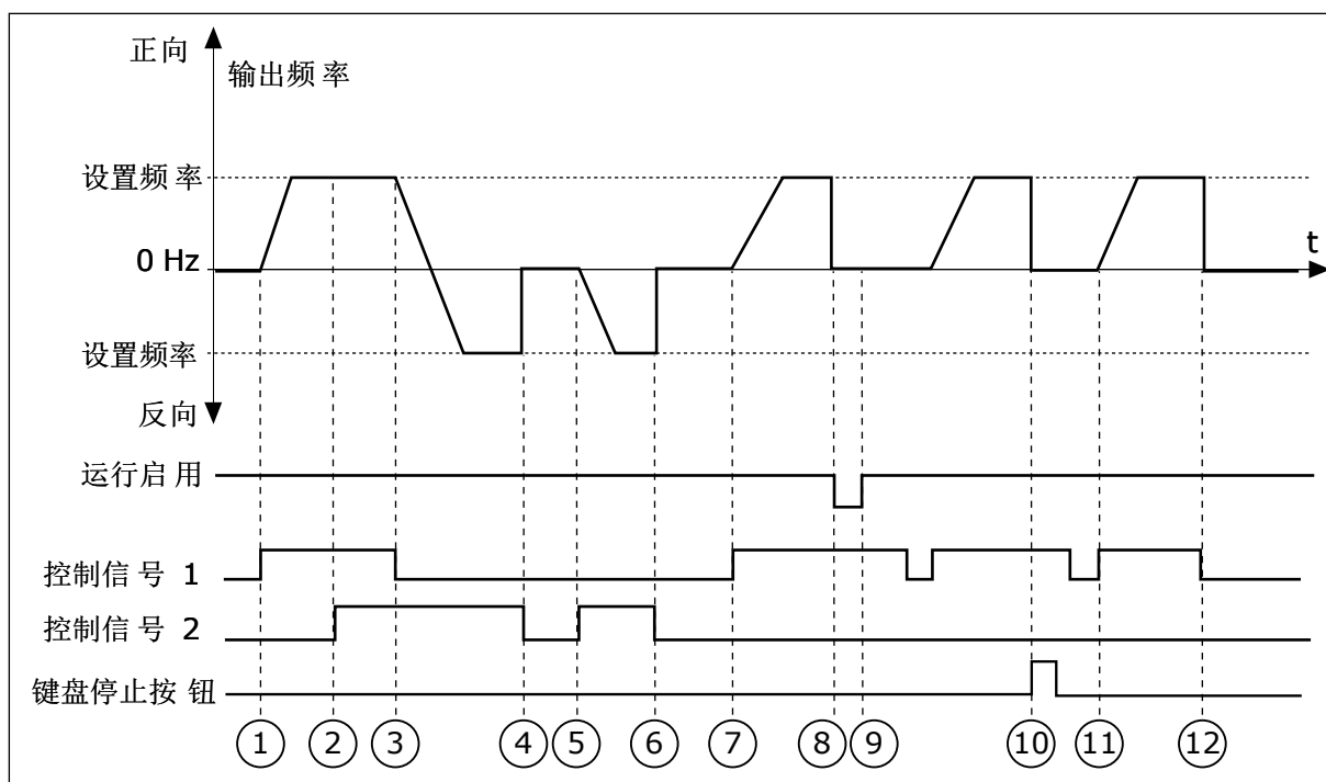
图 17: I/O A 启动/停止逻辑 = 2
