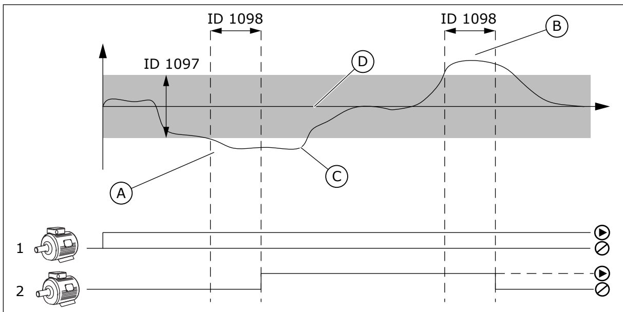
图 50: 辅助泵的启动或停止 ( P3.14.8 = 带宽 , P3.14.9 = 带宽延迟 )
