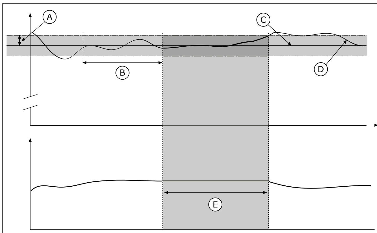
图 37: 死区功能
