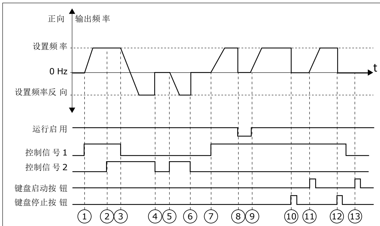
图 15: I/O A 启动/停止逻辑 = 0
