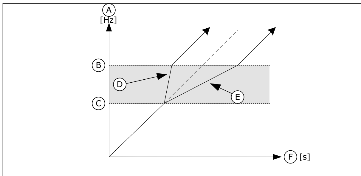
图 27: 斜坡时间因子参数
