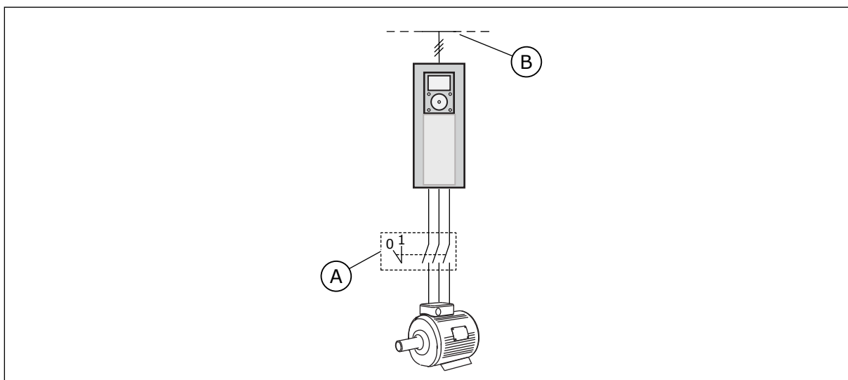
图 12: 变频器与电机之间的电机开关
