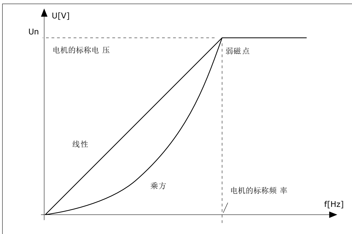
图 13: 电机电压的线性和乘方变化
