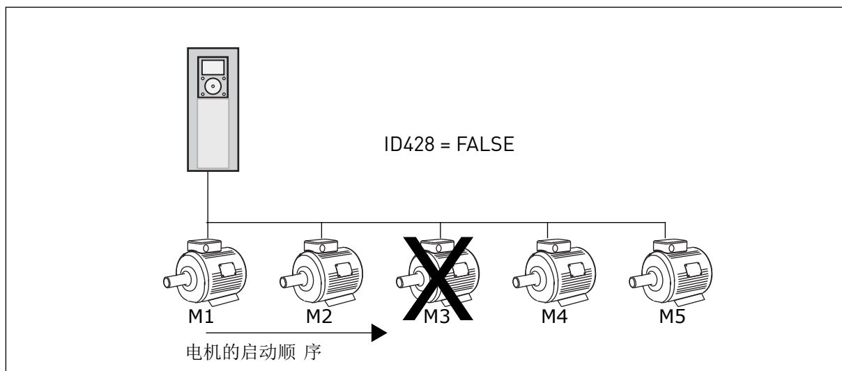
图 46: 互锁逻辑 2
