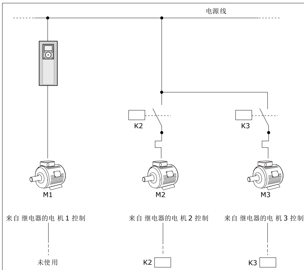
图 48: 选择 0
