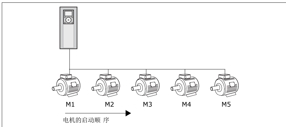
图 45: 互锁逻辑 1
