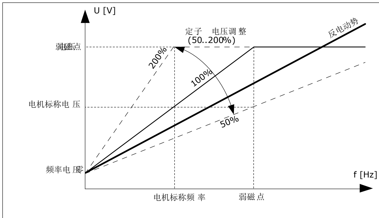
图 14: 定子电压调整
