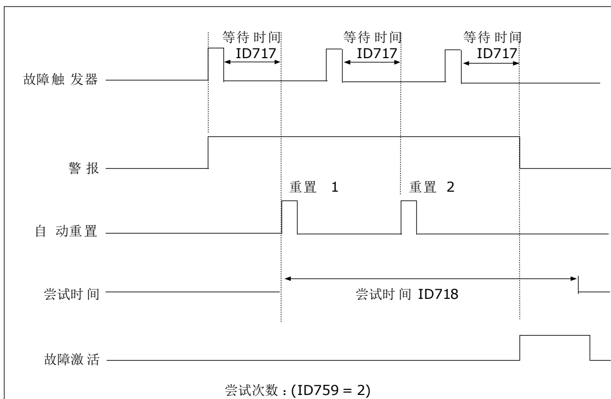
图 33: 自动重置功能
