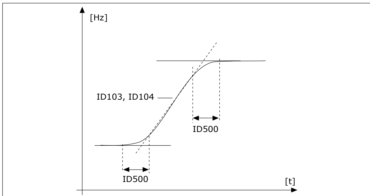
图 21: 加速/减速曲线 ( S 形 )
