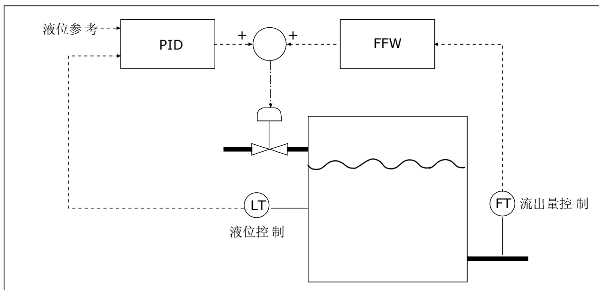
图 40: 前馈控制
