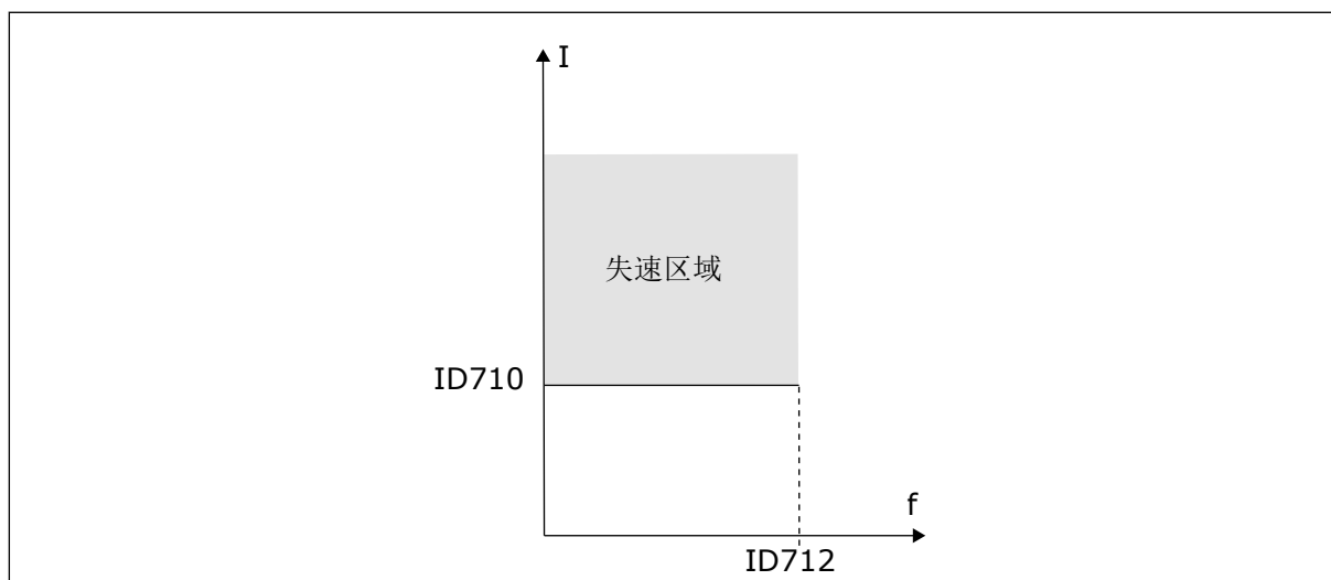
图 30: 失速特征设置
