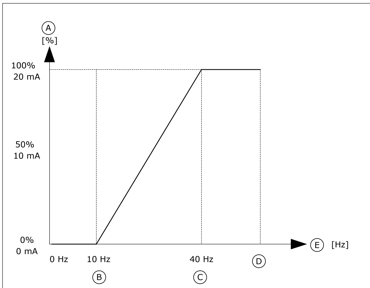
图 25: A01 信号的缩放
