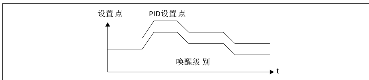
图 39: 唤醒模式：相对设置点
