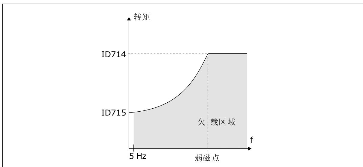
图 31: 设置最小负载
