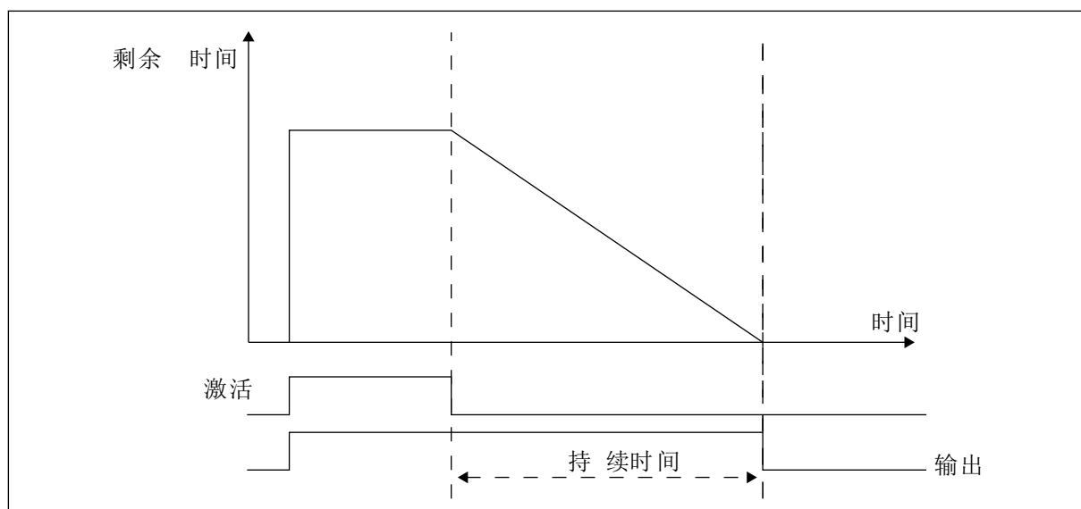
图 35: 激活信号来自数字输入或虚拟数字输入，例如时间通道。定时器从下降沿往下计数。
