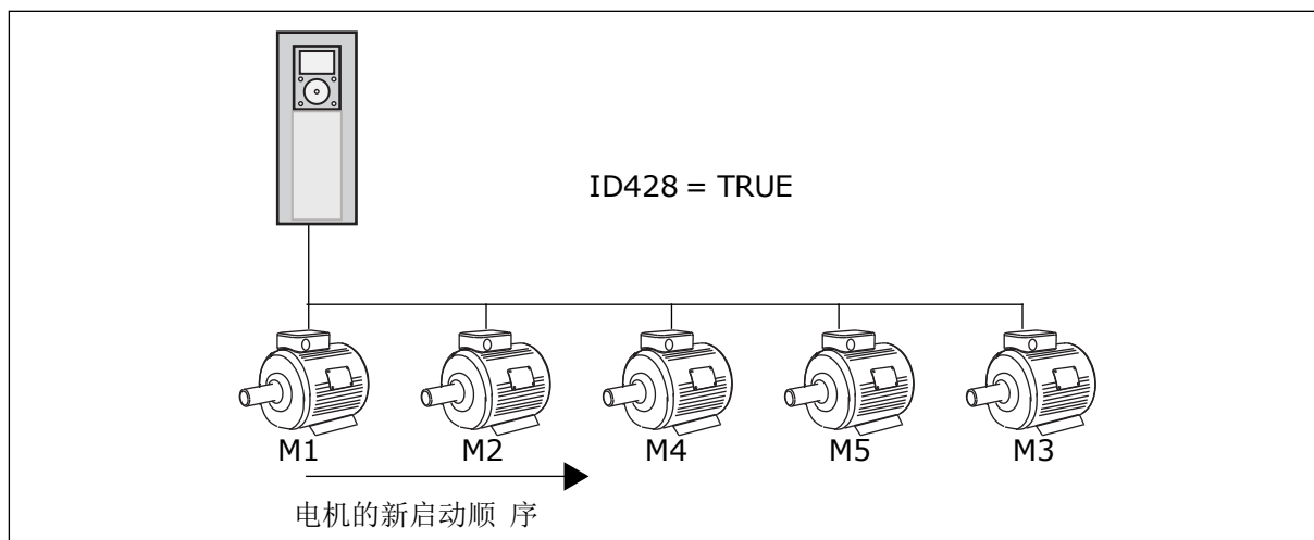
图 47: 互锁逻辑 3
