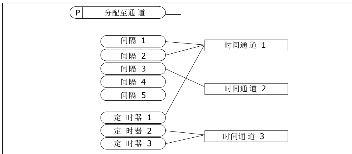
图 34: 将间隔和定时器分配至时间通道很灵活。每个间隔和定时器都有一个参数，可以使用此参数将其分配至某个时间通道。
