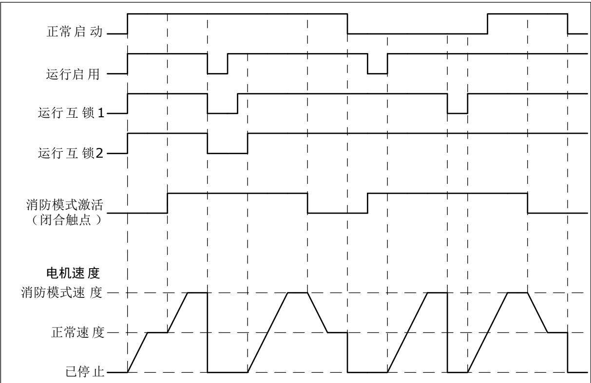
图 51: 消防模式功能
