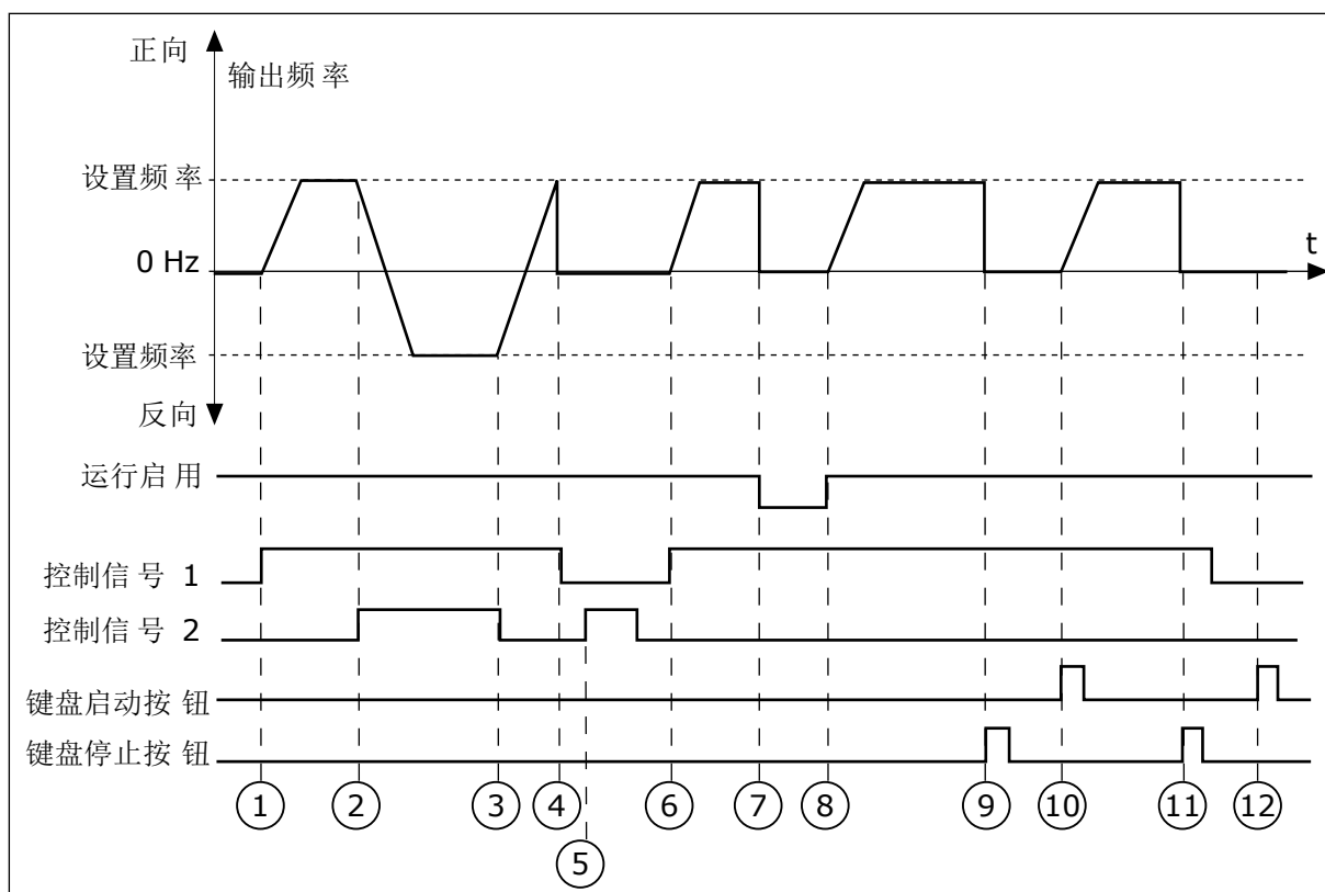
图 18: I/O A 启动/停止逻辑 = 3
