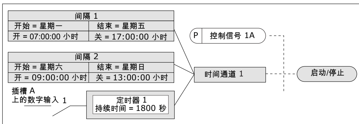
图 36: 时间通道 1 ( 而非数字输入 ) 用作启动命令的控制信号
