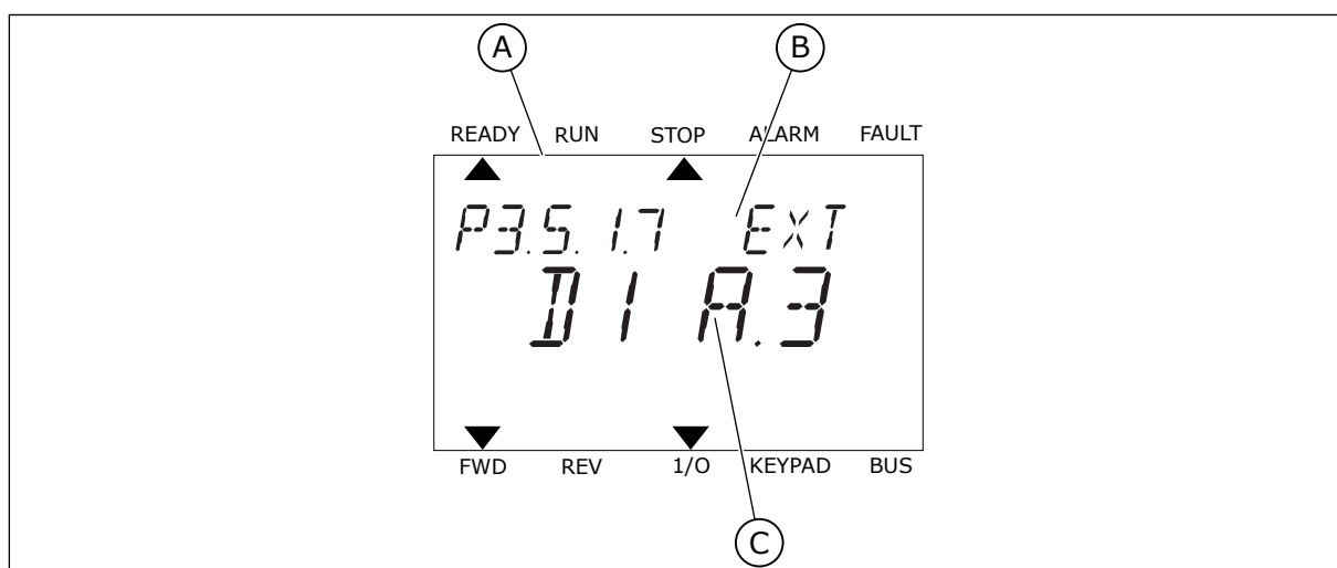
图 24: 文本显示屏中的“数字输入”菜单
