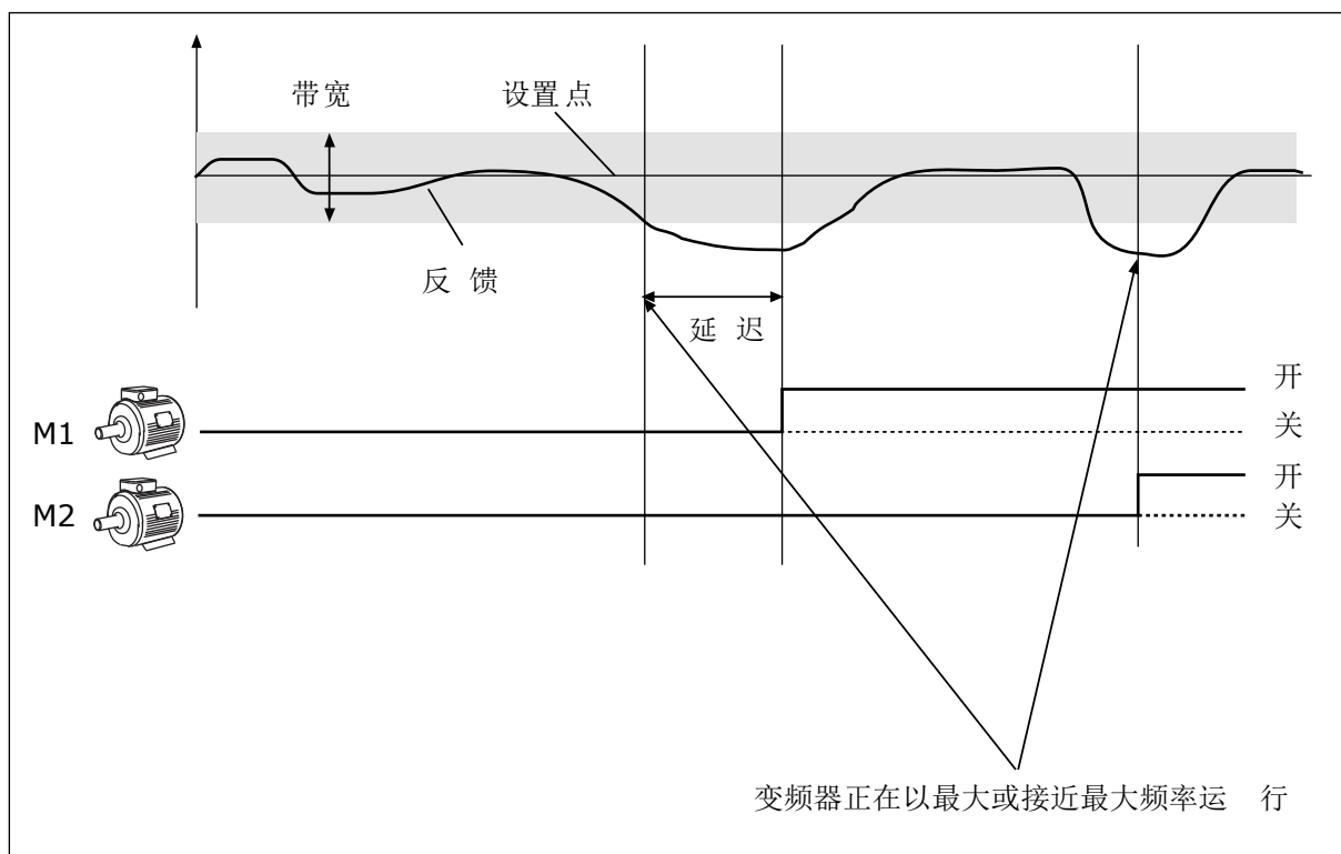
图 44: 多泵功能
