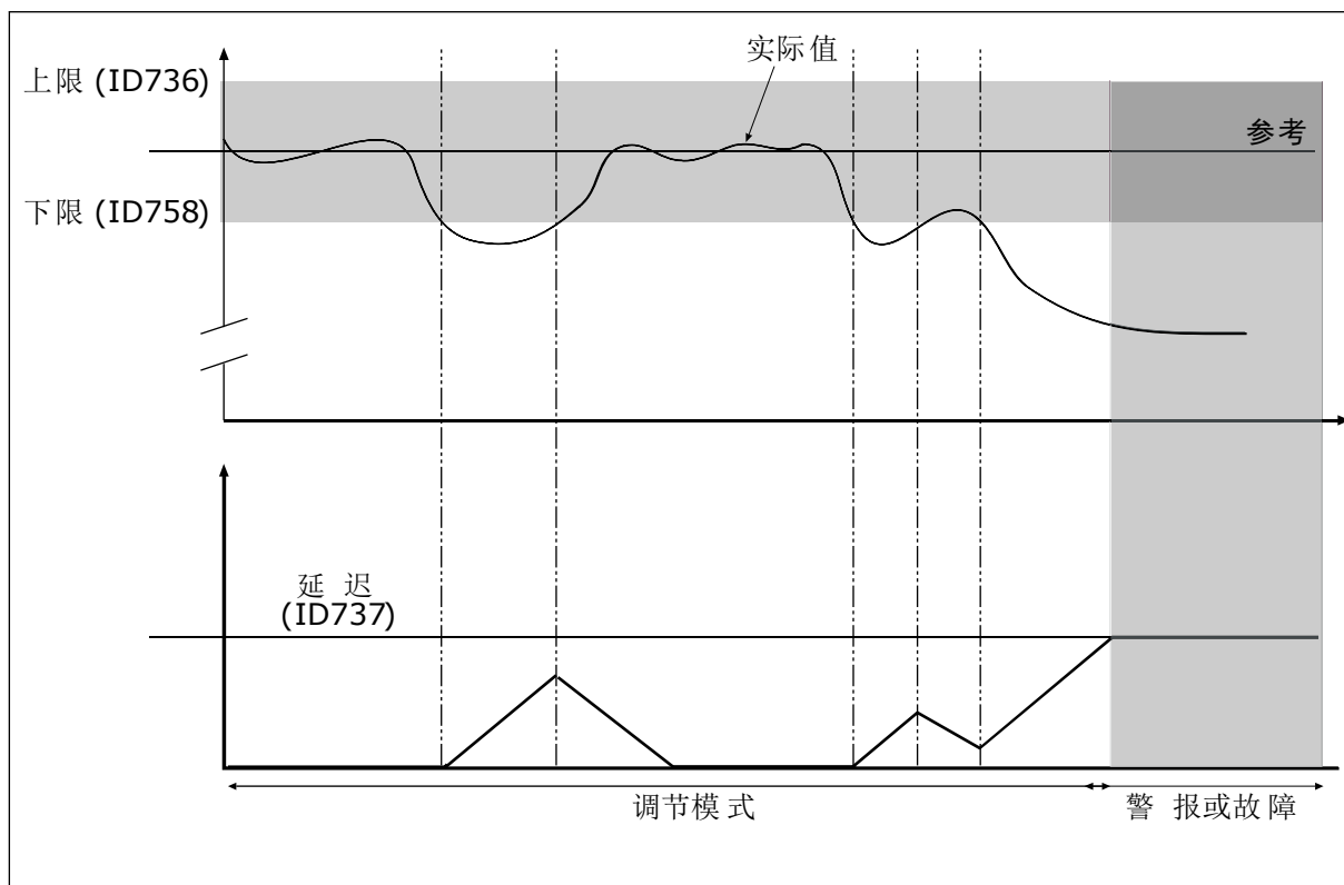
图 41: 反馈监控功能
