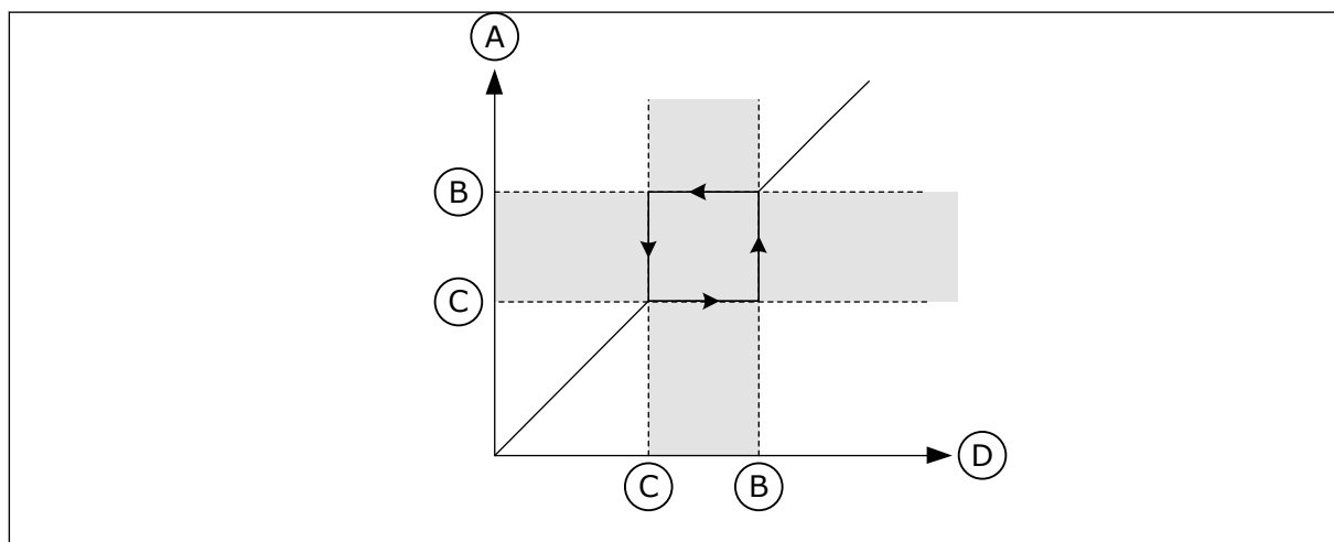
图 26: 禁止的频率
