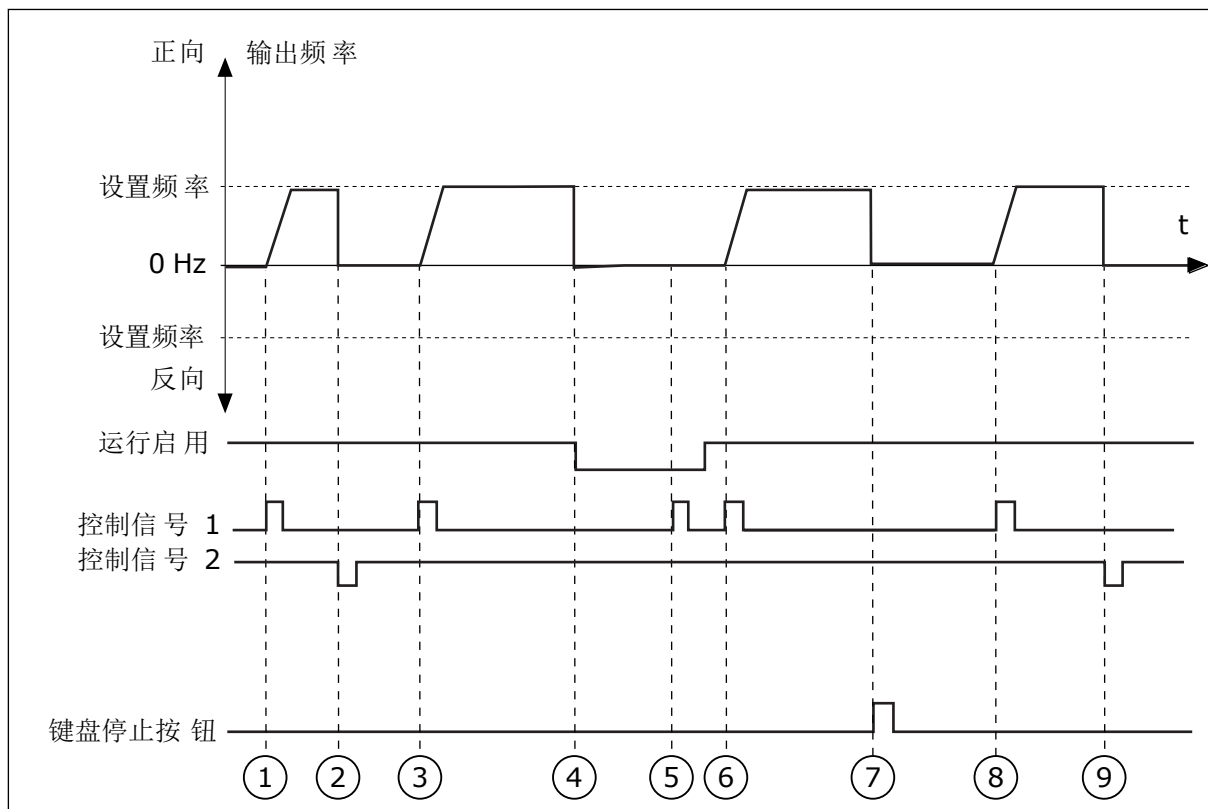
图 16: I/O A 启动/停止逻辑 = 1
