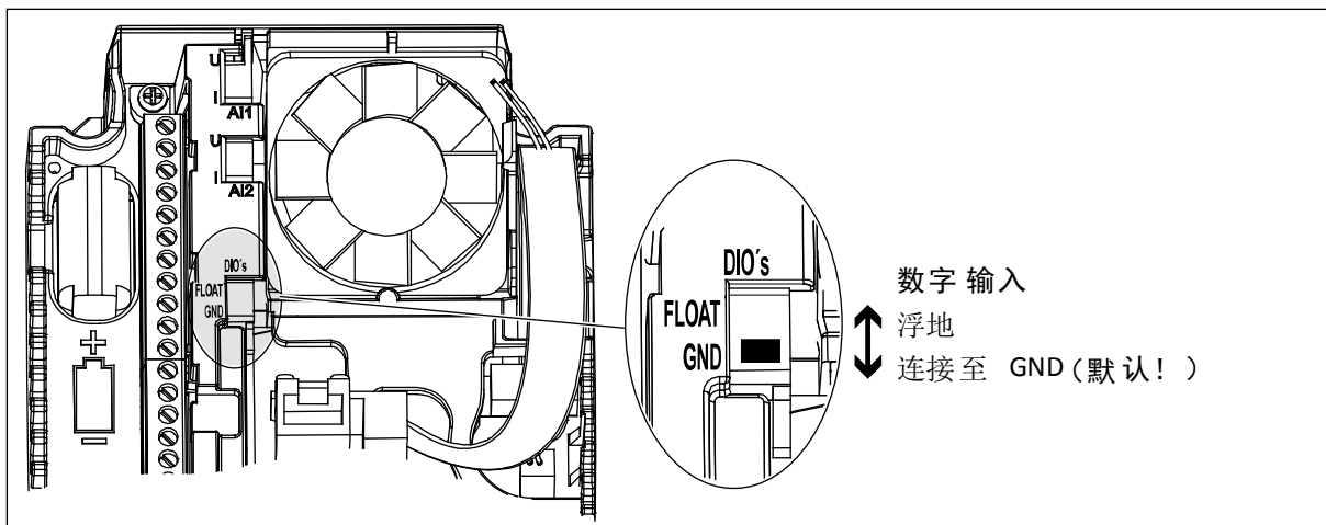
图 7: DIP 开关
