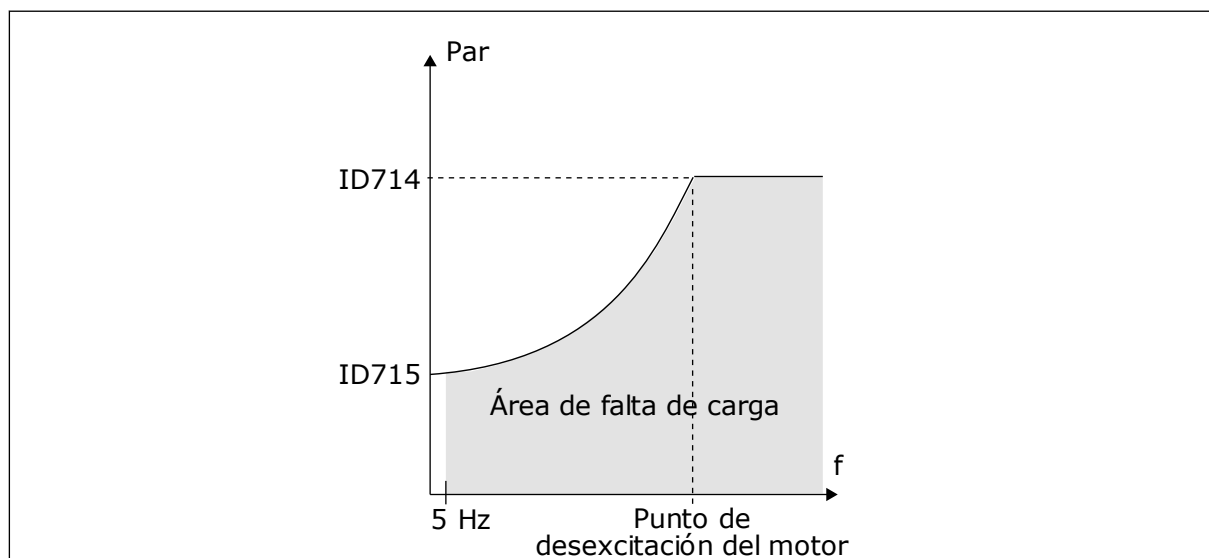
Imag. 69: Ajuste de la carga mínima
