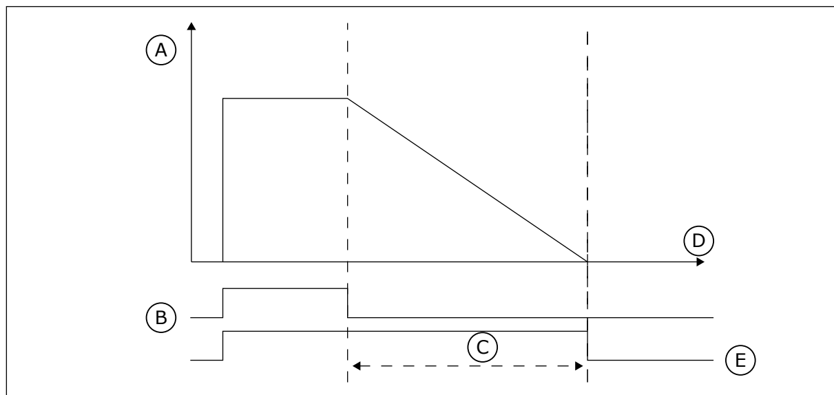
Imag. 74: La señal de activación procede de una entrada digital o una entrada digital virtual, como un canal de tiempo. El temporizador inicia la cuenta atrás desde el flanco descendente.
