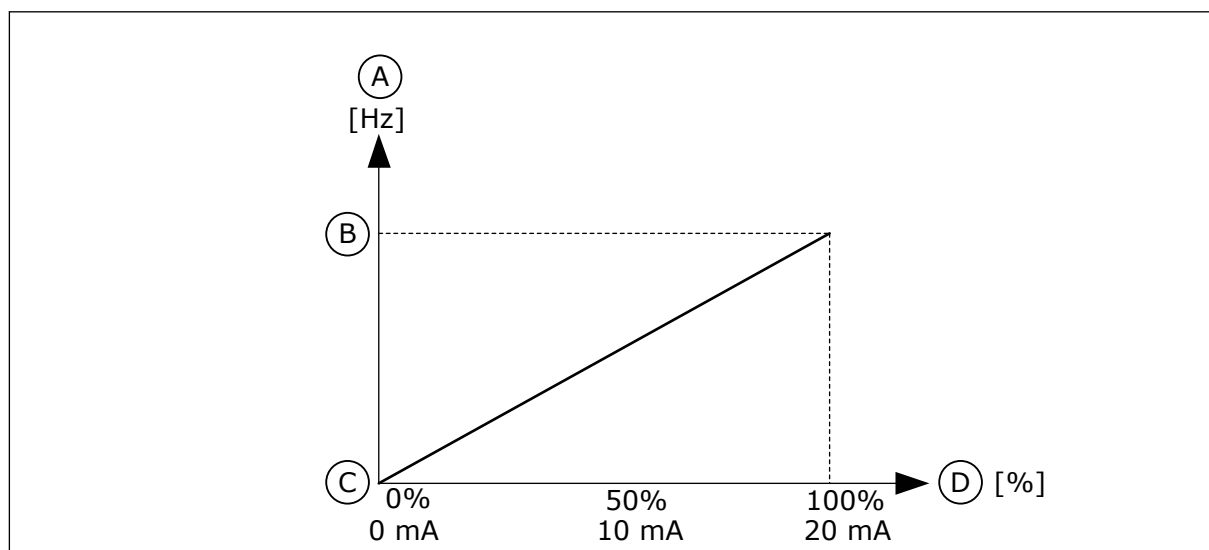
Imag. 60: Inversión de la señal de entrada analógica 1 (AI1), selección 0
