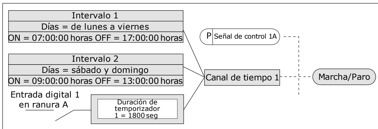
Imag. 78: El canal de tiempo 1 se utiliza como señal de control para la orden de marcha en lugar de una entrada digital
