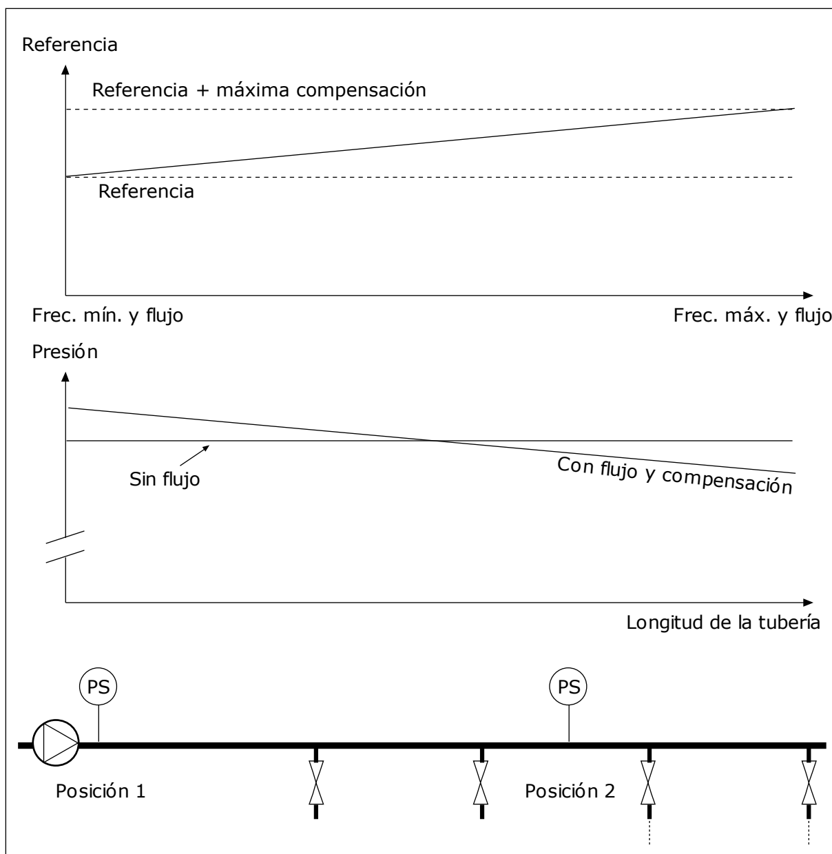
Imag. 85: Habilitar la referencia 1 para la compensación por pérdida de presión.
