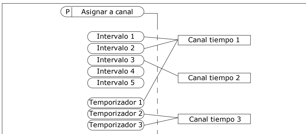
Imag. 73: La asignación de intervalos y temporizadores a los canales de tiempo es flexible. Cada intervalo y cada temporizador tiene un parámetro con el cual puede asignarlos a un canal de tiempo.
