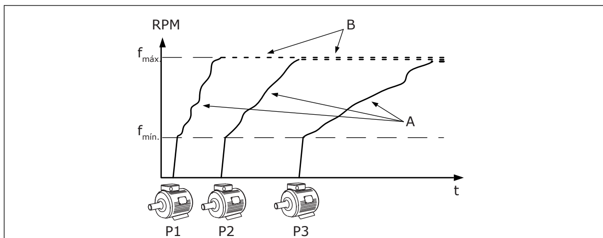
Imag. 15: Control en modo MultiMaster
