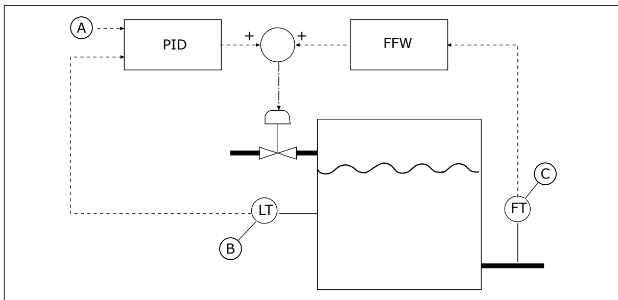
Fig. 80: Edasisöötmise juhtimine
