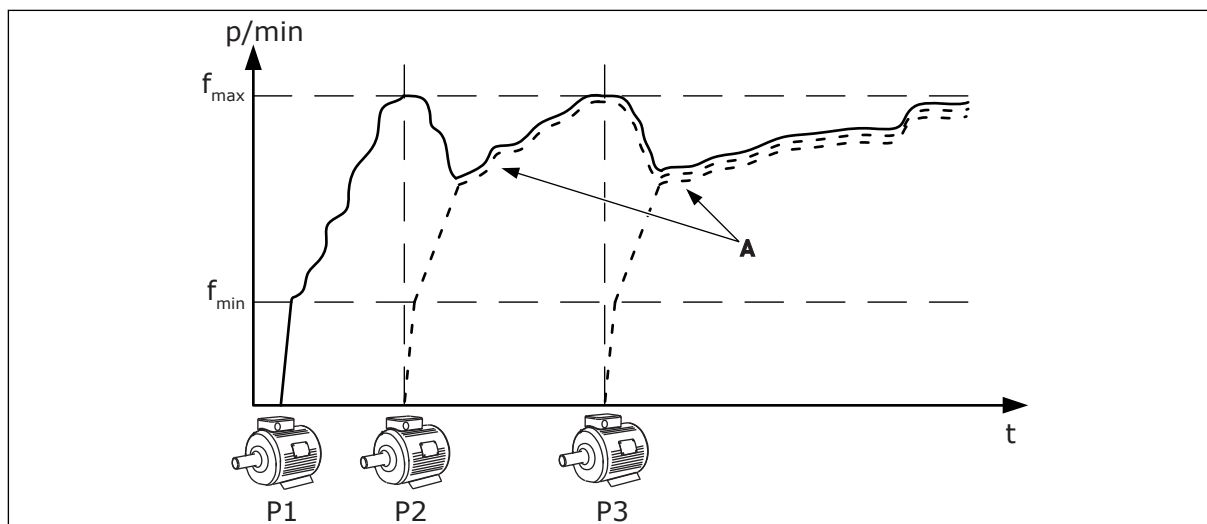
Fig. 14: Juhtimine Multifollower-režiimis
