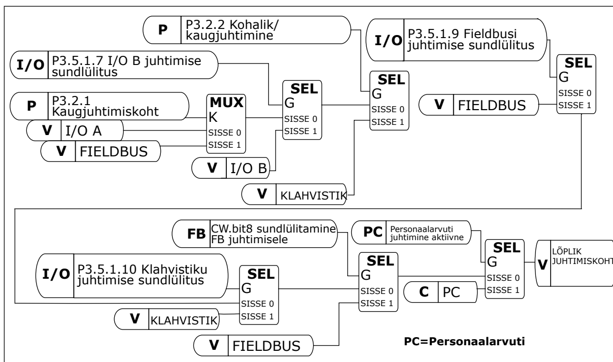
Fig. 41: Juhtimiskoht
