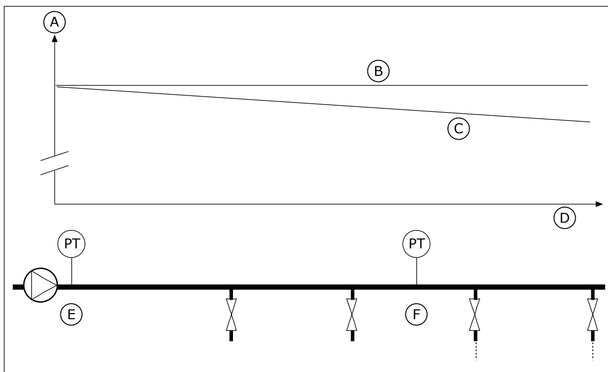
Fig. 84: Rõhuanduri asukoht
