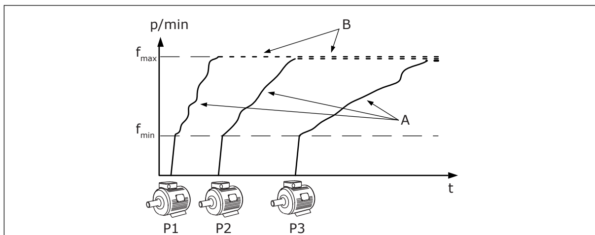
Fig. 15: Juhtimine Multimaster-režiimis
