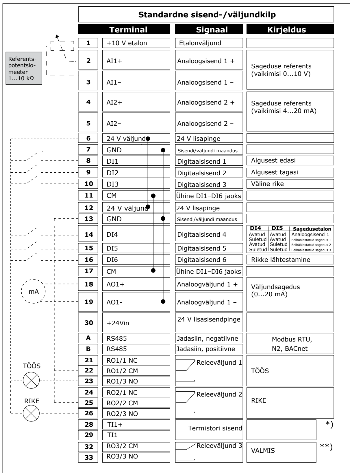
Fig. 4: Standardse ning HVAC rakenduste vaikimisi juhtühendused
