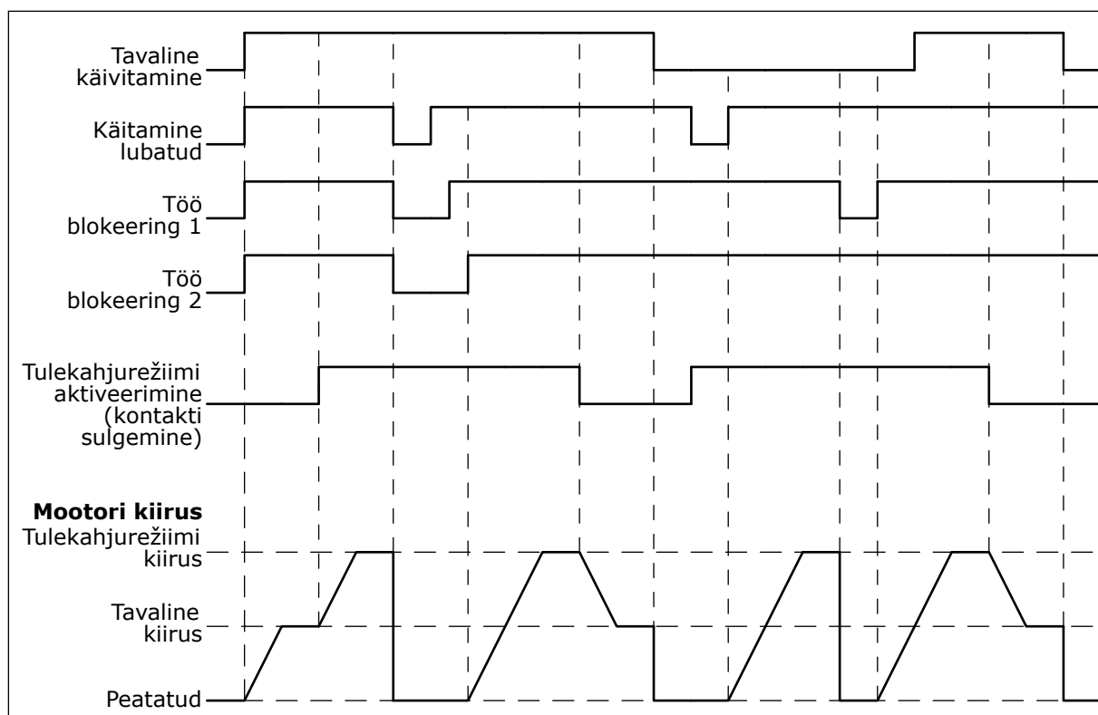
Fig. 103: Tulekahjurežiimi funktsioon
