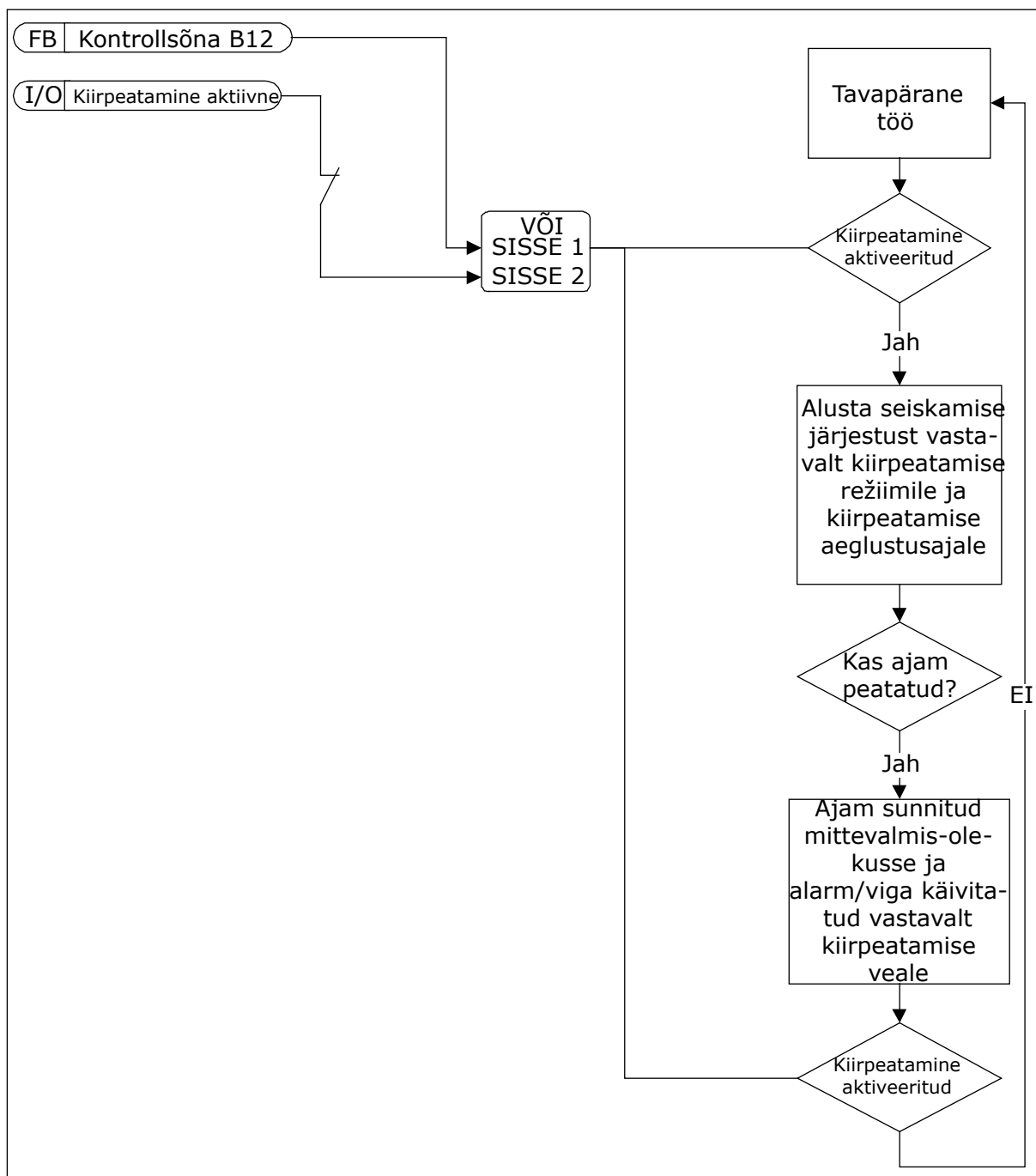
Fig. 71: Kiirpeatamise loogika
