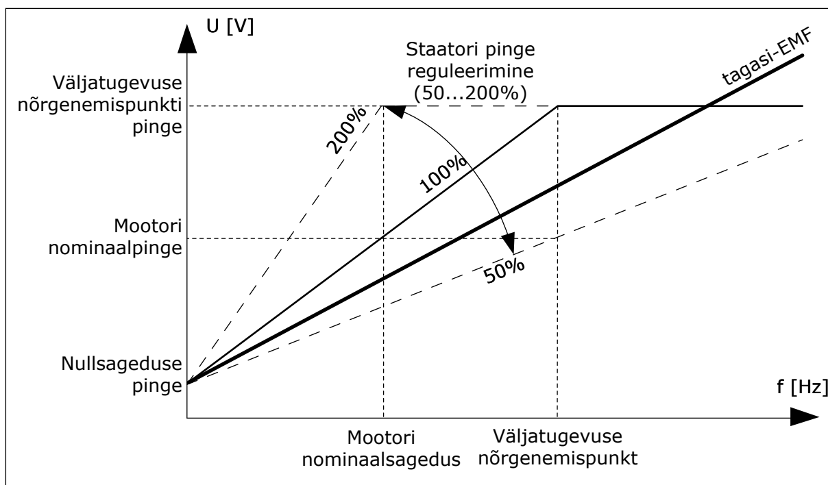
Fig. 37: Staatore pinge reguleerimine
