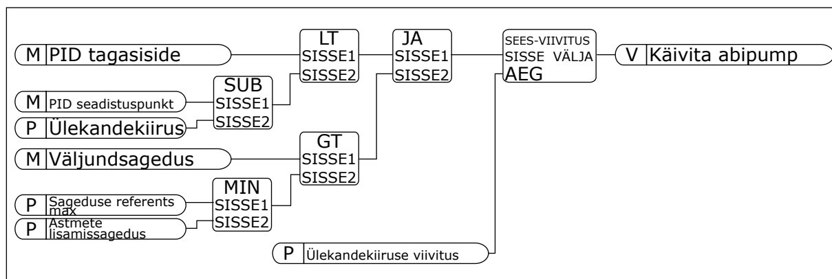
Fig. 101: Astmete lisamissagedus
