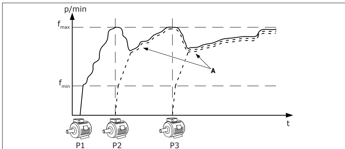
Fig. 92: Juhtimine Multifollower-režiimis
