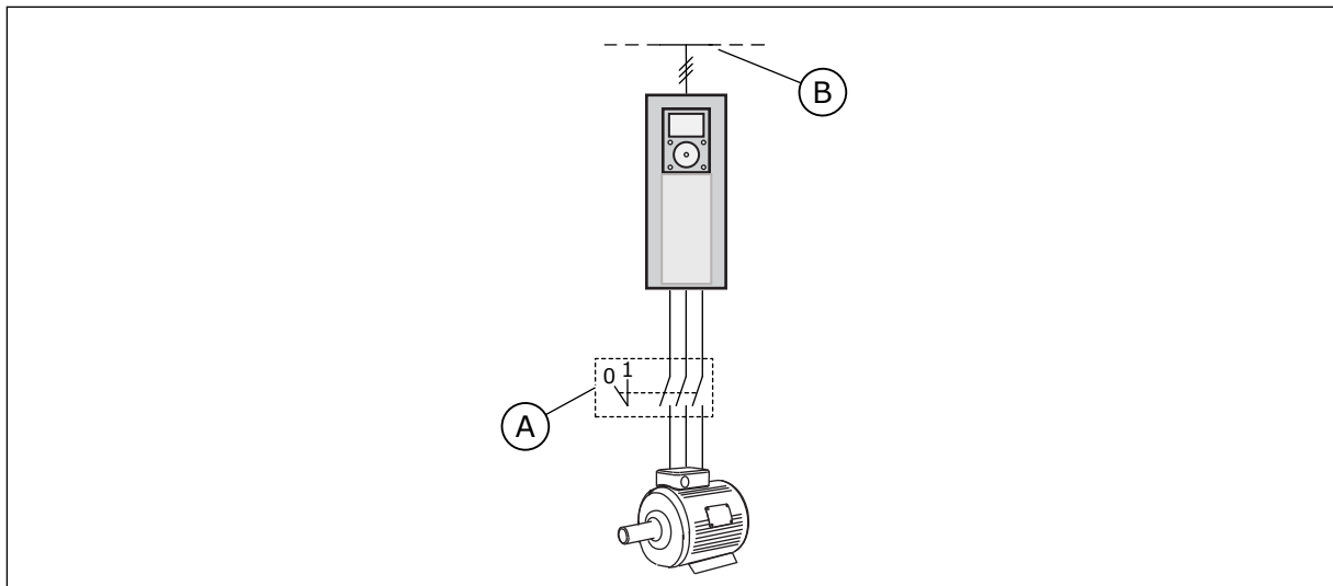
Fig. 36: Mootori lüliti mootori ja ajami vahel
