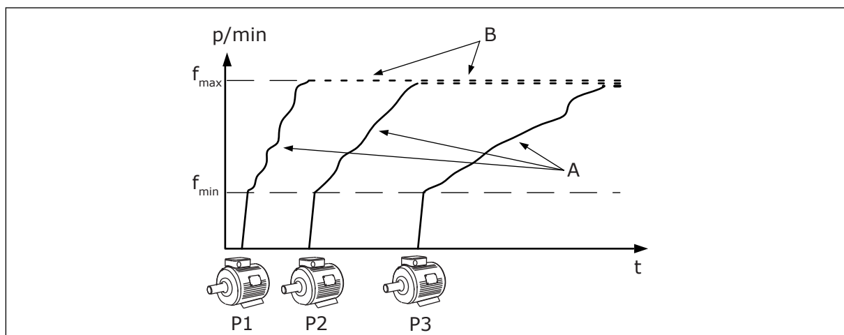
Fig. 93: Juhtimine Multimaster-režiimis
