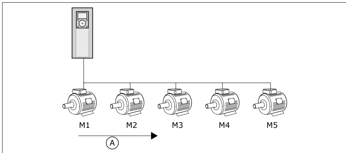
Abb. 81: Interlock-Logik 1
