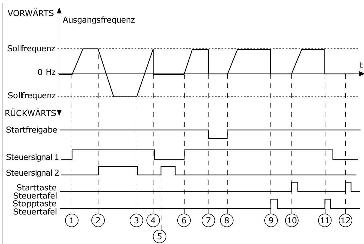
Abb. 31: E/A A Start/Stopp-Auswahl = 3
