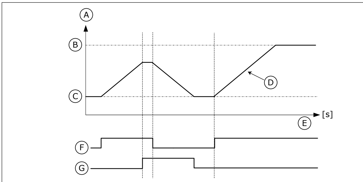
Abb. 37: Motorpotentiometer-Parameter
