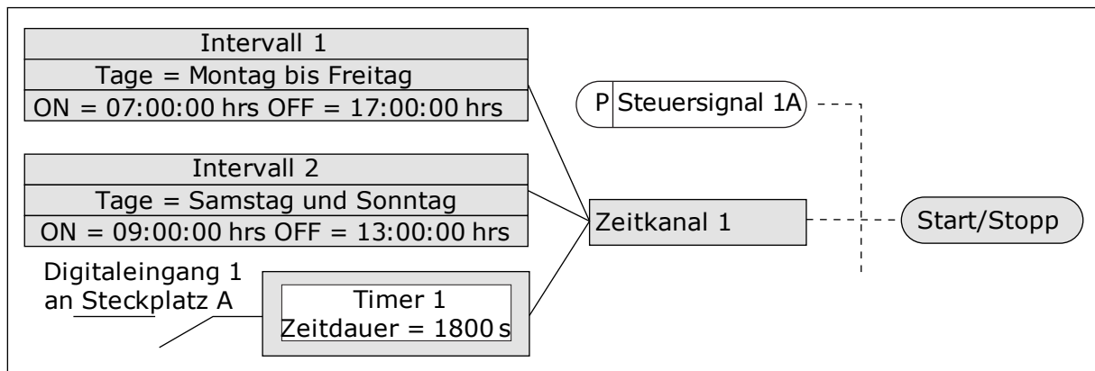
Abb. 69: Zeitkanal 1 wird anstelle eines Digitaleingangs als Steuersignal für den Startbefehl verwendet.
