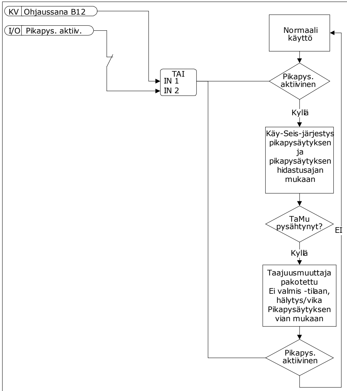
Kuva 71: Pikapysäytyslogiikka.
