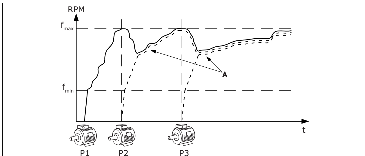
Kuva 92: Ohjaus rinnansäätötilassa.
