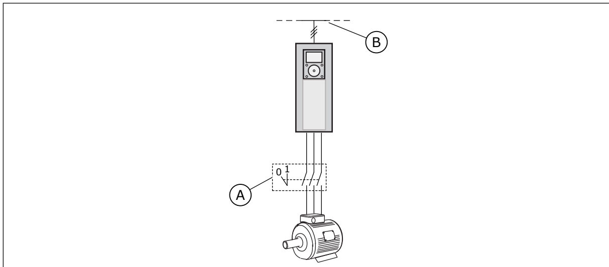
Kuva 36: Taajuusmuuttajan ja moottorin välissä oleva moottorikytkin
