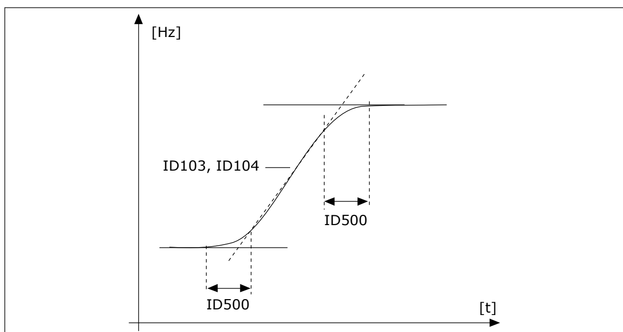
Kuva 48: Kiihdytys-/hidastuskäyrä (S-muoto)
