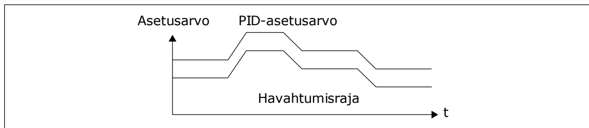
Kuva 82: Havahtumistila: suhteellinen asetusrvo.
