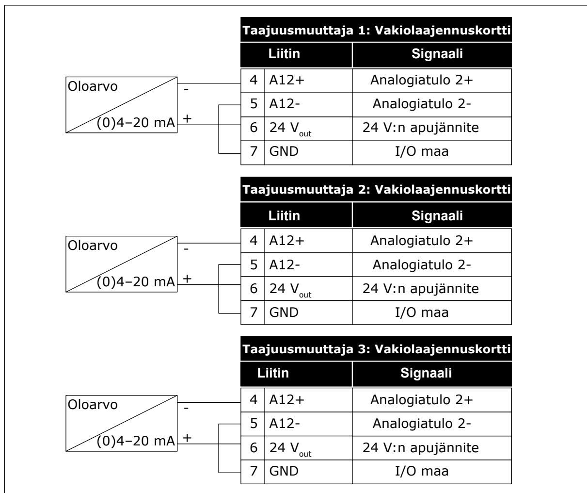
Kuva 94: Takaisinkytkentäanturien kytkentä taajuusmuuttajiin
