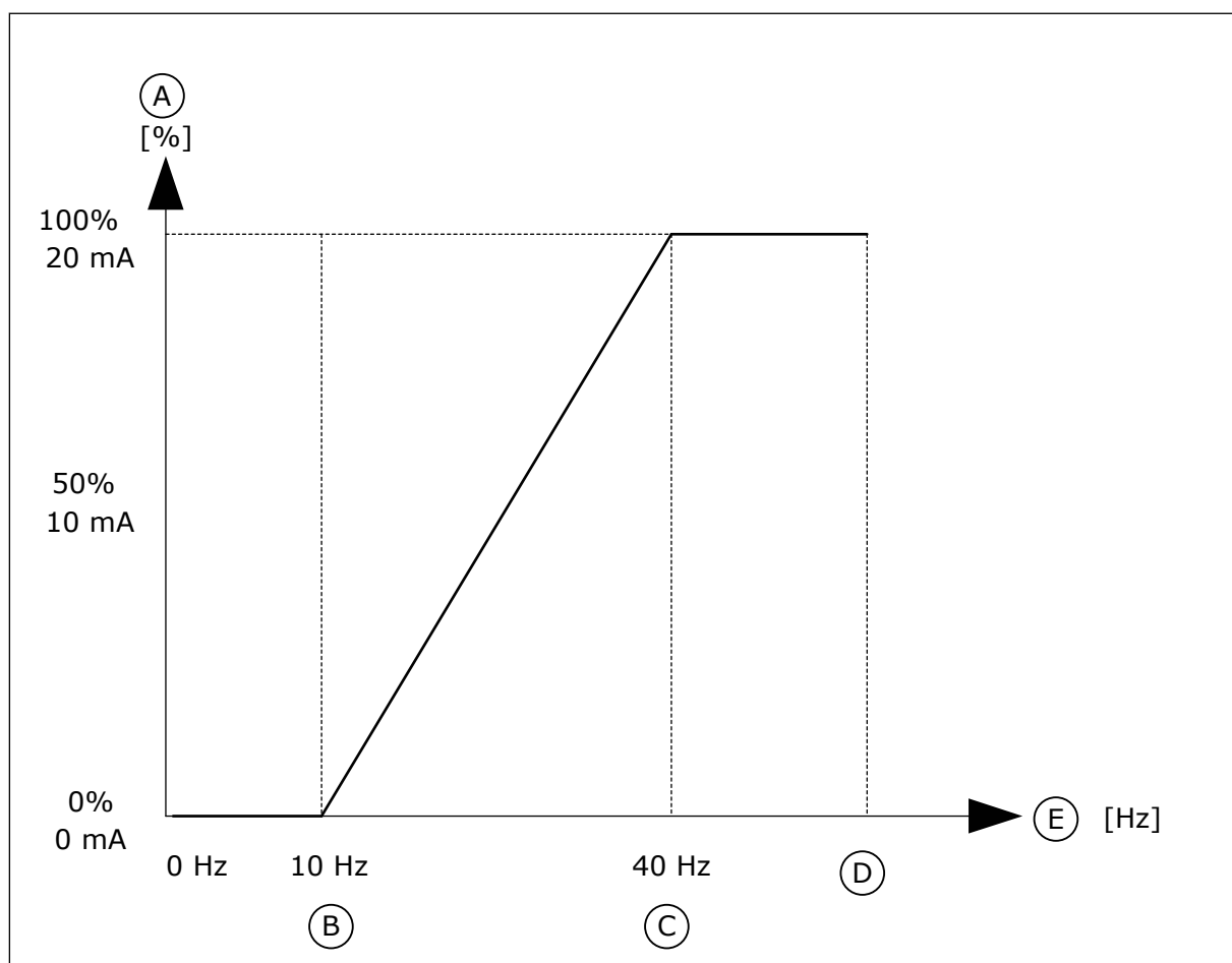
Kuva 62: A01-signaalin skaalaus
