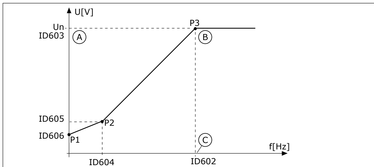
Kuva 39: Ohjelmoitava U/f-käyrä
