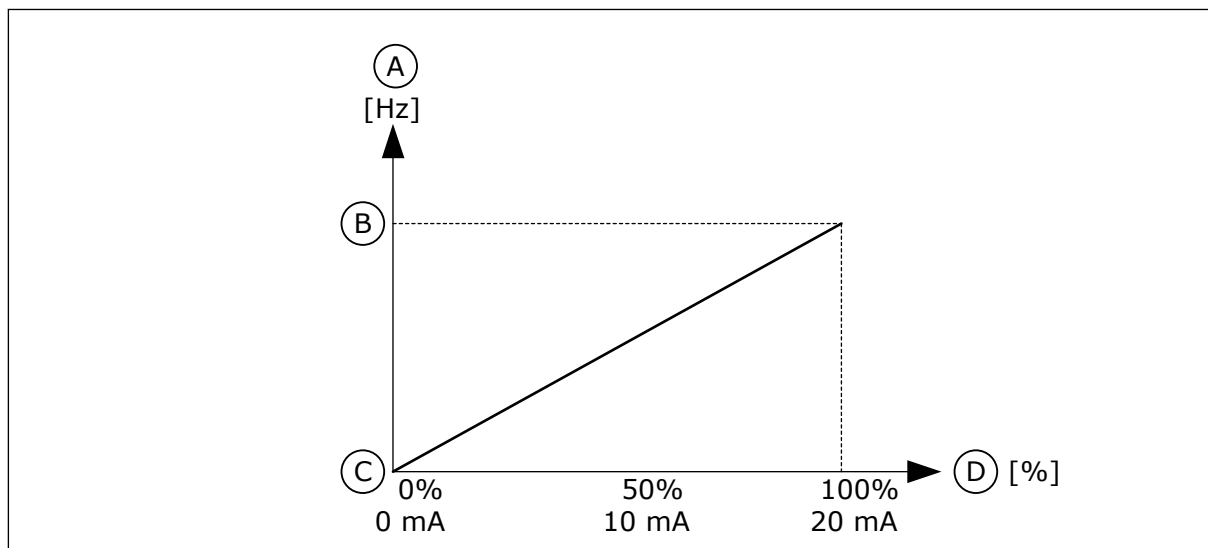
Kuva 57: Analogiatulon signaaliarvo, valinta 0
