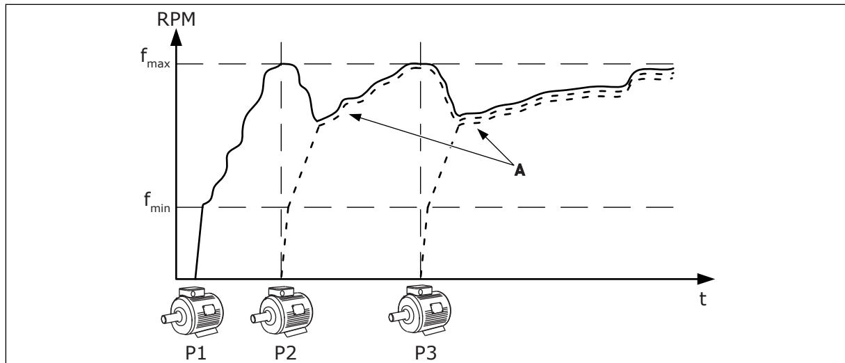
Kuva 14: Ohjaus rinnansäätötilassa.
