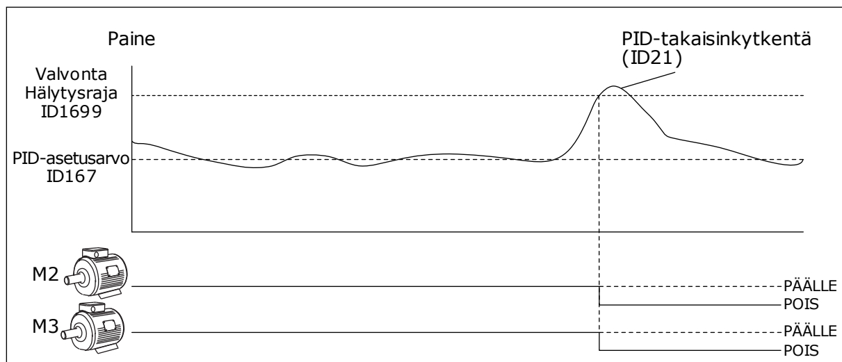
Kuva 100: Ylipaineen valvontatoiminto
