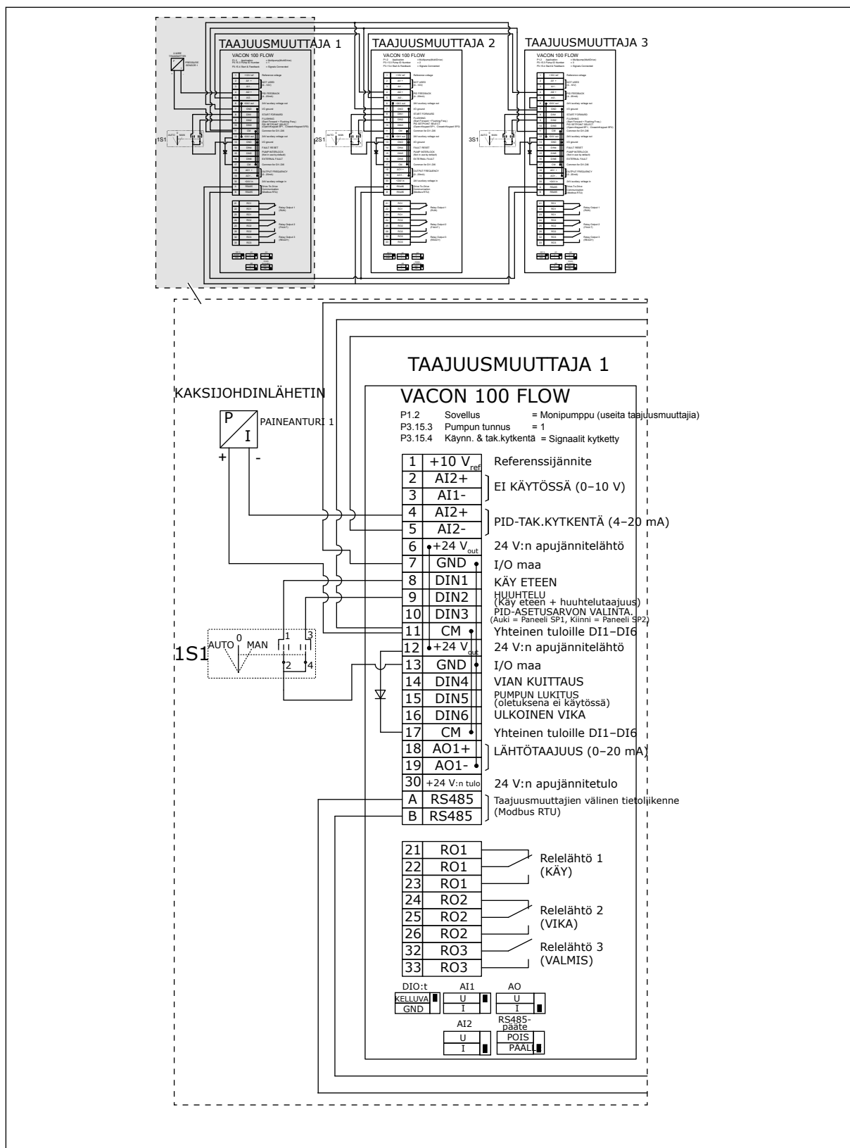
Kuva 21: Usean taajuusmuuttajan monipumppujärjestelmän kytkentäkaavio, esimerkki 2A
