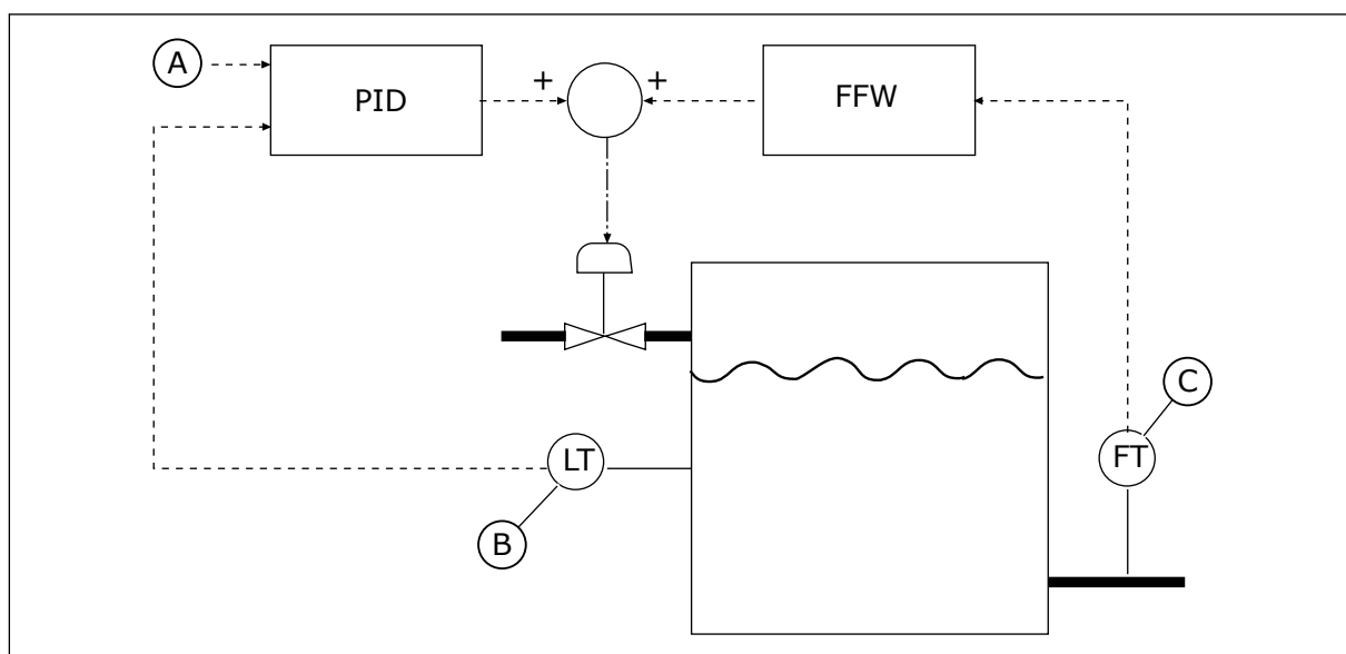
Kuva 80: Myötäkytkentäohjaus.
