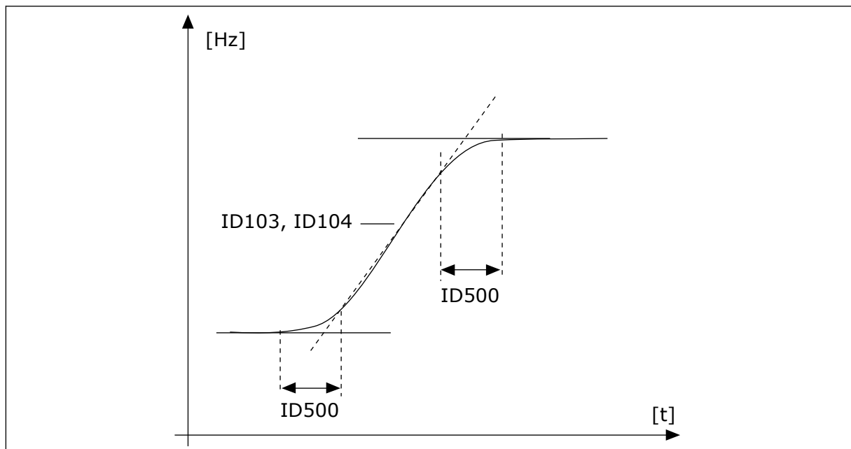
Kuva 49: Kiihdytys-/hidastuskäyrä (S-muoto)
