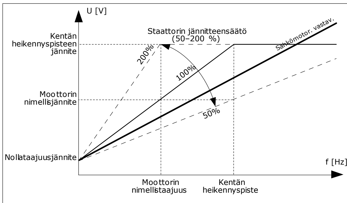
Kuva 37: Staatton jännitteensäätö
