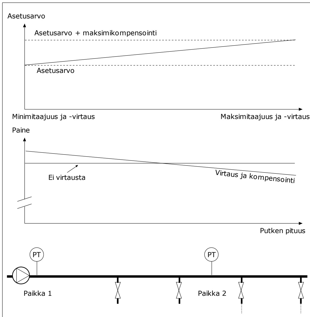
Kuva 85: Painehäviön kompensoinnin asetusarvo 1 on käytössä.
