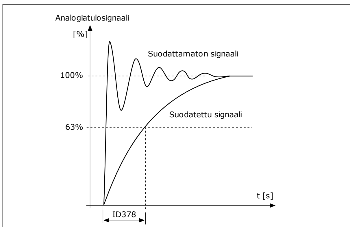
Kuva 56: AI1-signaalin suodatus.
