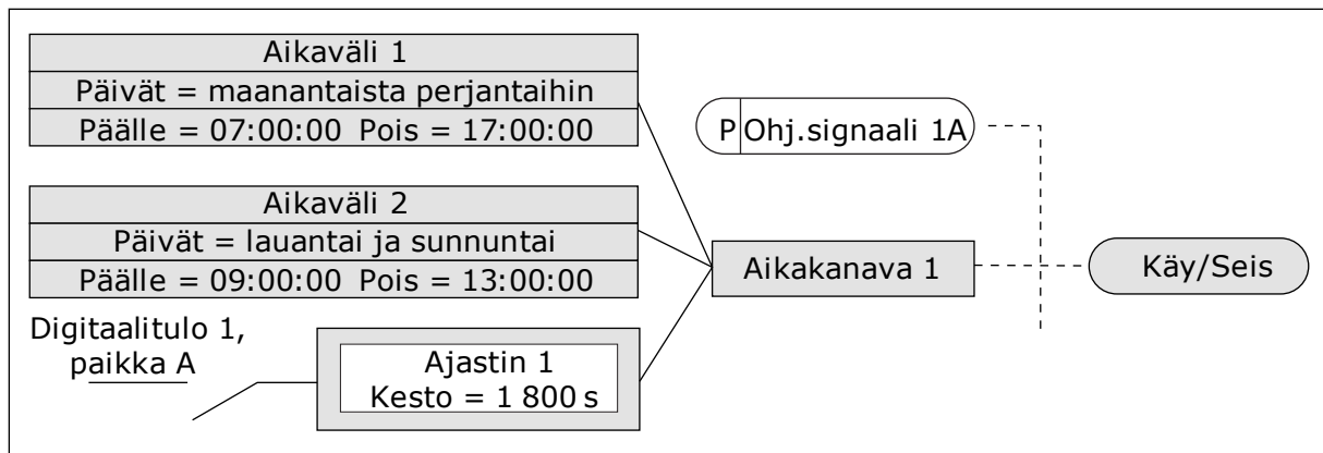
Kuva 78: Käynnistyskomennon ohjaussignaalina käytetään aikakanavaa 1 digitaalitulon sijasta.
