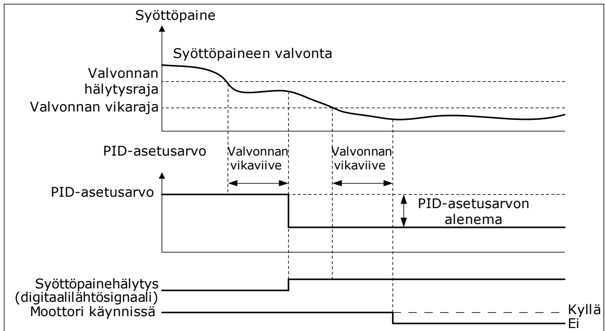
Kuva 87: Syöttöpaineen valvontatoiminto
