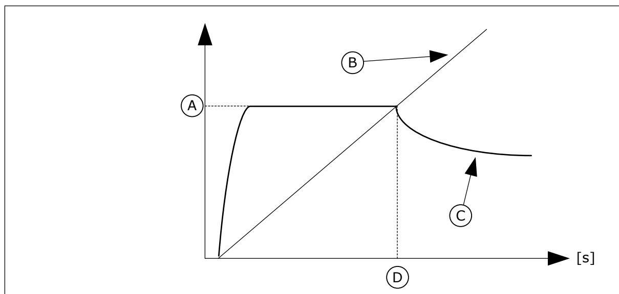
Kuva 40: I/f-käynnistyksen parametrit
