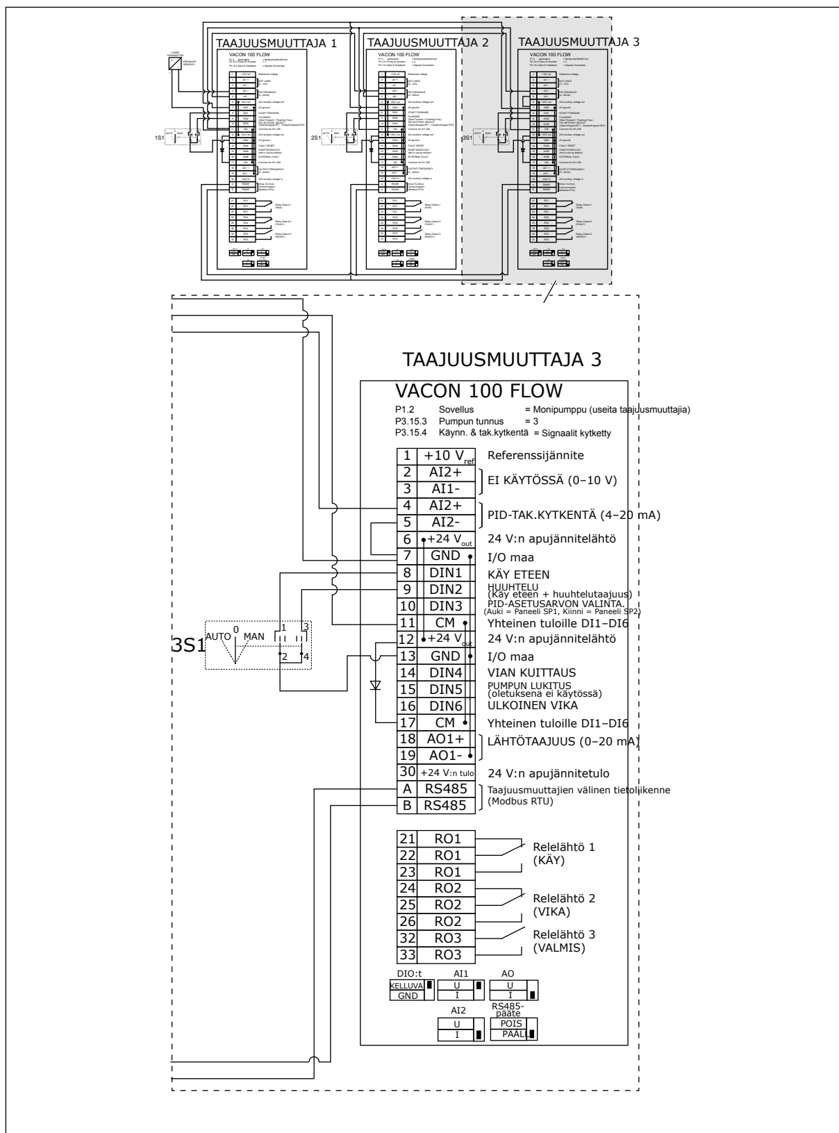
Kuva 23: Usean taajuusmuuttajan monipumppujärjestelmän kytkentäkaavio, esimerkki 2C
