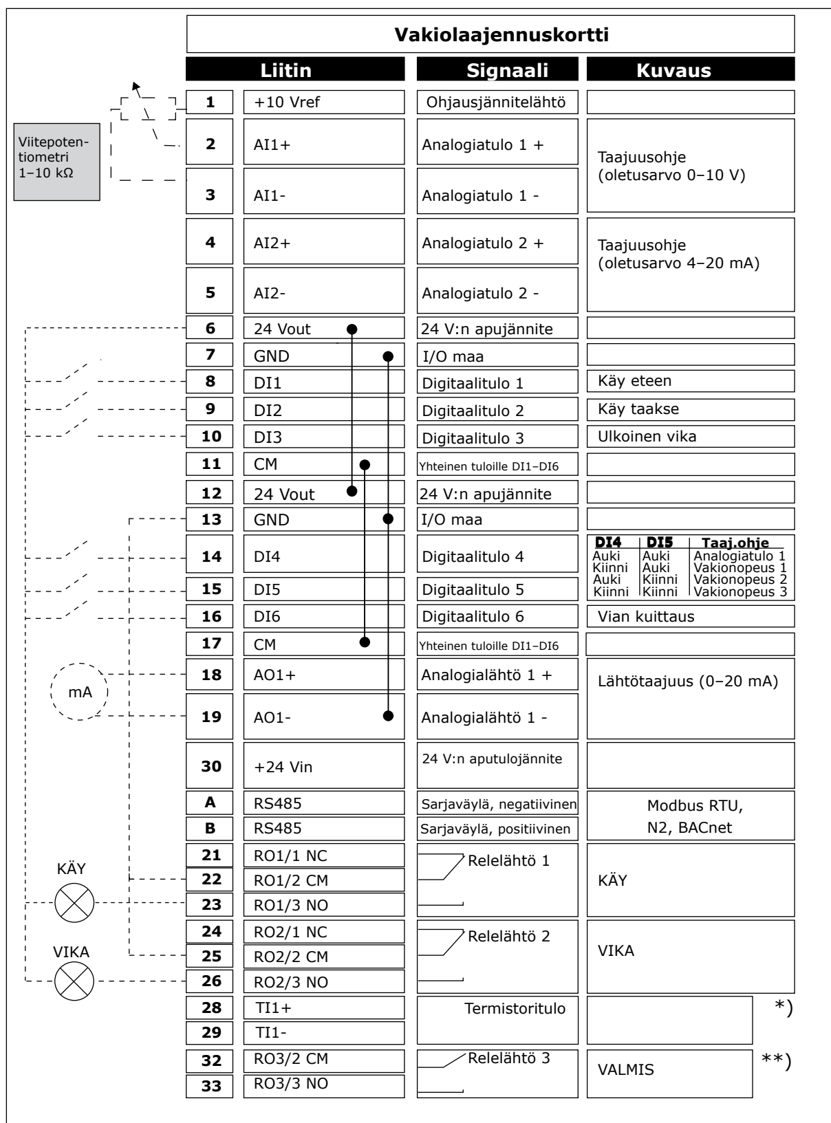
Kuva 4: Vakio- ja HVAC-sovellusten oletusohjausliitännät
