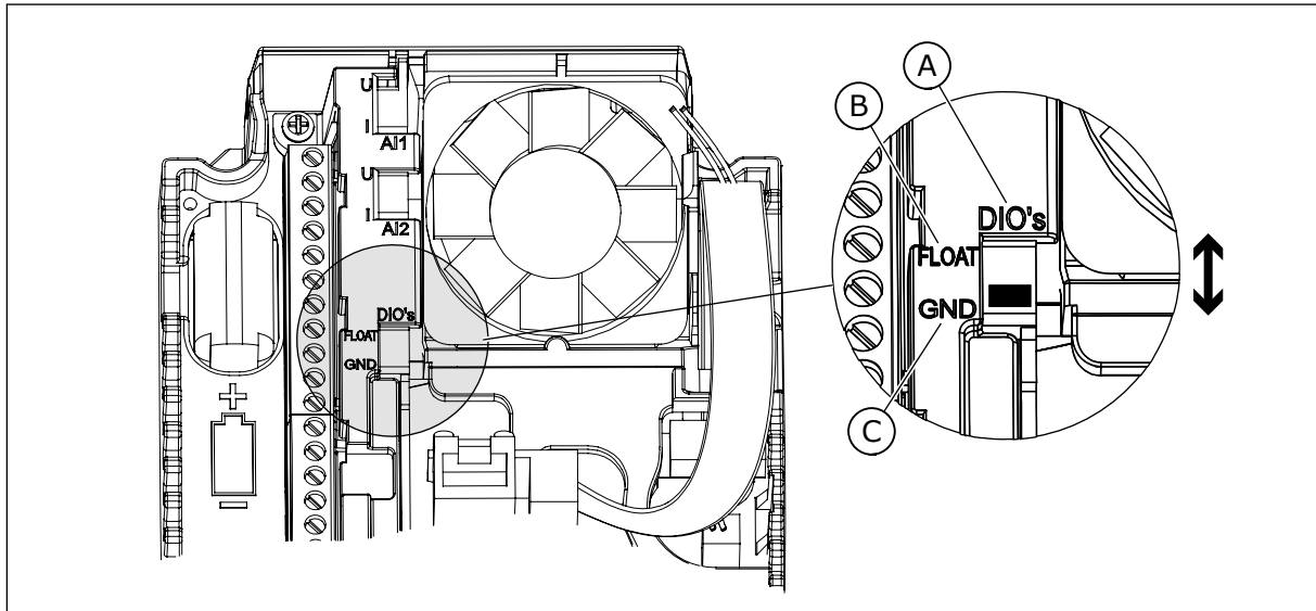
Kuva 12: DIP-kytkin
