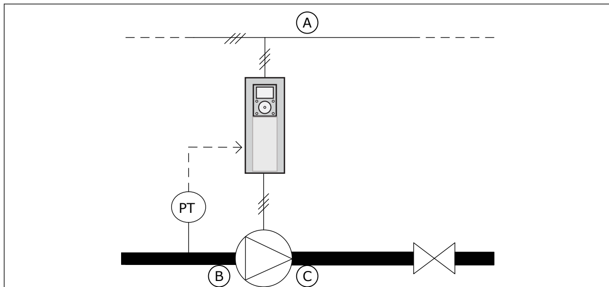
Kuva 86: Paineanturin paikka
