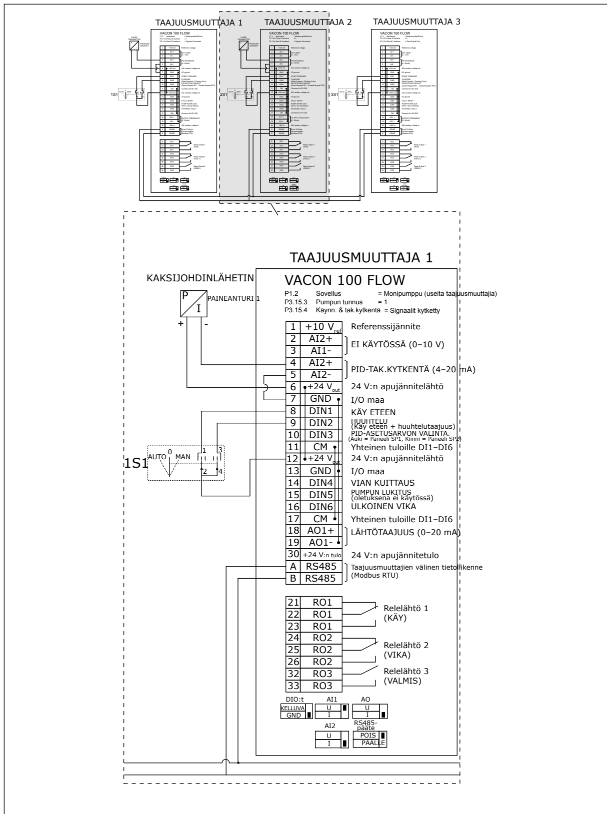
Kuva 25: Usean taaajuusmuuttajan monipumppujärjestelmän kytkentäkaavio, esimerkki 3B
