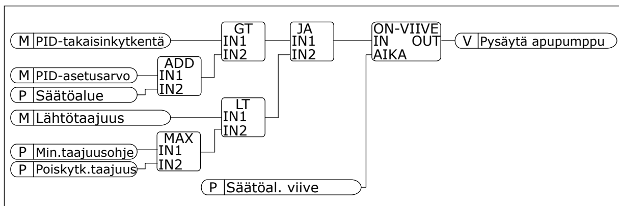
Kuva 102: Poiskytkentätaajuus
