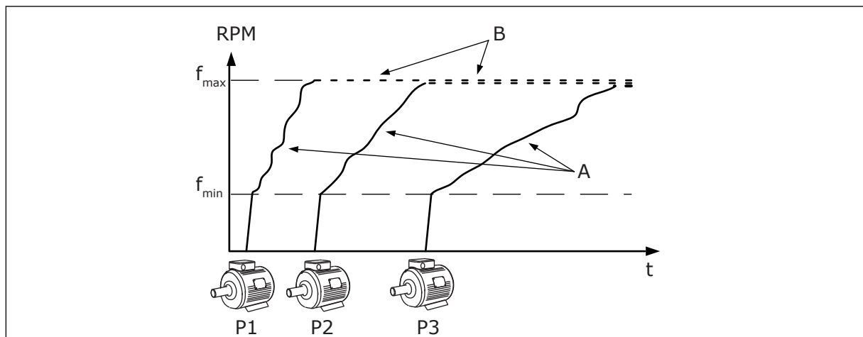
Kuva 15: Ohjaus monisäätötilassa.
