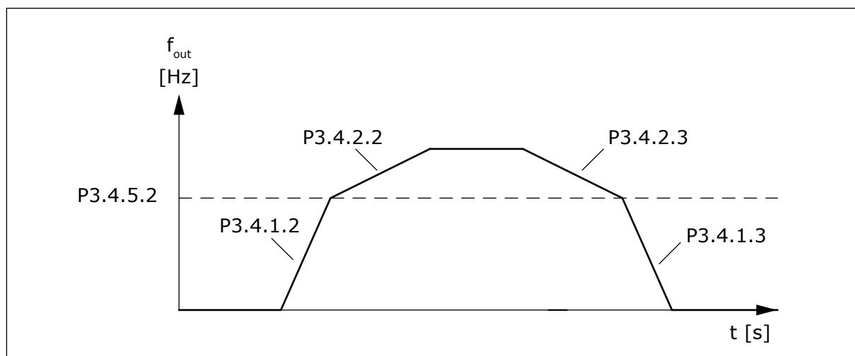
Kuva 50: Rampin 2 aktivointi, kun lähtötaajuus ylittää kynnysarvon. (P3.4.5.2 = Kiihdyt. 2 taajuusraja, P3.4.1.2 = Kiiht.aika 1, P3.4.2.2 = Kiiht.aika 2, P3.4.1.3 = Hid.aika 1, P3.4.2.3 = Hid.aika 2).
