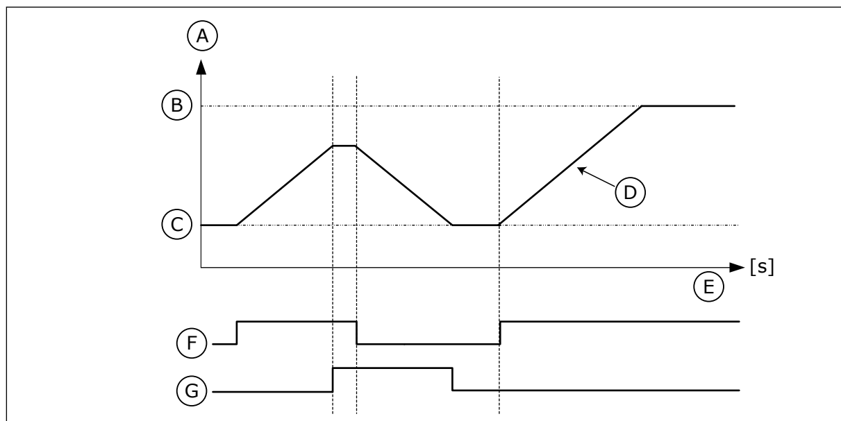
Kuva 47: Moottoripotentiometrin parametrit
