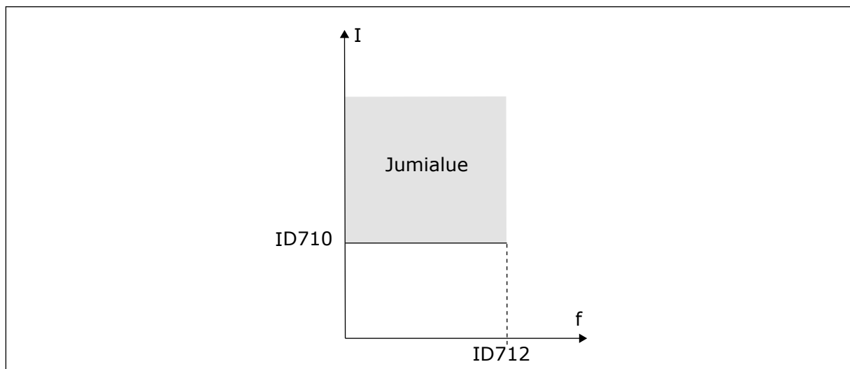
Kuva 68: Jumisuojan asetukset
