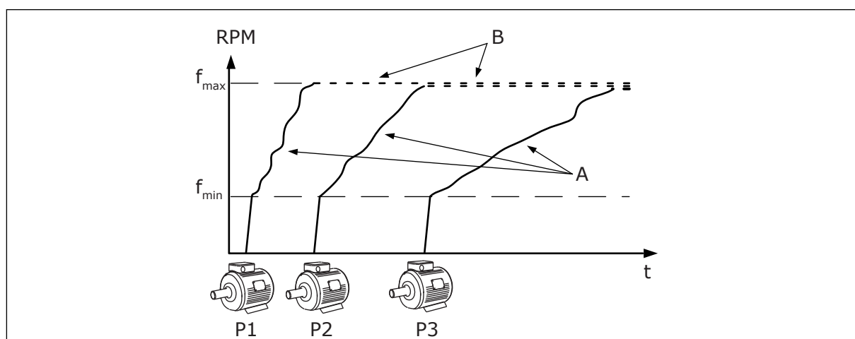
Kuva 93: Ohjaus monisäätötilassa.
