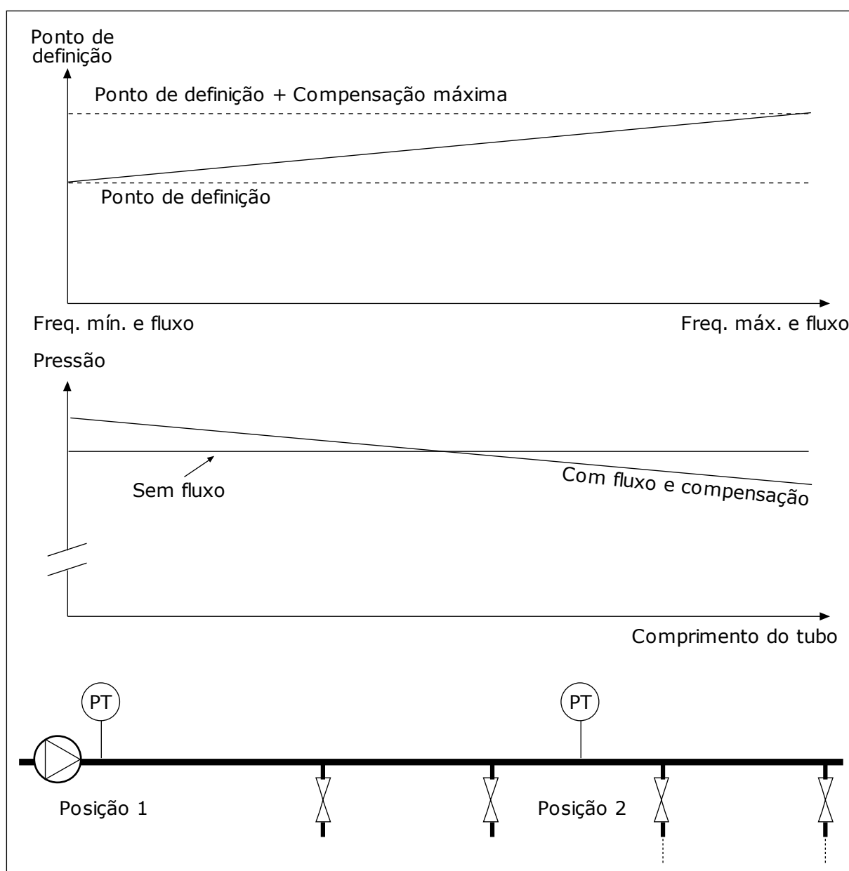
Fig. 76: Ativar ponto de definição 1 para compensação de perda de pressão
