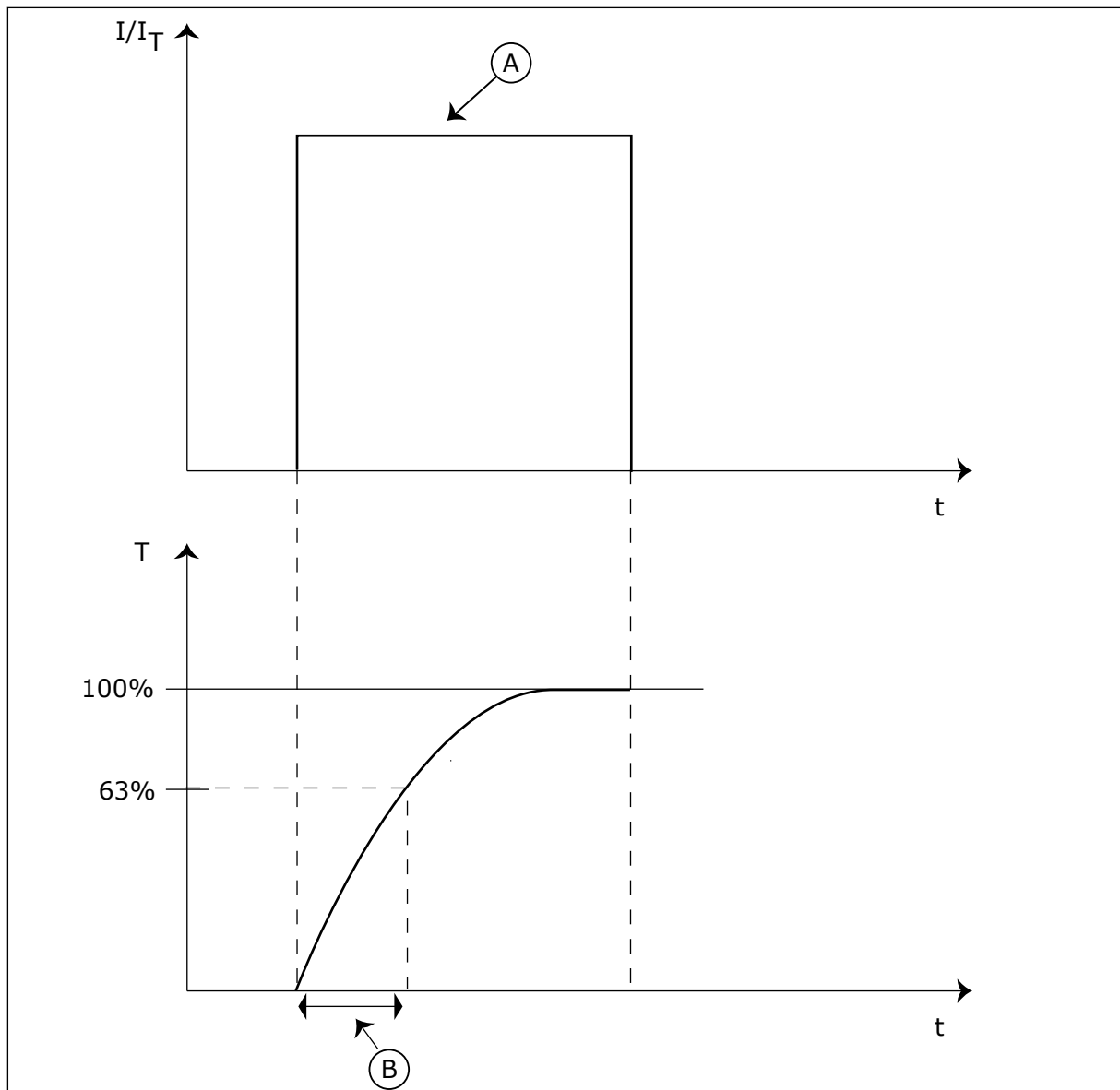
Bild 57: Motorns termiska tidskonstant
