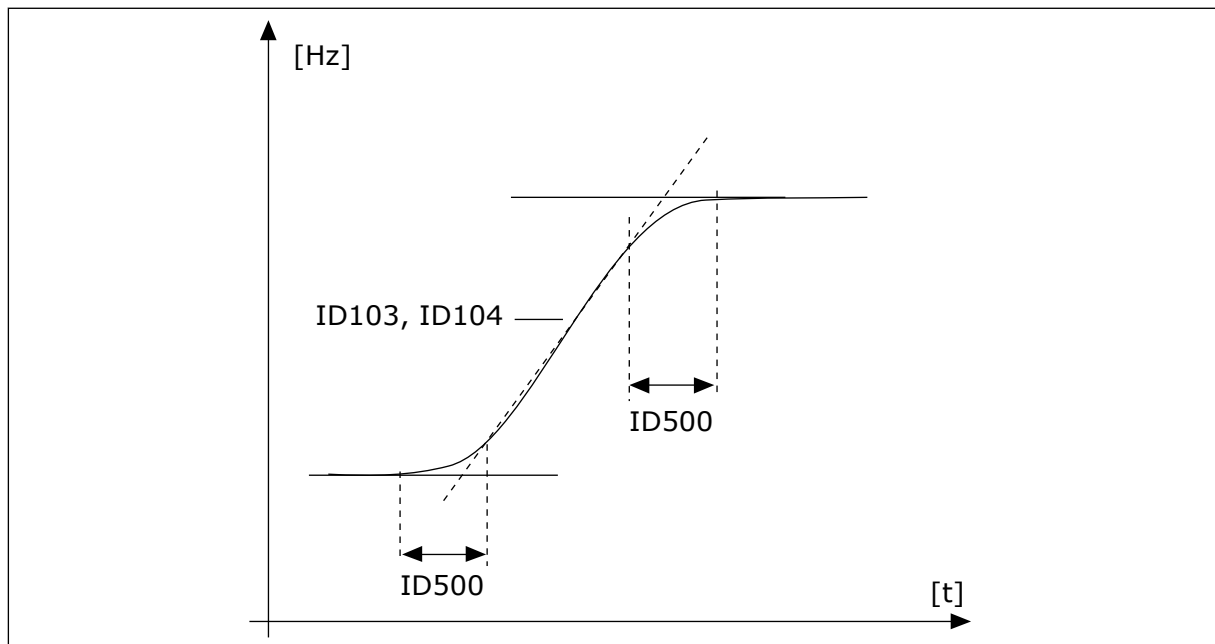
Bild 41: Acceleration/retardation (S-formad)
