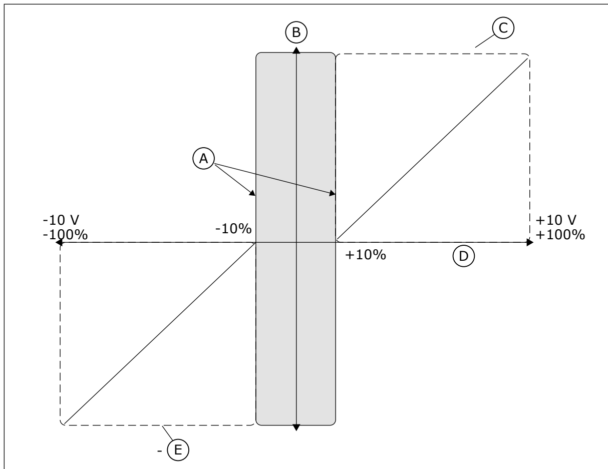
Bild 38: Joystickfunktionen
