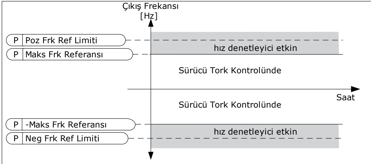
Şekil 35: Tork kontrolü frekans limiti, seçim 0
