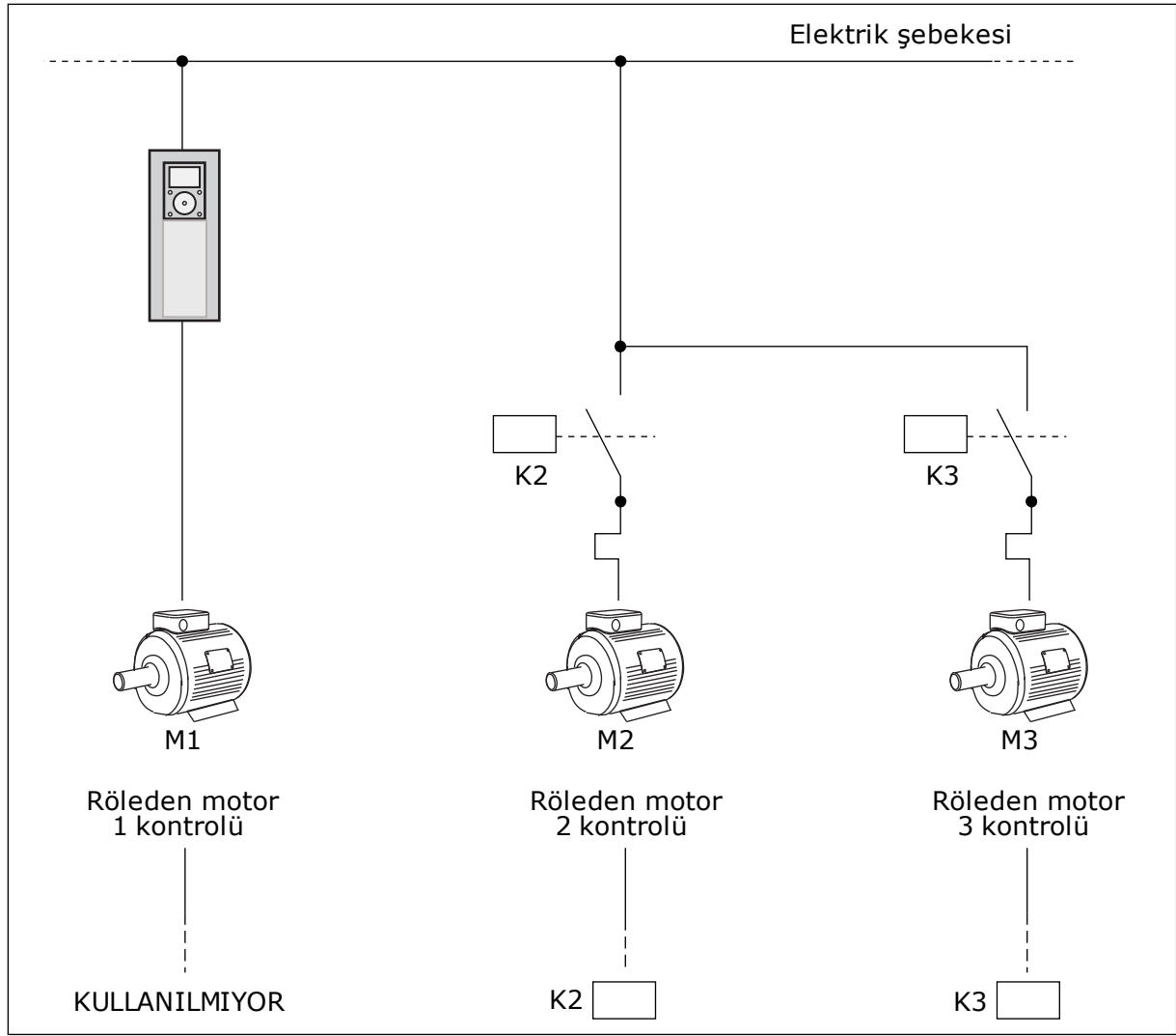
Şekil 84: Seçim 0
