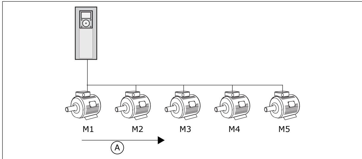
Şekil 81: Bağlantı mantığı 1
