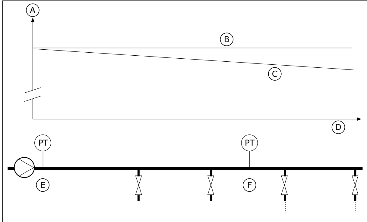
Şekil 75: Basınç sensörünün konumu
