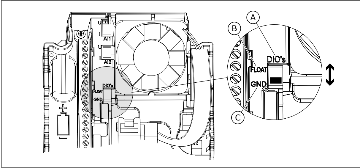
Şekil 11: DIP anahtarı
