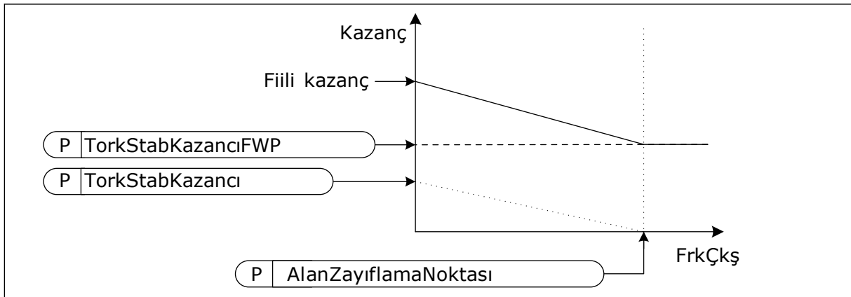
Şekil 26: Tork stabilizör kazancı
