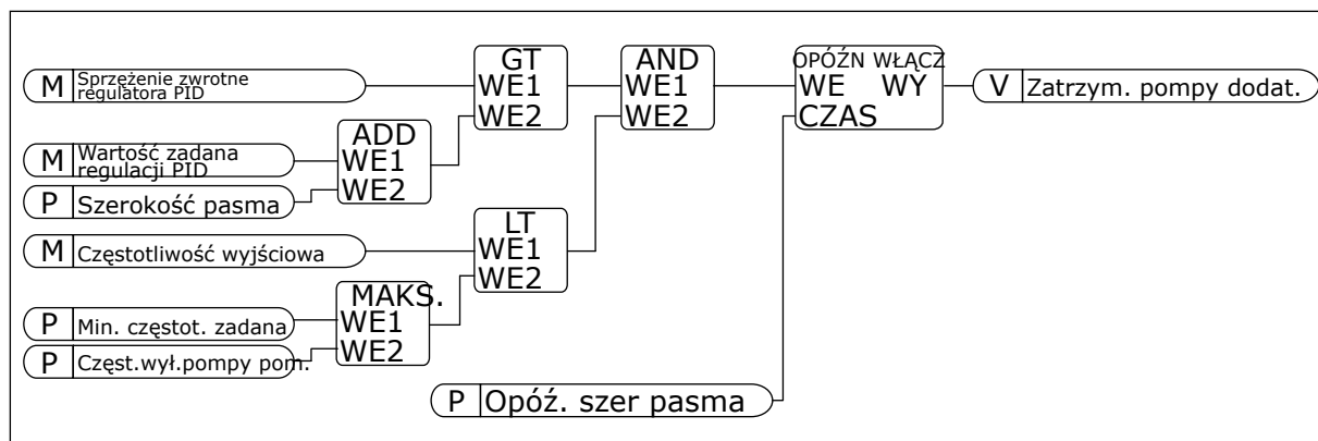
Rys. 102: Częst.wył.pompy pom.
