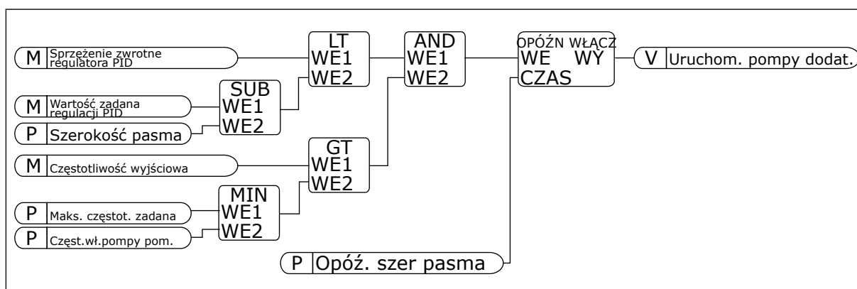
Rys. 101: Częst.wł.pompy pom.
