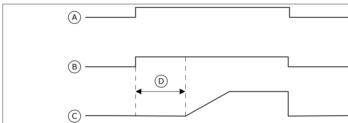
Fig. 106: A função Bomba priming
