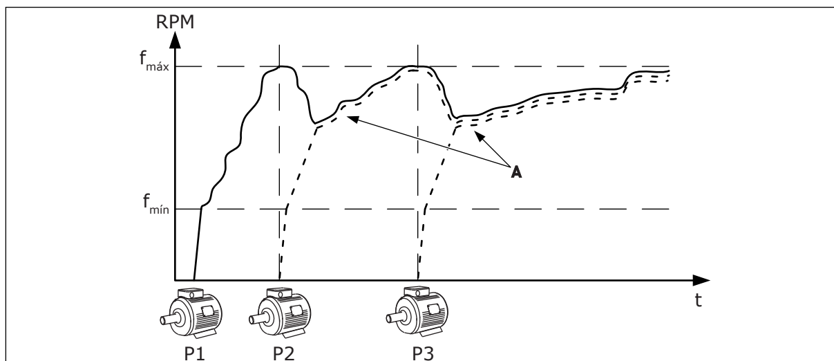
Fig. 14: Controle no modo Multisseguir
