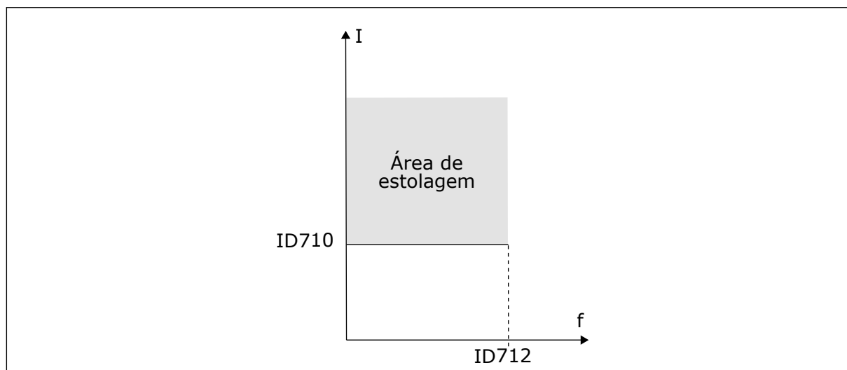
Fig. 68: As configurações das características da bloqueio do rotor
