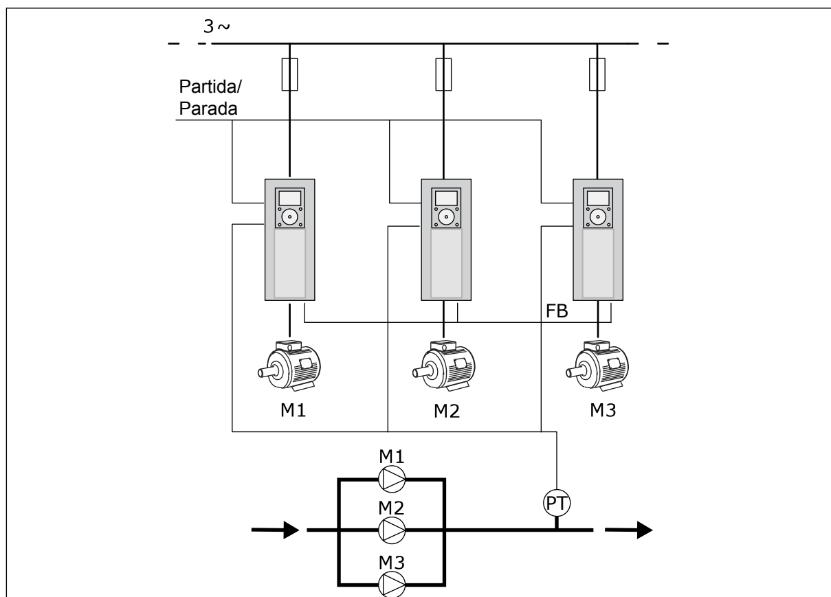
Fig. 13: Configuração Multibomba (multiconversor)
