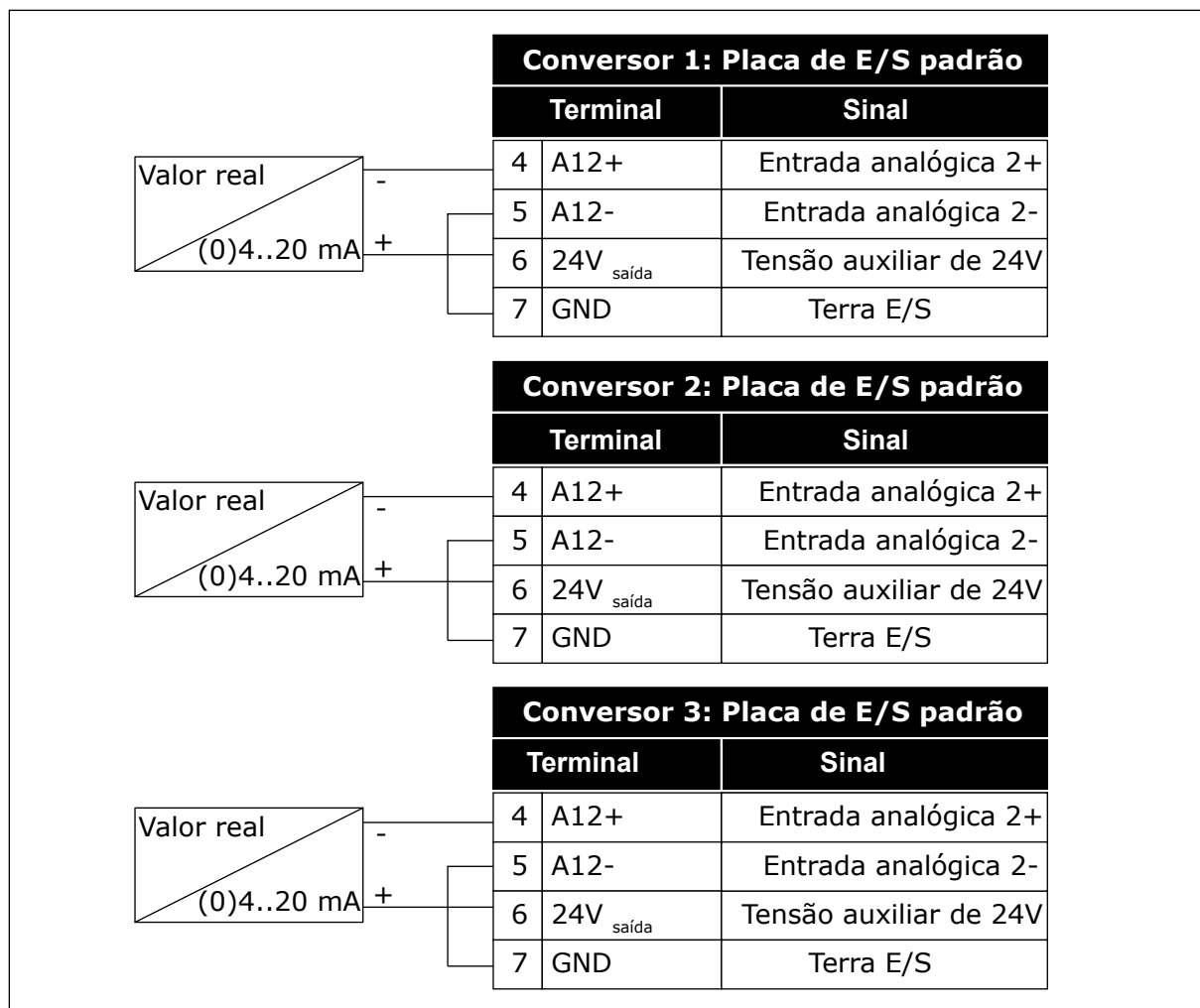
Fig. 94: Cabeamento dos sensores de realimentação para cada conversor
