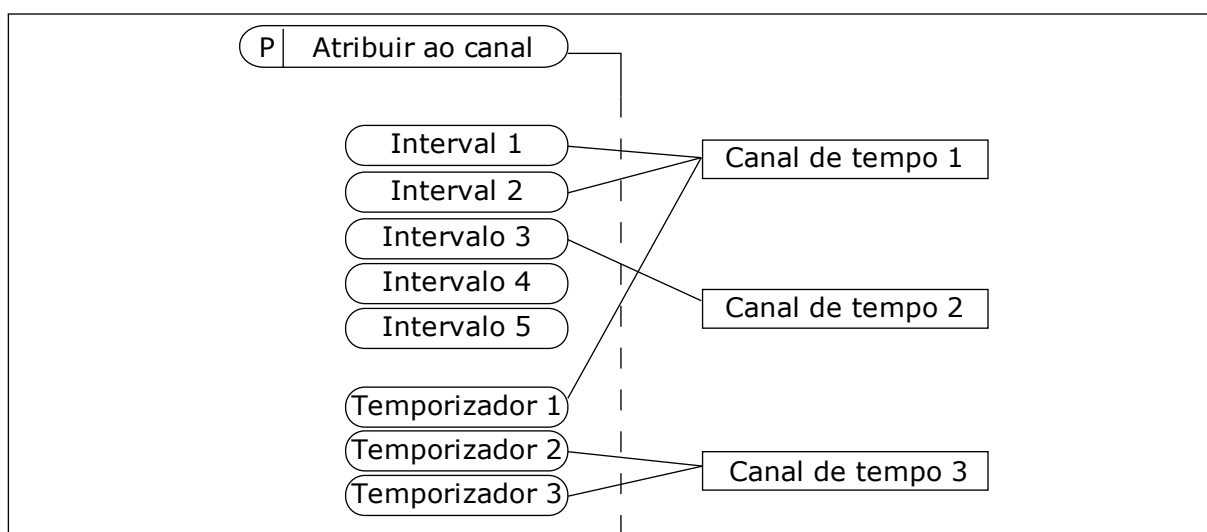
Fig. 73: A atribuição de intervalos e temporizadores aos canais de tempo é flexível. Cada intervalo e temporizador tem um parâmetro com o qual você pode atribuí-lo a um canal de tempo.
