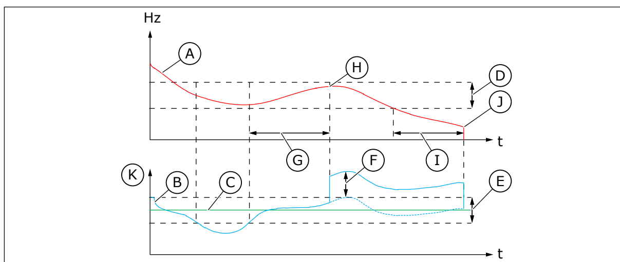
Fig. 88: Suspensão, sem demanda detectada
