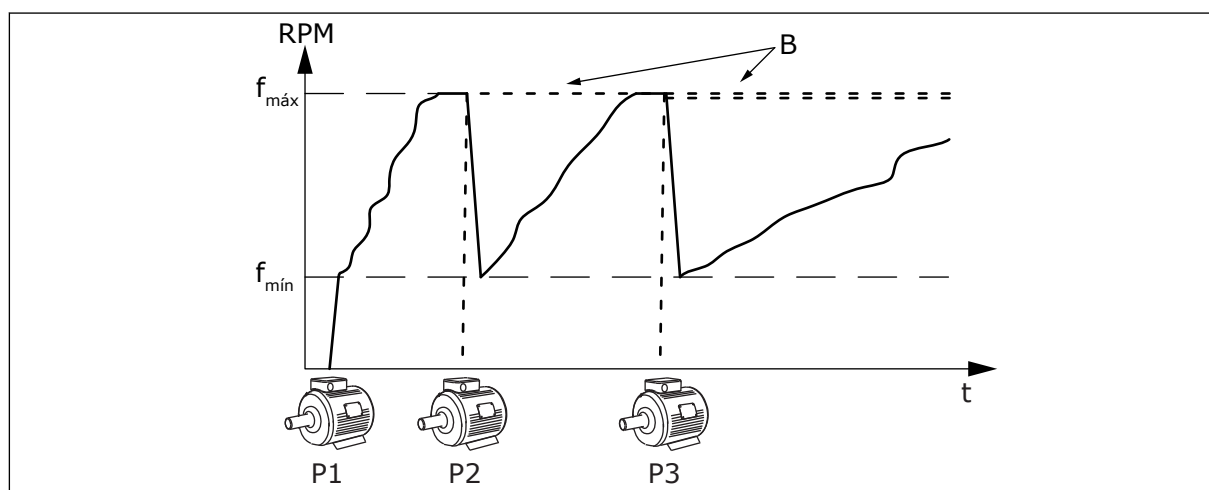
Fig. 91: Controle no modo de Conversor único
