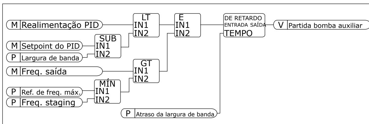
Fig. 101: Frequência de staging
