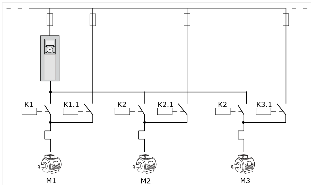
Fig. 10: Diagrama de controle, quando todos os motores estão configurados para sofrer troca automática
