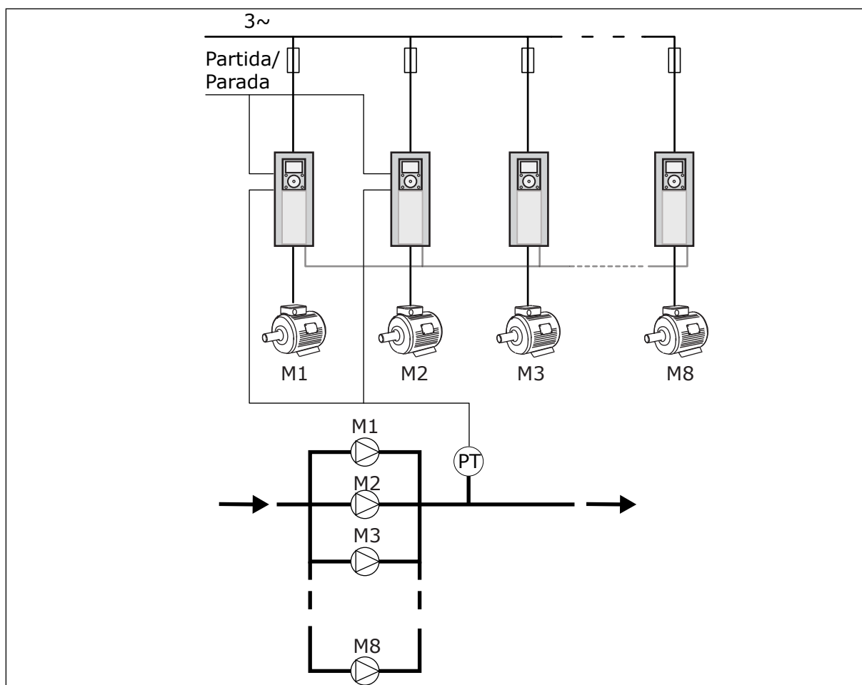
Fig. 90: Configuração de Multiconversor (PT = sensor de pressão)
