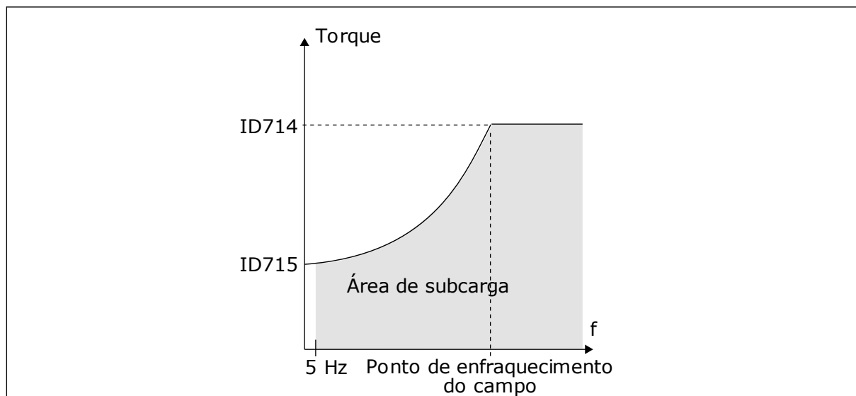
Fig. 69: Configuração da carga mínima
