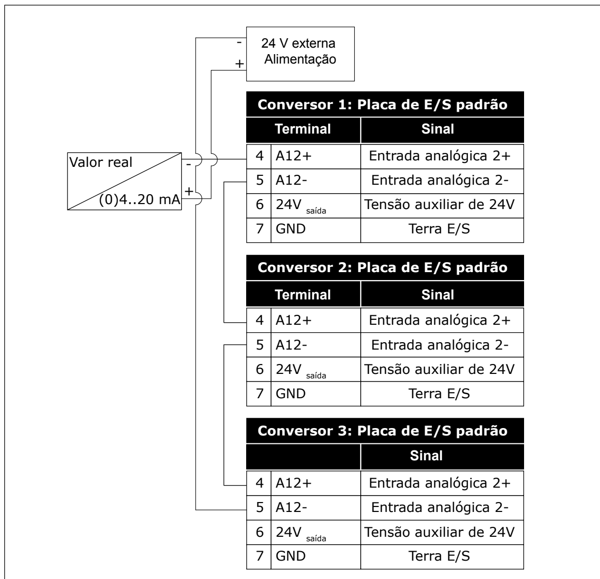
Fig. 96: Cabeamento do mesmo sensor para todos os conversores (alimentado por 24V externos)
