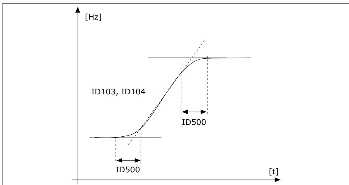
Fig. 49: A curva de aceleração/desaceleração (em forma de S)
