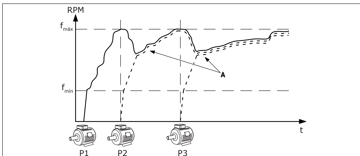
Fig. 92: Controle no modo Multisseguidor
