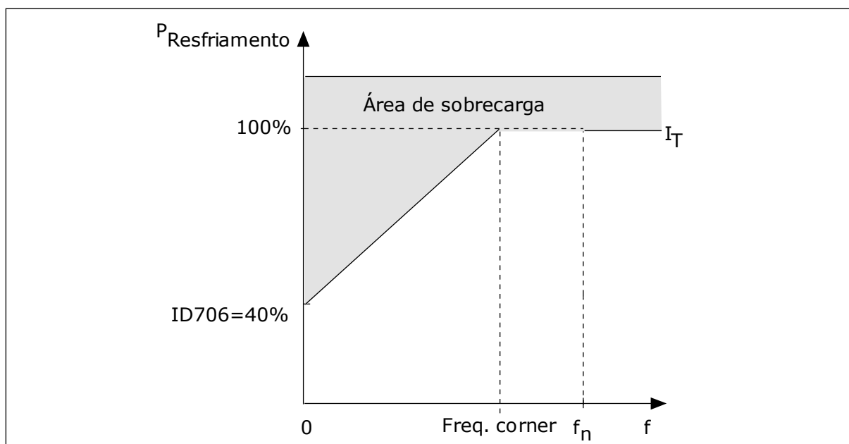
Fig. 65: Curva I_T da corrente térmica do motor
