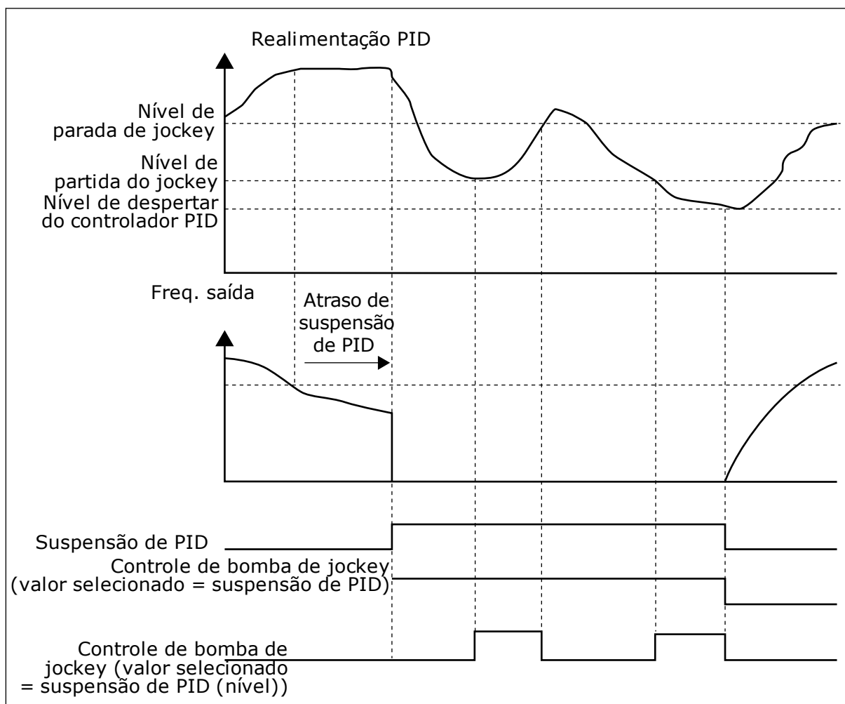
Fig. 105: A função Bomba jockey
