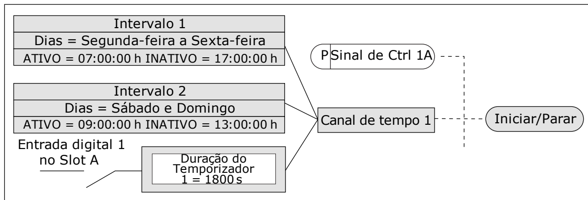
Fig. 78: O Canal de tempo 1 é usado como o sinal de controle para o comando de partida, em vez de uma entrada digital.
