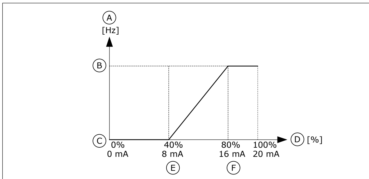
Fig. 59: Mín./máx. personalizados do sinal de AI1
