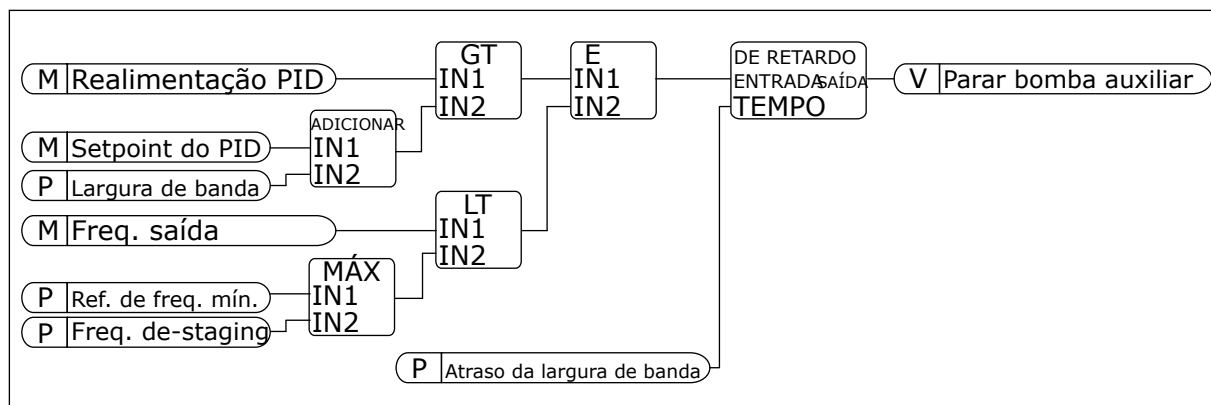
Fig. 102: Frequência de de-staging
