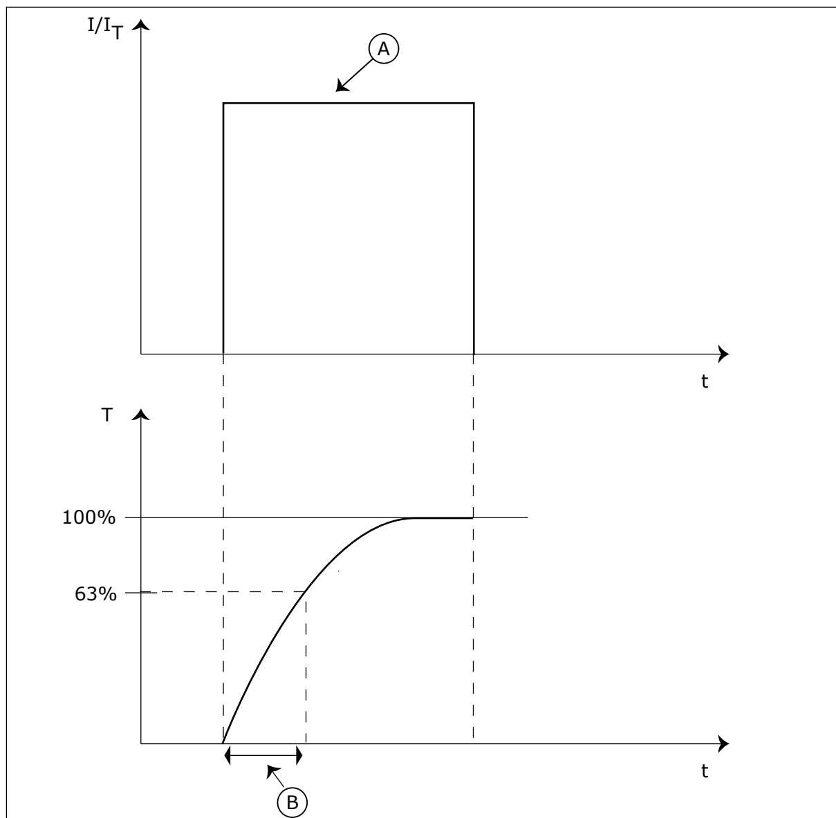
Fig. 66: A constante de tempo térmica do motor
