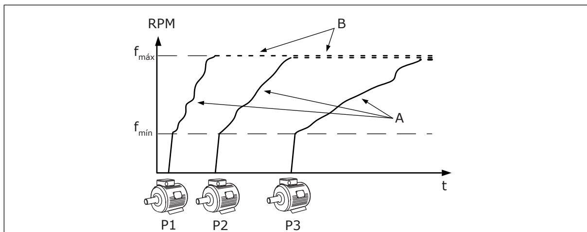
Fig. 93: Controle no modo Multimestre
