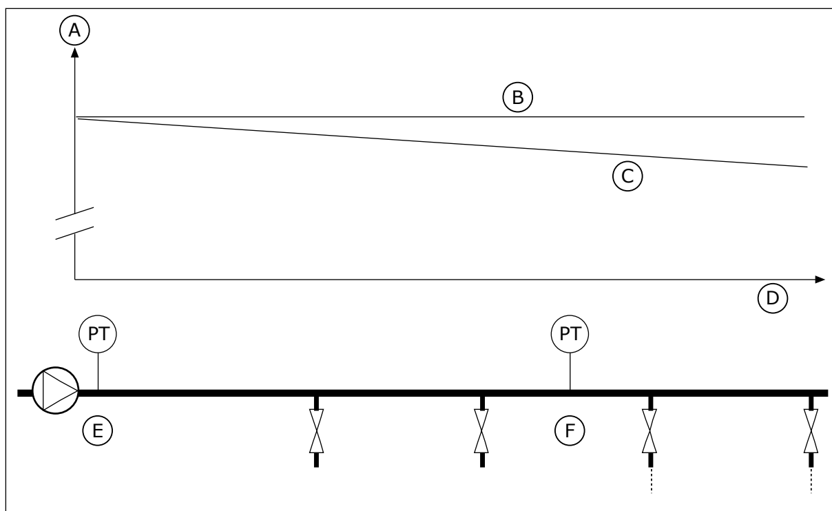
Fig. 84: A posição do sensor de pressão
