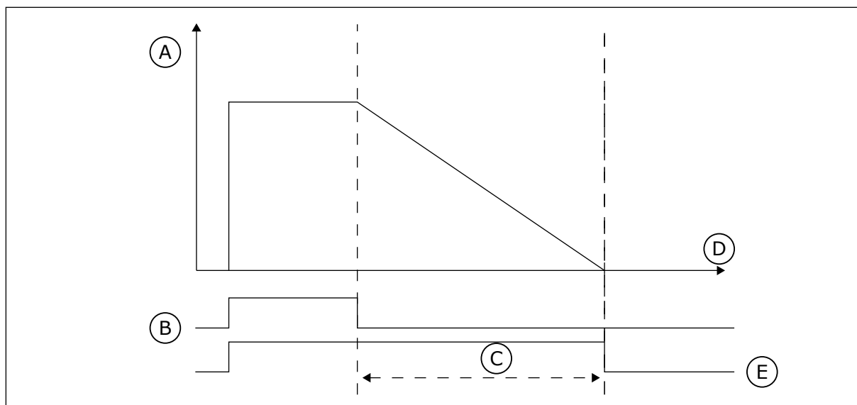
Fig. 74: O sinal de ativação virá de uma entrada digital ou de uma entrada digital virtual, como um canal de tempo. O temporizador conta para baixo a partir da borda em queda.
