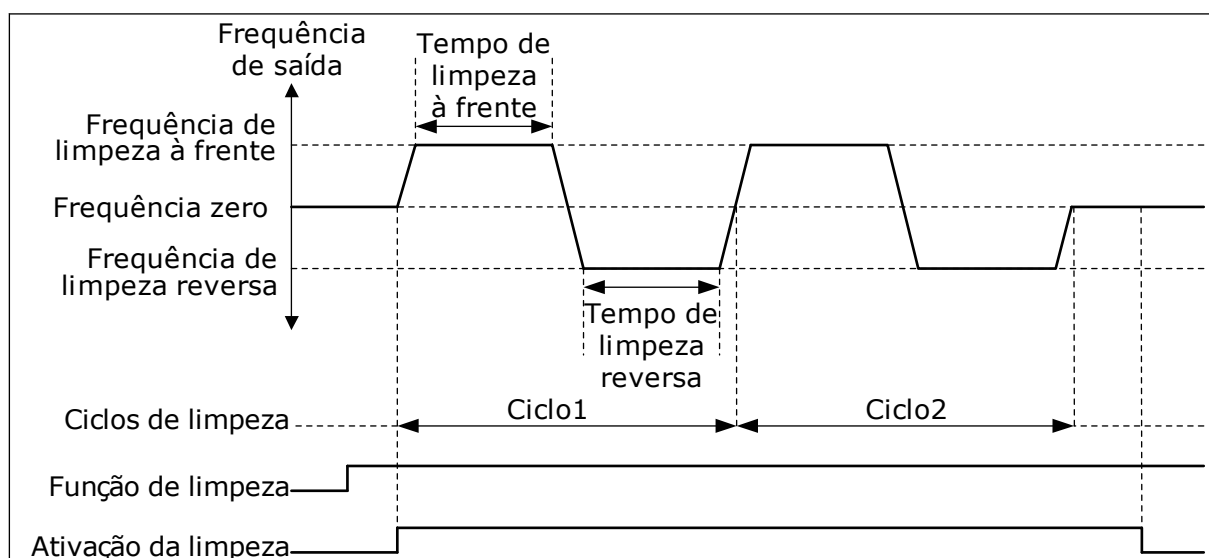
Fig. 104: A função Limpeza automática
