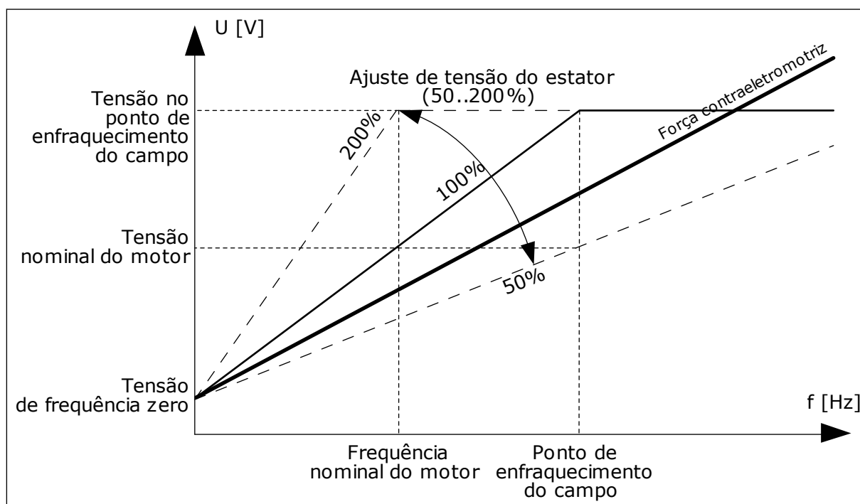
Fig. 37: O ajuste de tensão do estator
