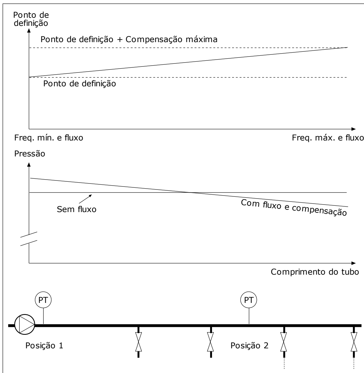
Fig. 85: Ativar ponto de definição 1 para compensação de perda de pressão
