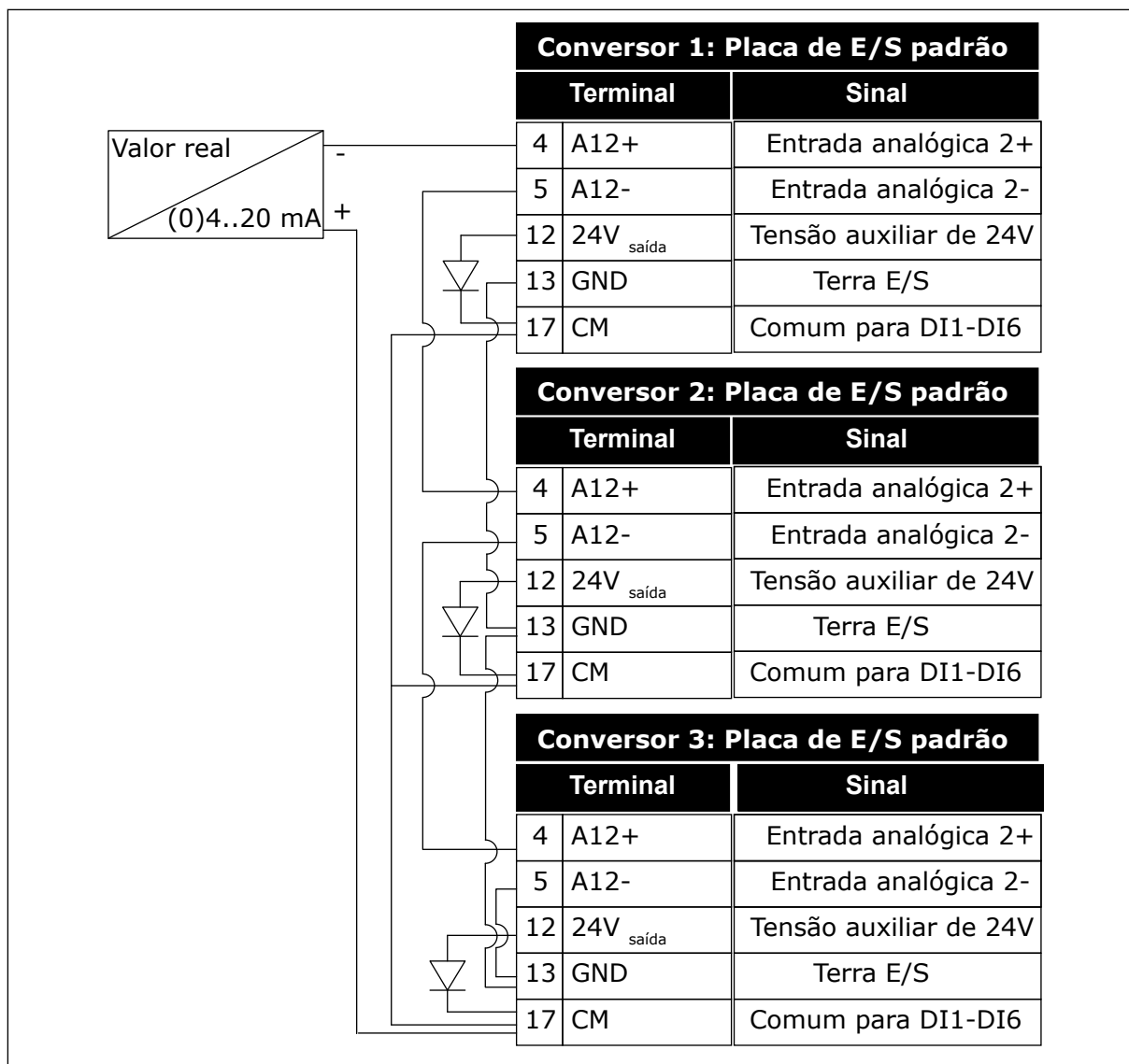
Fig. 95: Cabeamento do mesmo sensor para todos os conversores (alimentado pela placa de E/S do conversor)
