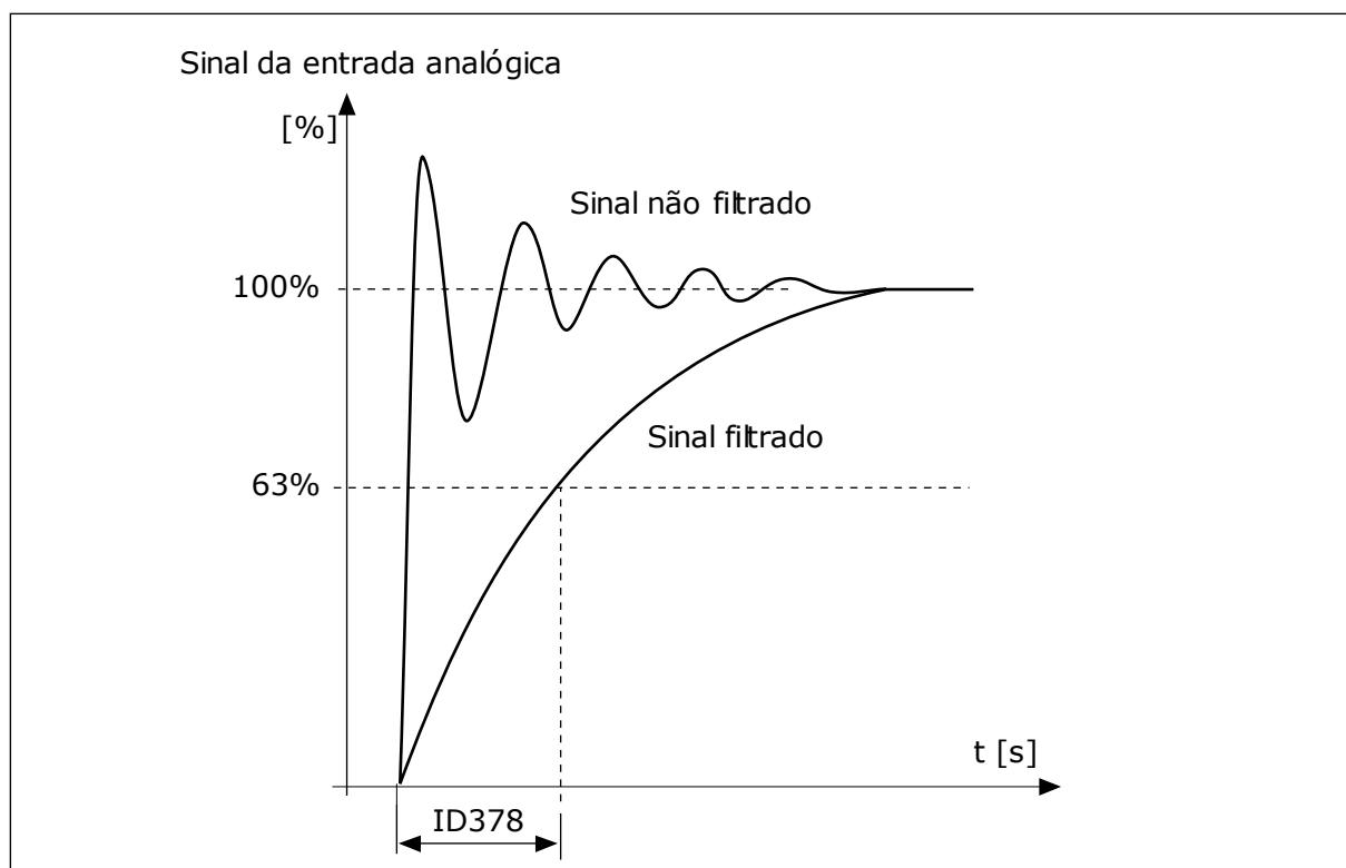
Fig. 56: A filtragem do sinal de AI1
