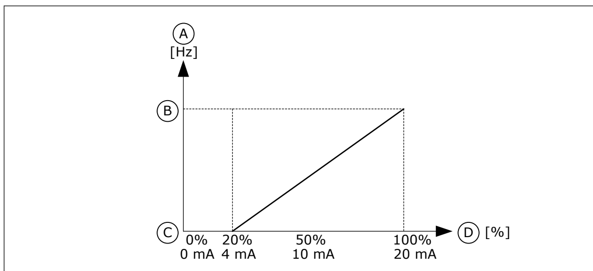
Fig. 58: A faixa de sinal da entrada analógica, seleção '1'
