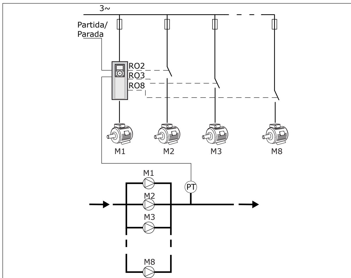
Fig. 89: Configuração de conversor único (PT = sensor de pressão)
