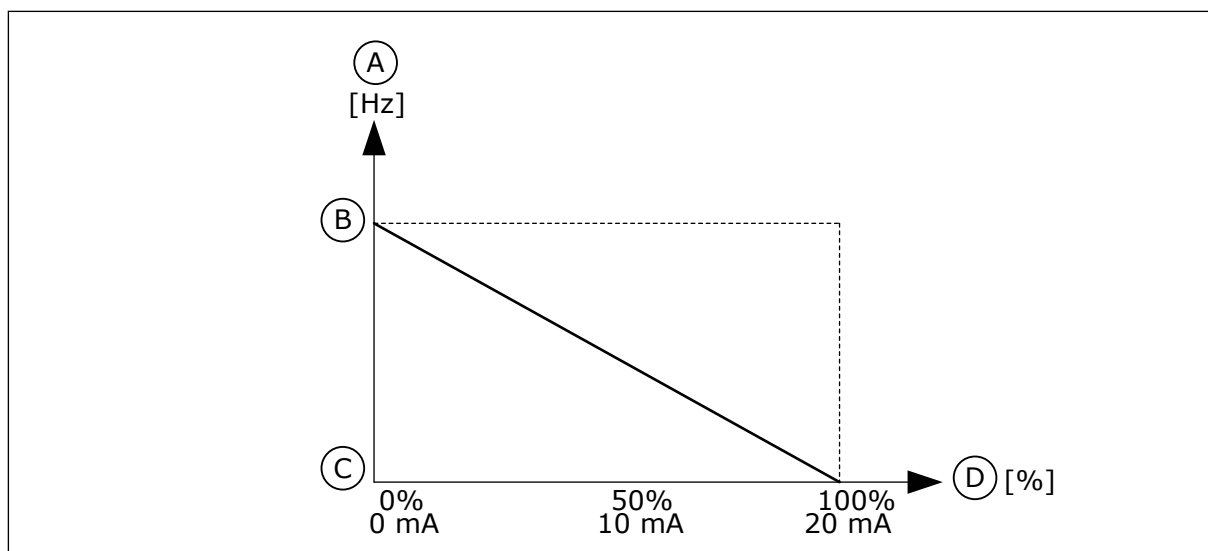
Fig. 61: Inversão do sinal de AI1, seleção 1
