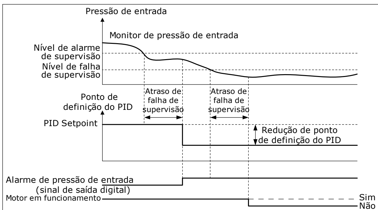
Fig. 87: A função de supervisão de pressão de entrada
