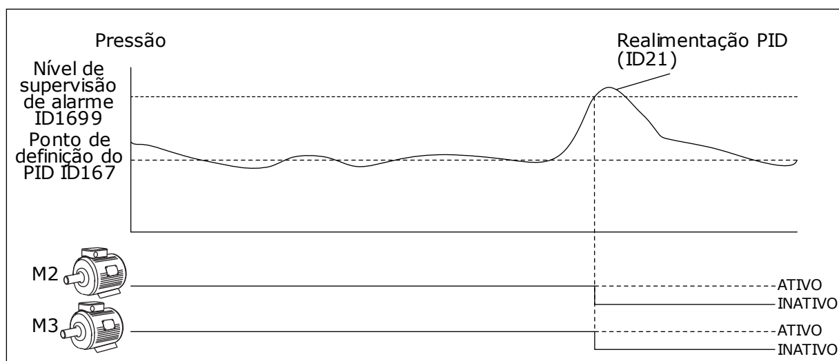
Fig. 100: A função de supervisão de sobrepressão
