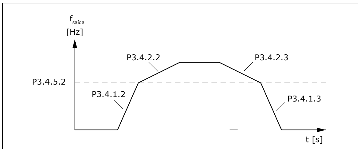
Fig. 50: Ativação da rampa 2 quando a frequência de saída exceder o nível do limiar. (P3.4.5.2 = Limiar de frequência da rampa, P3.4.1.2 = Tempo de aceleração 1, P3.4.2.2 = Tempo de aceleração 2, P3.4.1.3 = Tempo de desaceleração 1, P3.4.2.3 = Tempo de desaceleração 2)
