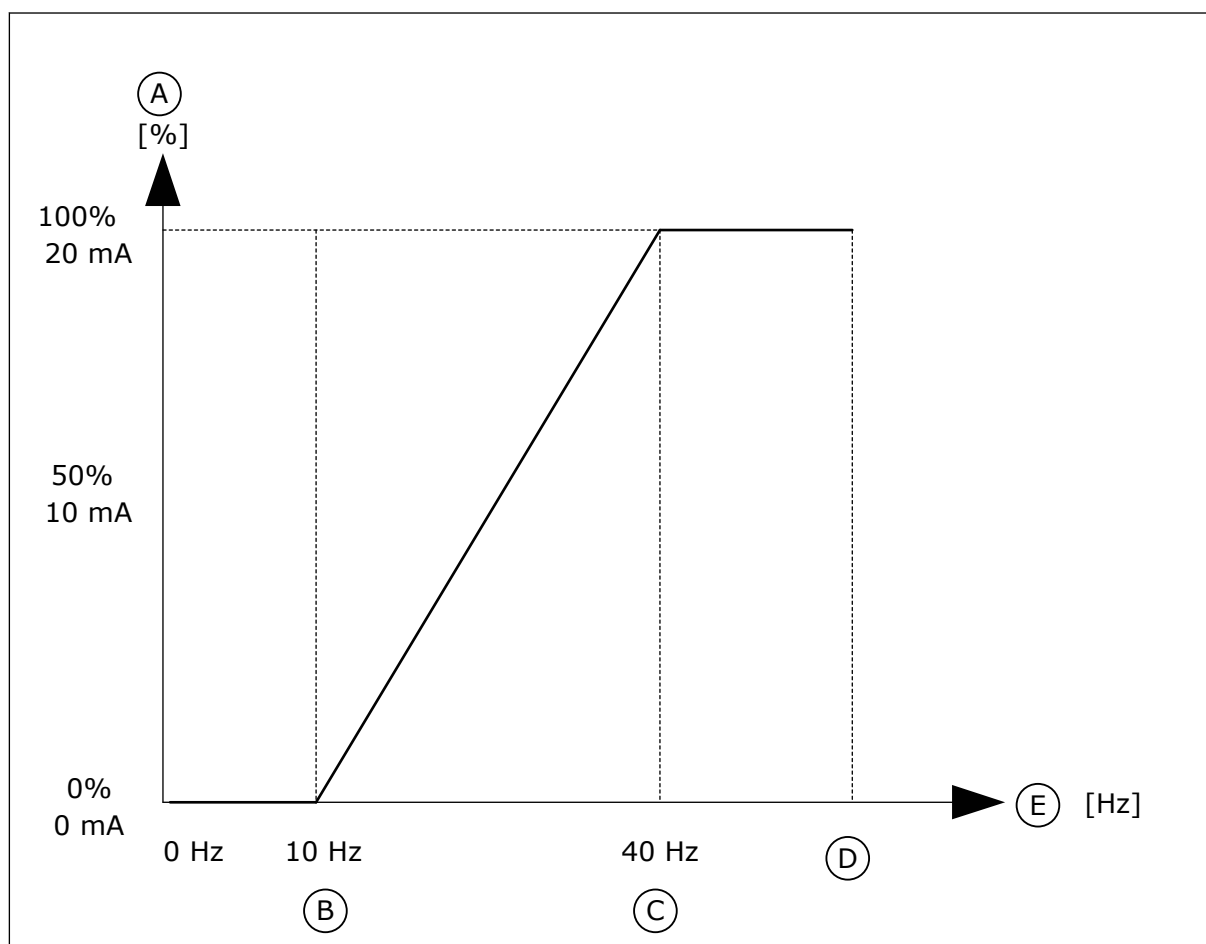
Fig. 62: A escala do sinal de AO1
