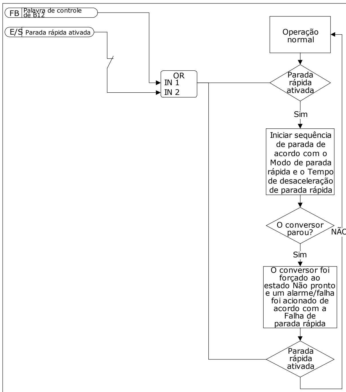
Fig. 71: A lógica da parada rápida
