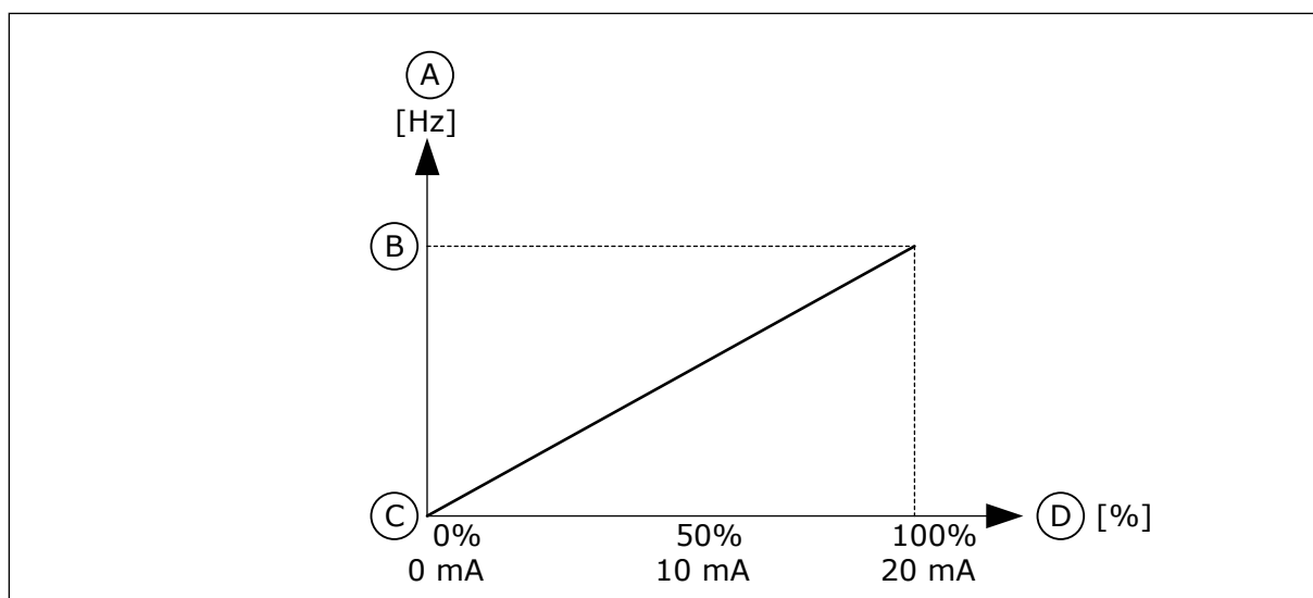
Fig. 57: A faixa de sinal da entrada analógica, seleção '0'
