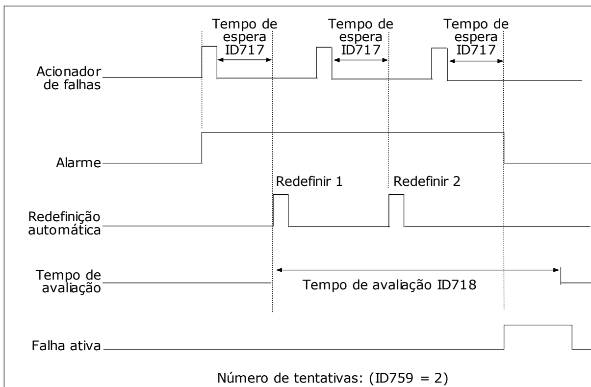
Fig. 72: A função Reset automático
