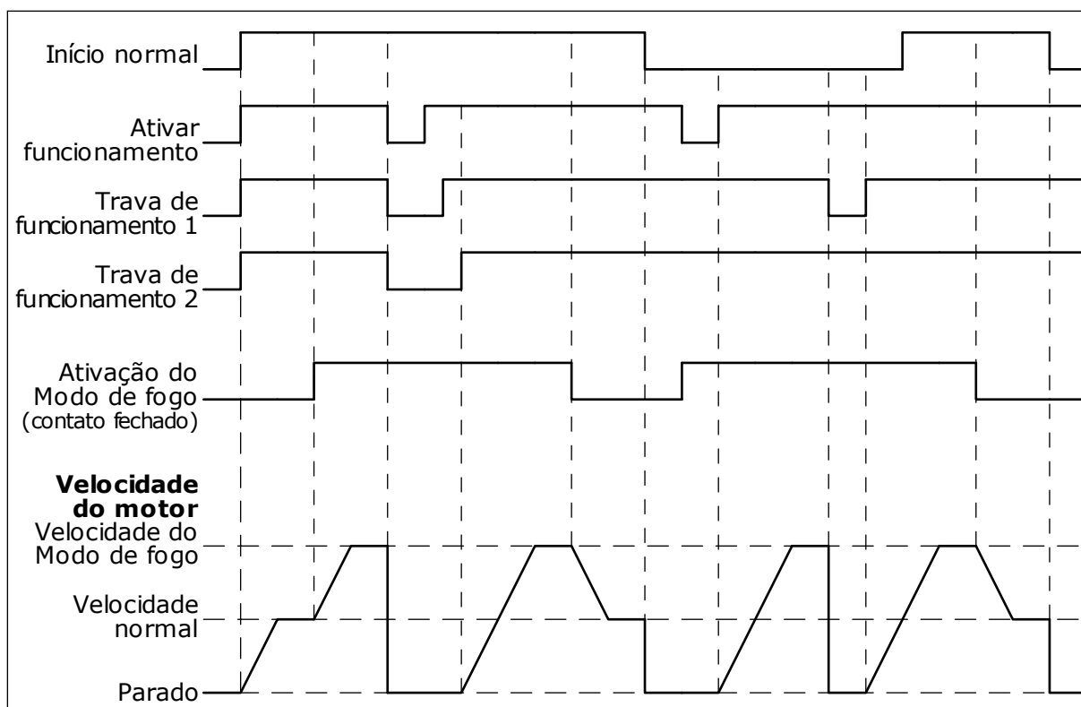
Fig. 103: A função do Modo de incêndio
