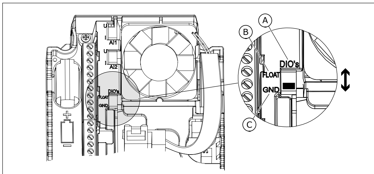
Fig. 5: Comutatorul DIP
