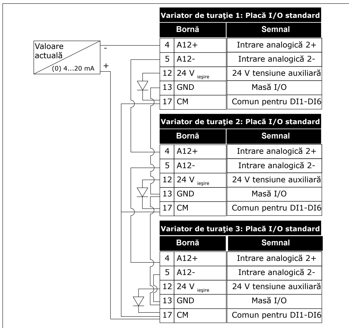
Fig. 95: Cablarea aceluiași senzor pentru toate variatoarele de turație (alimentat de la placa I/O a variatorului de turație)
