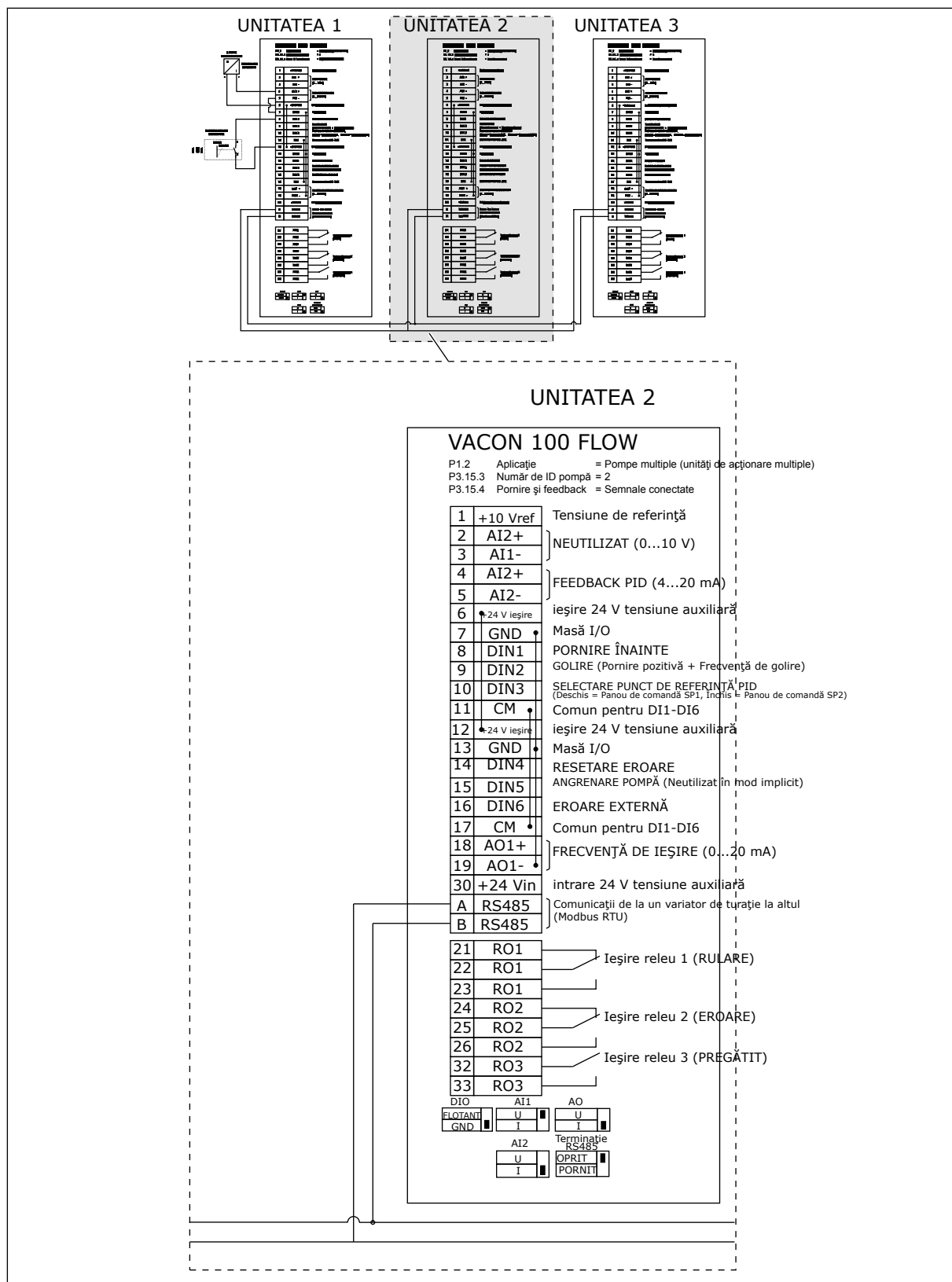
Fig. 31: Diagramă de cablaj electric a sistemului Pompe multiple (acționare multiplă), exemplul 5B
