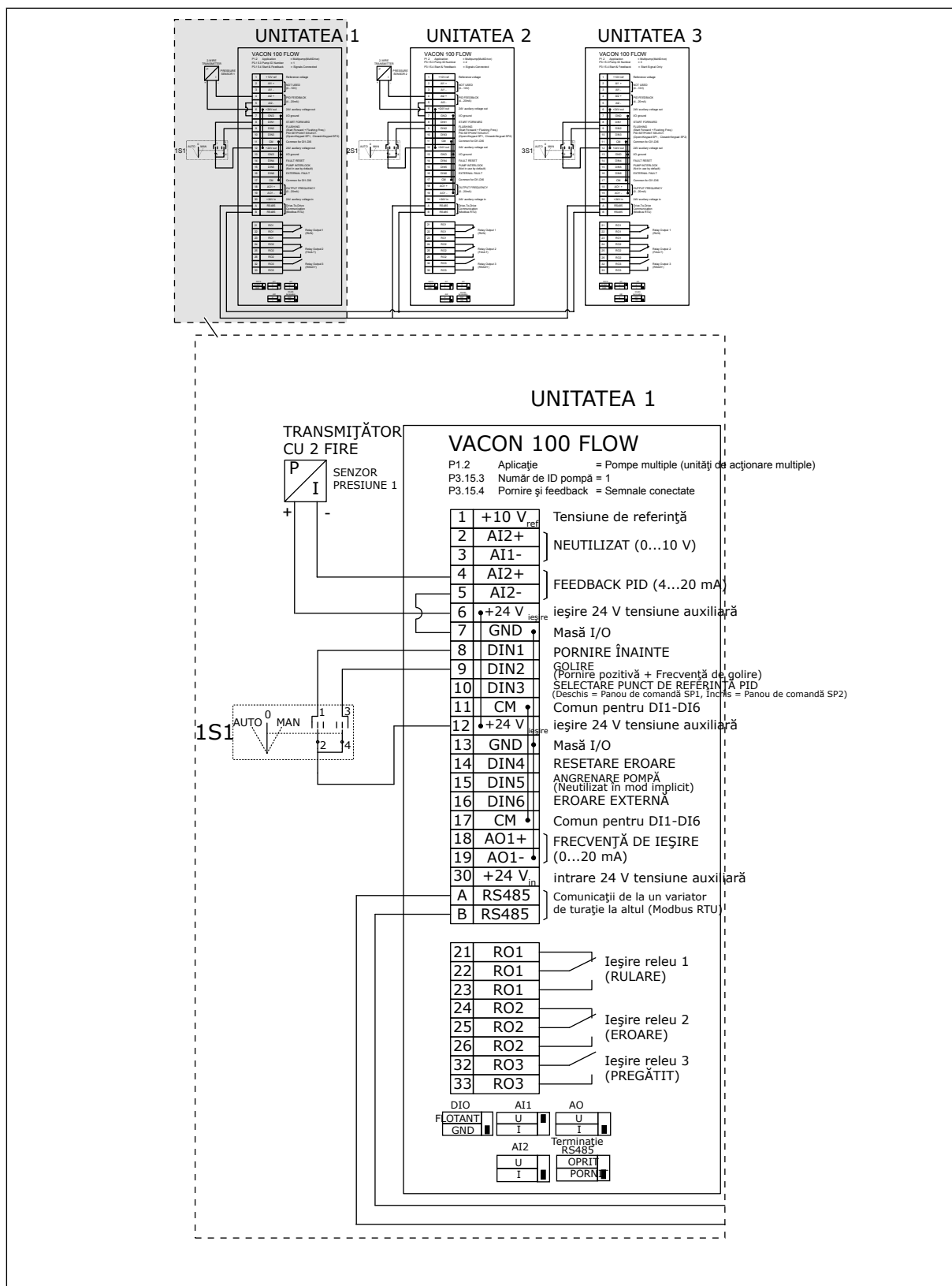
Fig. 24: Diagramă de cablaj electric a sistemului Pompe multiple (acționare multiplă), exemplul 3A
