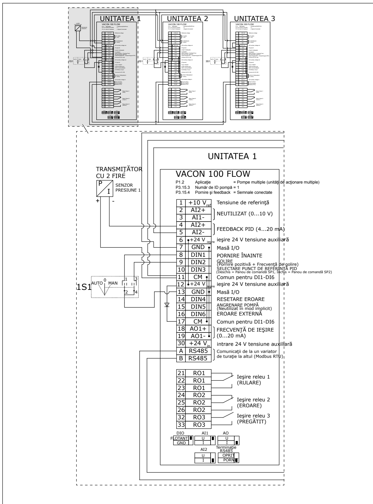
Fig. 21: Diagramă de cablaj electric a sistemului Pompe multiple (acționare multiplă), exemplul 2A
