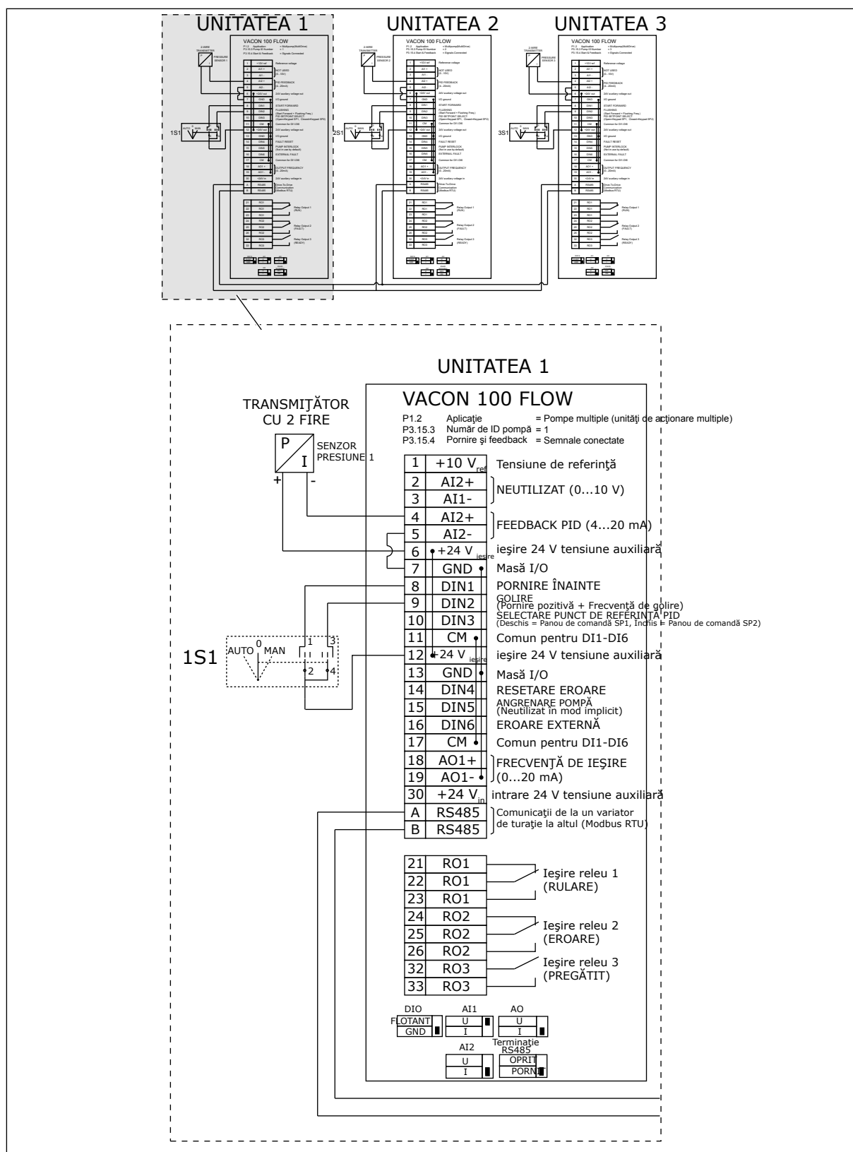
Fig. 18: Diagramă de cablaj electric a sistemului Pompe multiple (acționare multiplă), exemplul 1A
