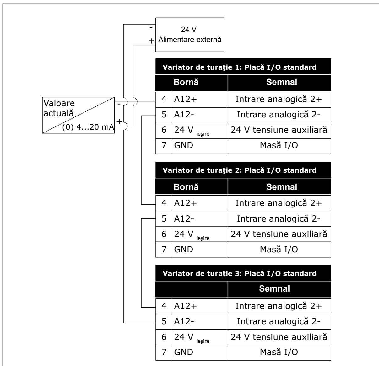
Fig. 96: Cablarea aceluiasi senzor pentru toate variatoarele de turație (alimentat de la o sursă externă de 24 V)
