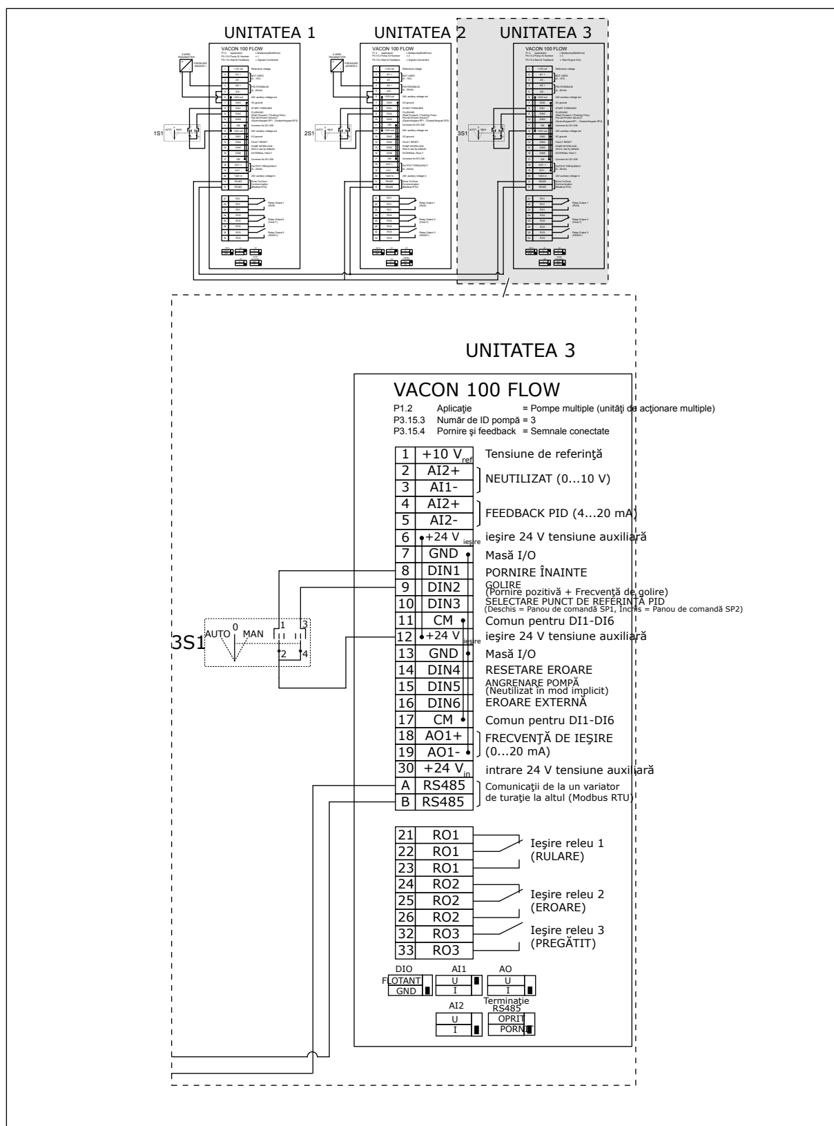
Fig. 26: Diagramă de cablaj electric a sistemului Pompe multiple (acționare multiplă), exemplul 3C
