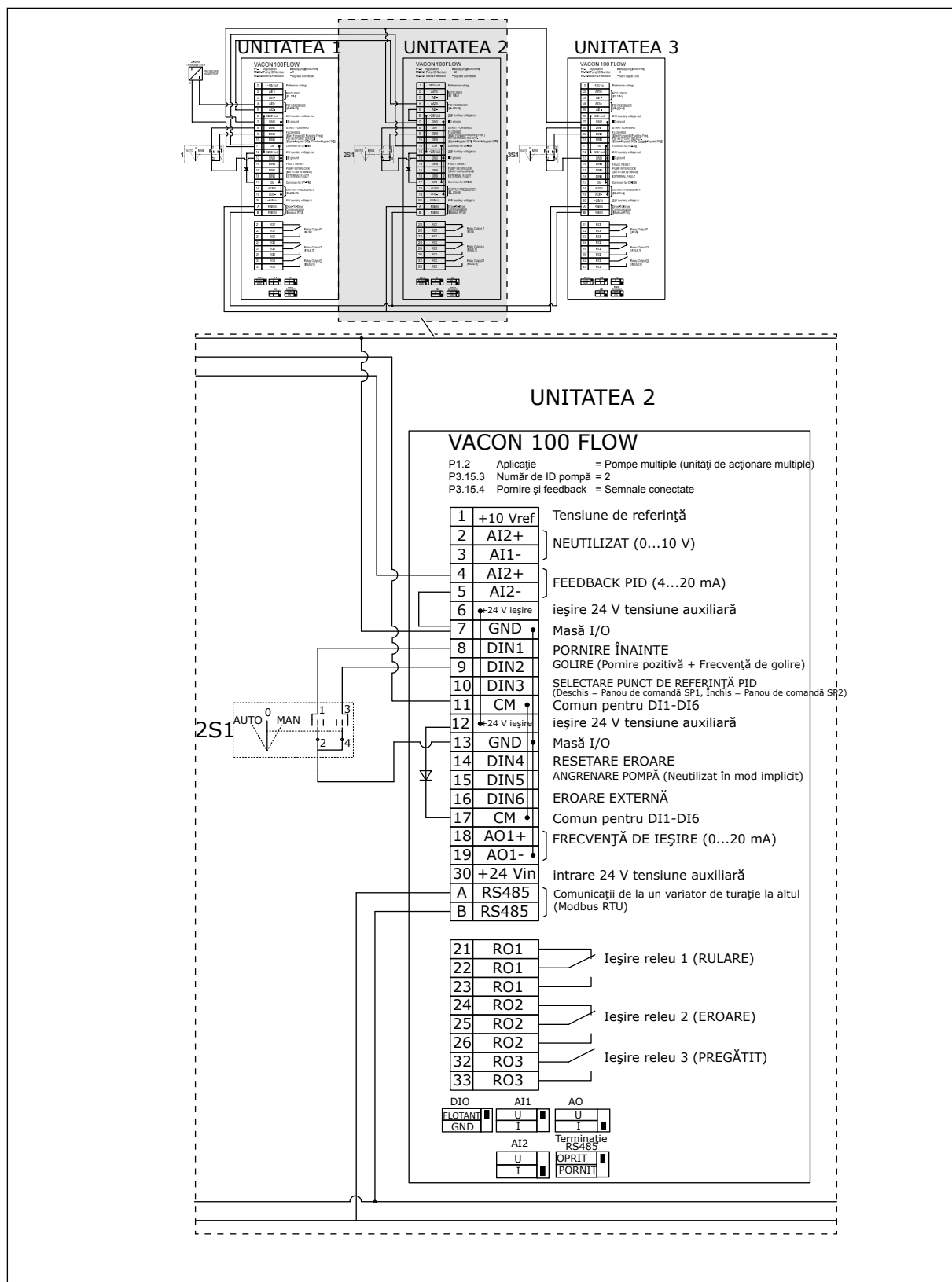
Fig. 28: Diagramă de cablaj electric a sistemului Pompe multiple (acționare multiplă), exemplul 4B
