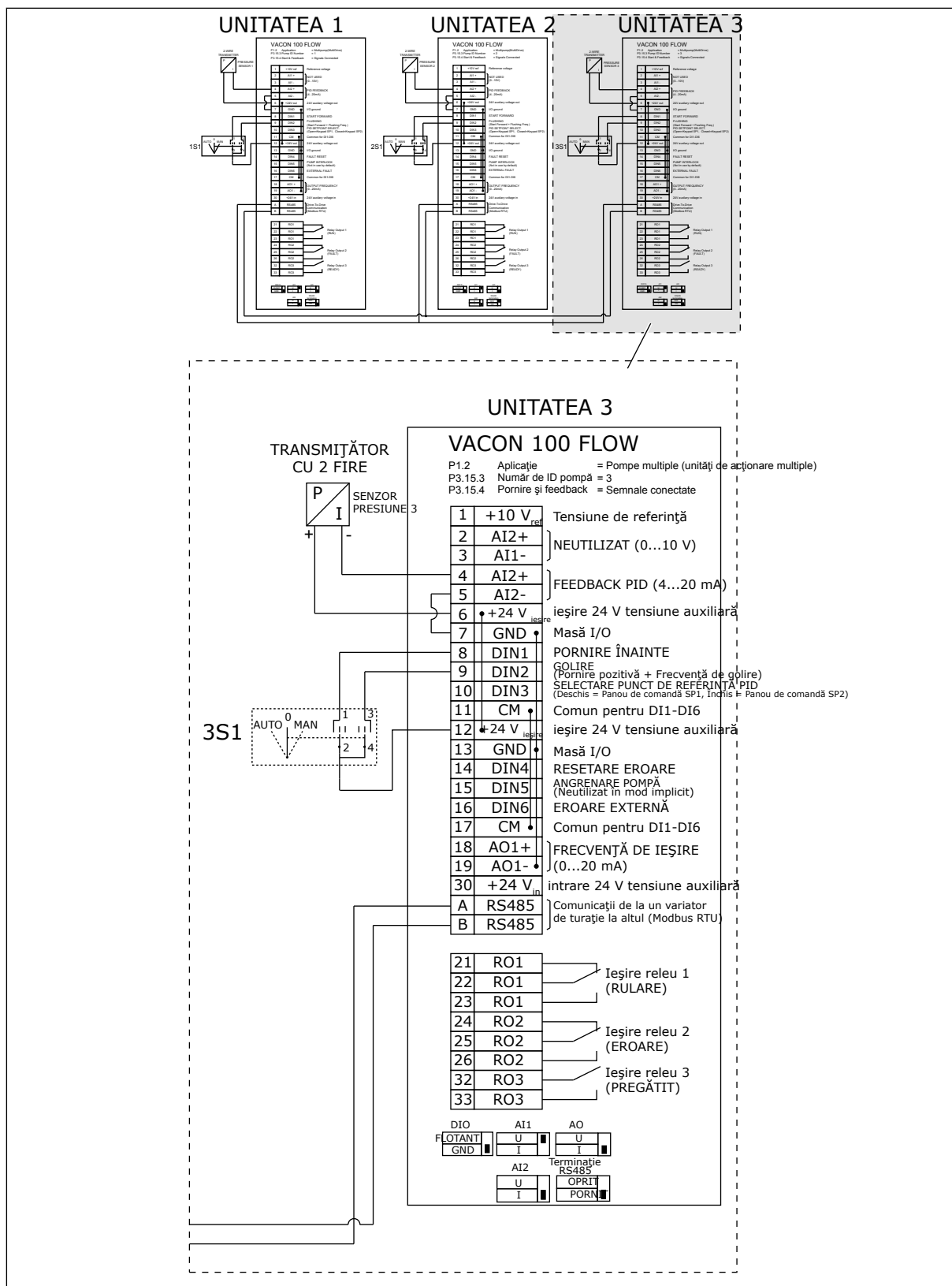
Fig. 20: Diagramă de cablaj electric a sistemului Pompe multiple (acționare multiplă), exemplul 1C
