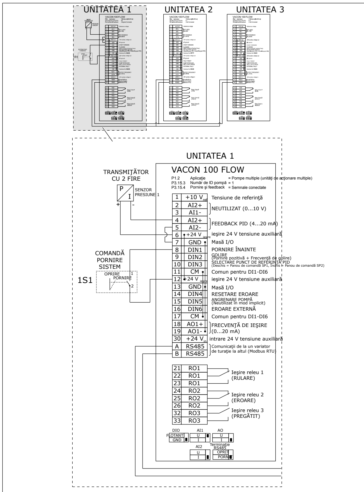
Fig. 30: Diagramă de cablaj electric a sistemului Pompe multiple (acționare multiplă), exemplul 5A
