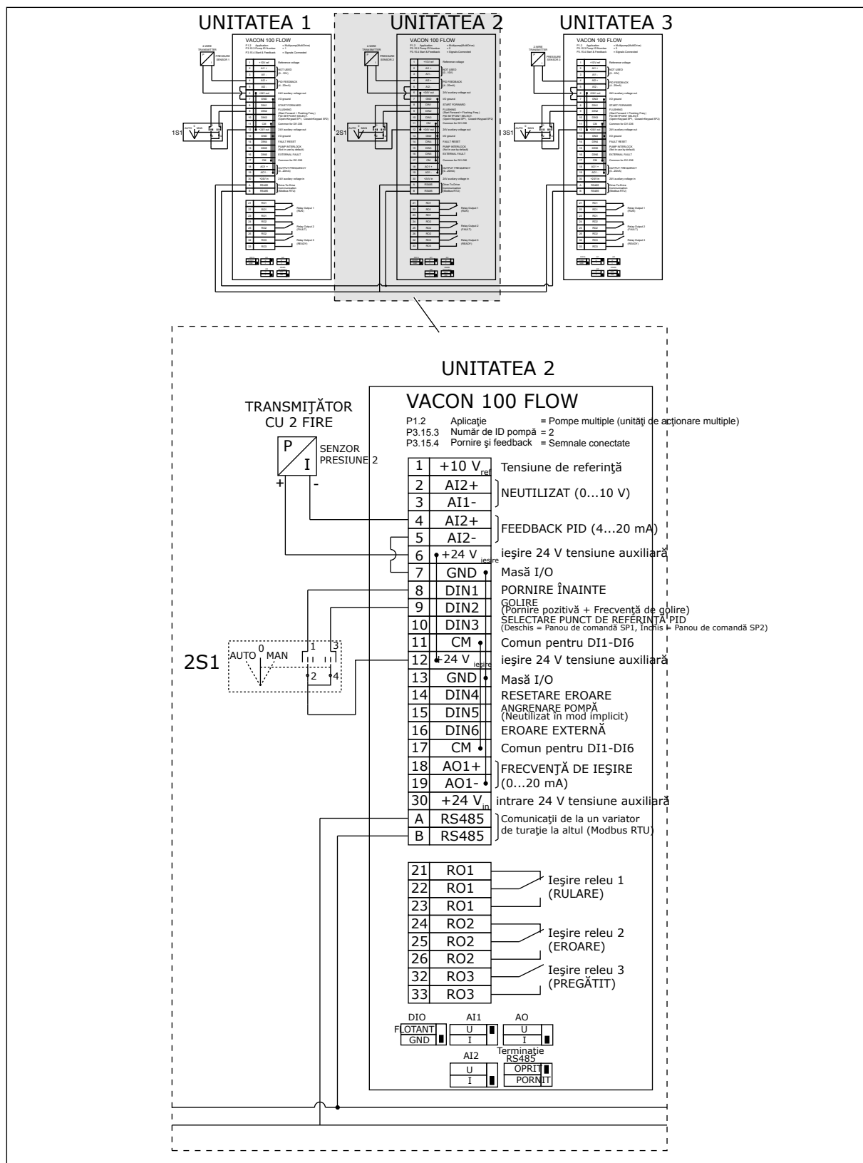
Fig. 19: Diagramă de cablaj electric a sistemului Pompe multiple (acționare multiplă), exemplul 1B
