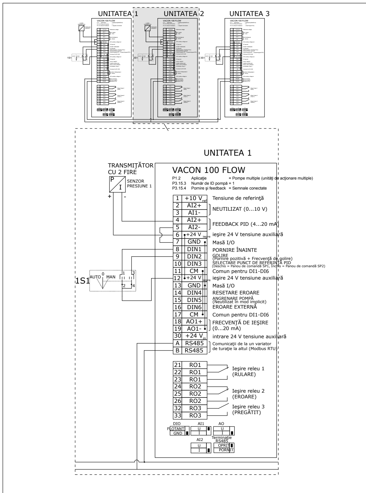
Fig. 25: Diagramă de cablaj electric a sistemului Pompe multiple (acționare multiplă), exemplul 3B
