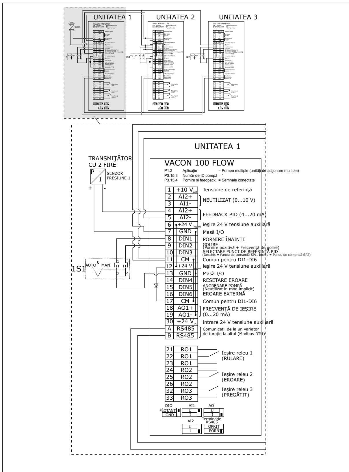
Fig. 27: Diagramă de cablaj electric a sistemului Pompe multiple (acționare multiplă), exemplul 4A
