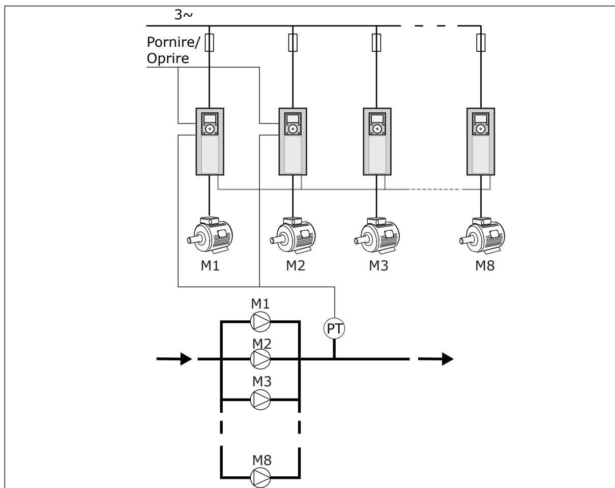
Fig. 90: Configurație cu unități de acționare multiple (PT = senzor de presiune)
