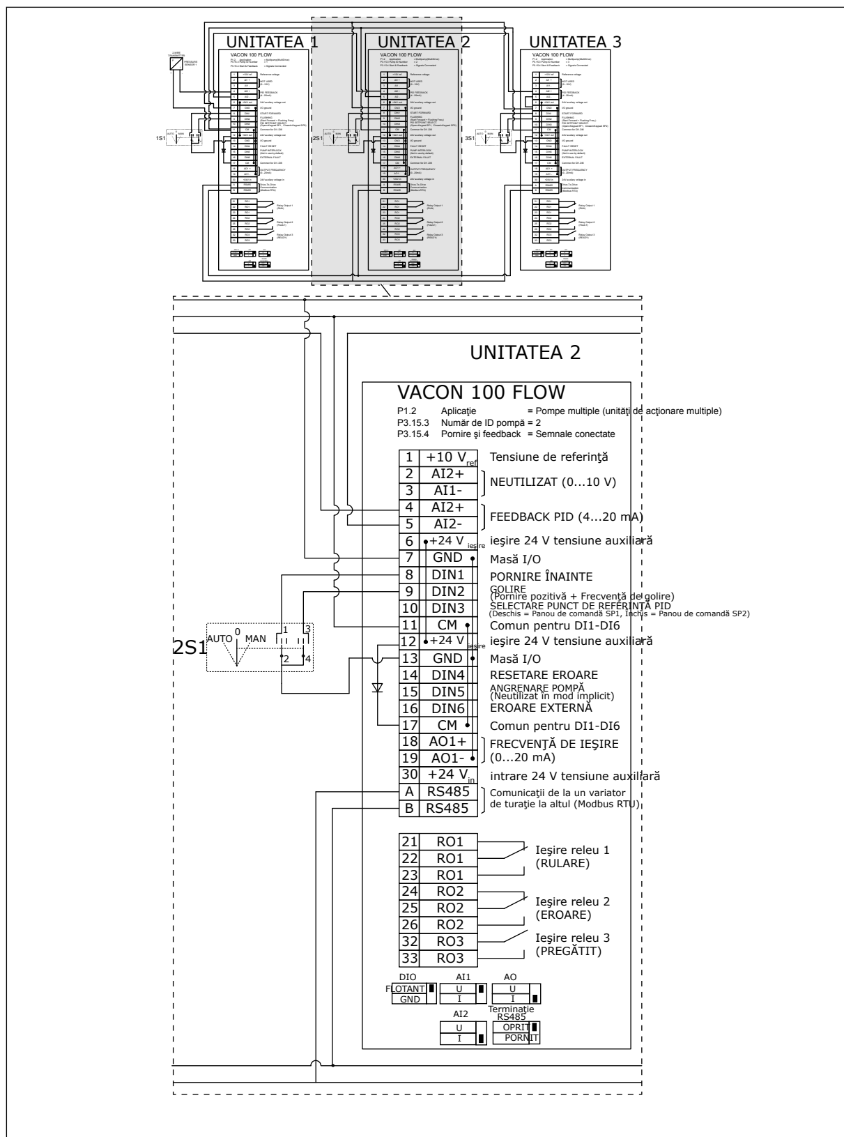
Fig. 22: Diagramă de cablaj electric a sistemului Pompe multiple (acționare multiplă), exemplul 2B
