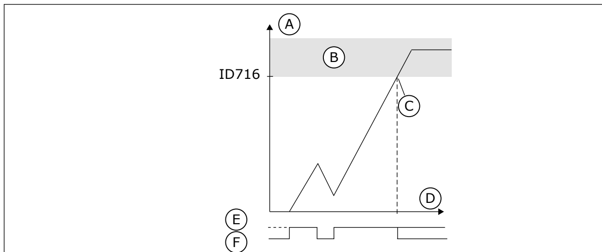
图 70: 欠载时间计数器功能
