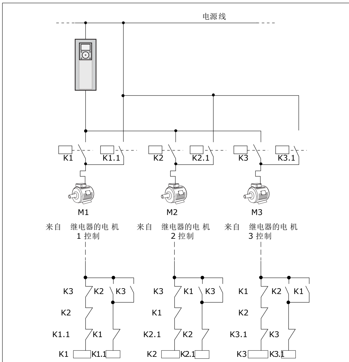
图 98: 选择 1
