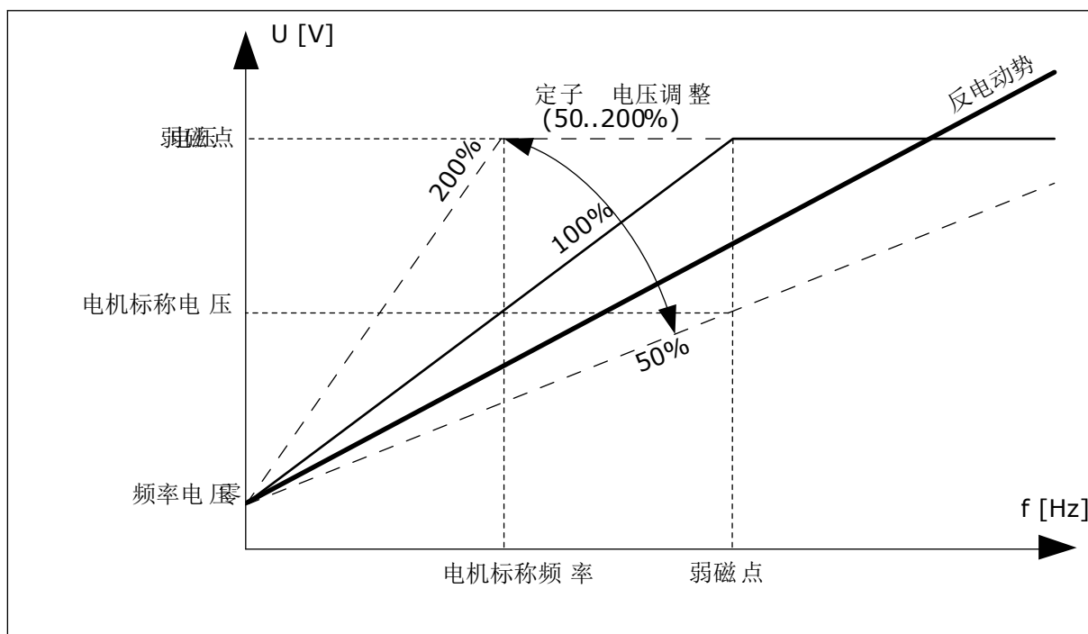
图 37: 定子电压调整
