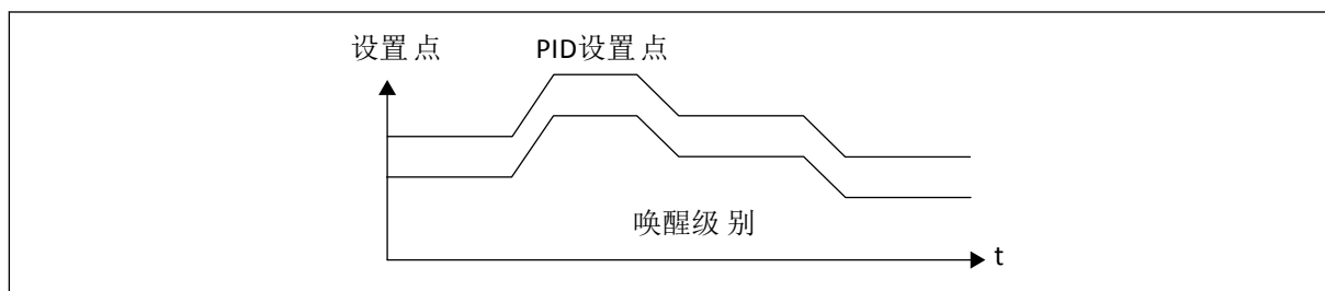
图 82: 唤醒模式：相对设置点
