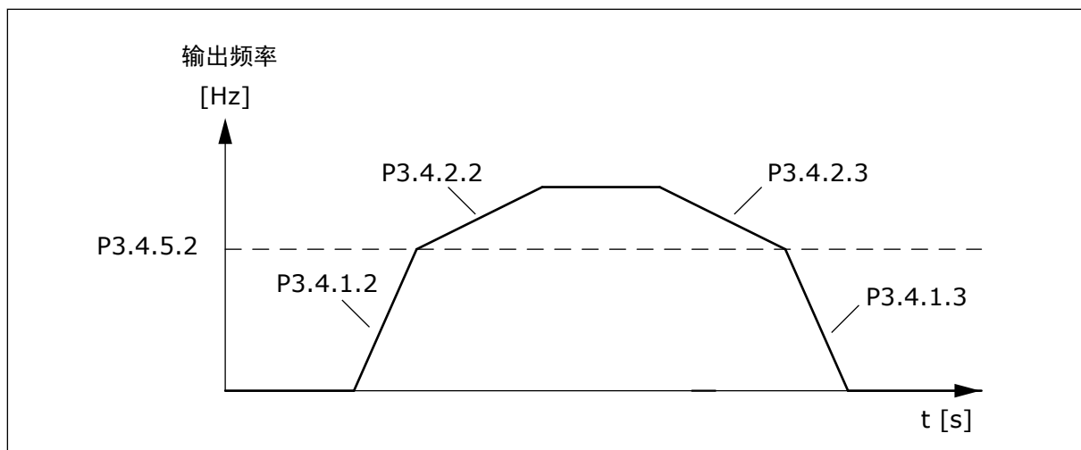
图 50: 当输出频率超出阈值级别时, 将激活斜坡 2。( P3.4.5.2 = 斜坡阈值频率、P3.4.1.2 = 加速时间 1、P3.4.2.2 = 加速时间 2、P3.4.1.3 = 减速时间 1、P3.4.2.3 = 减速时间 2 )
