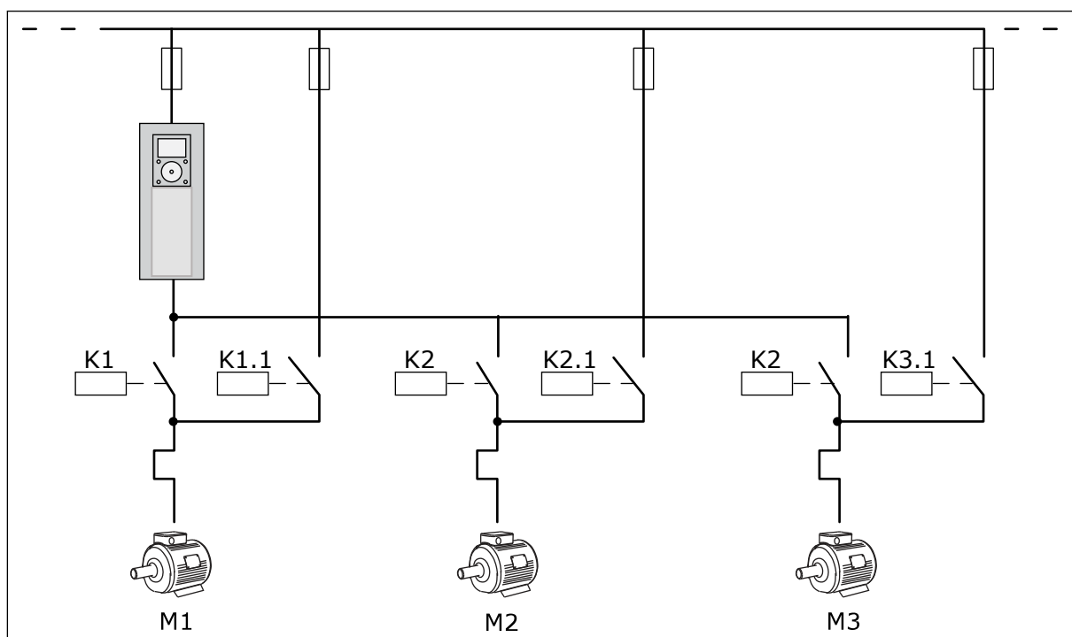
图 10: 所有电机均配置为自动切换的控制图
