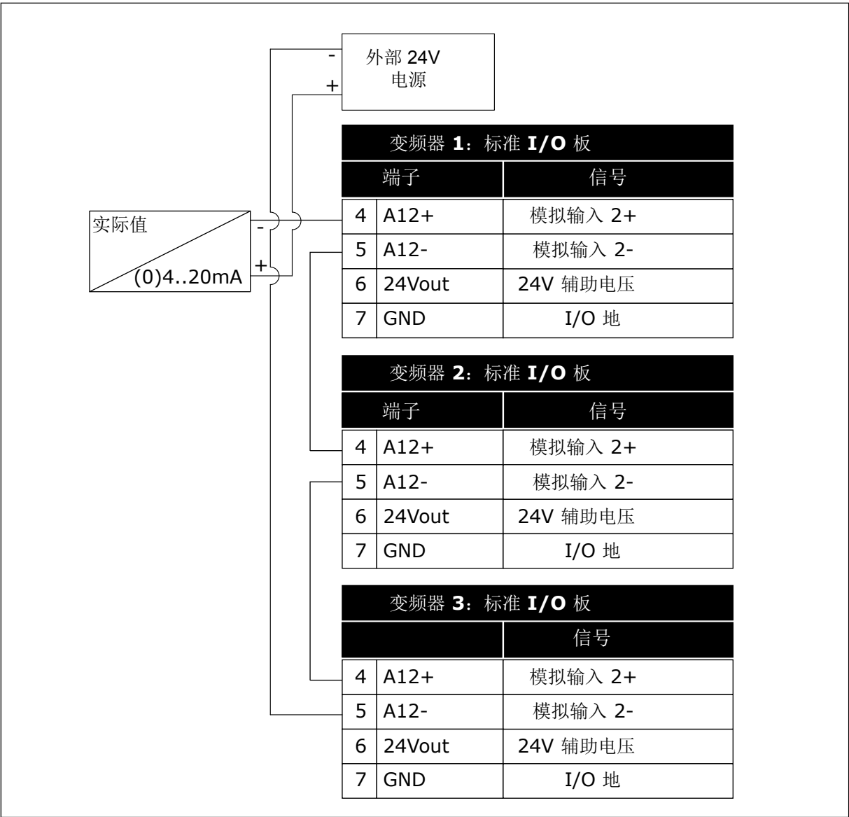
图 96: 所有变频器的相同传感器的接线 ( 从外部 24V 供电 )
