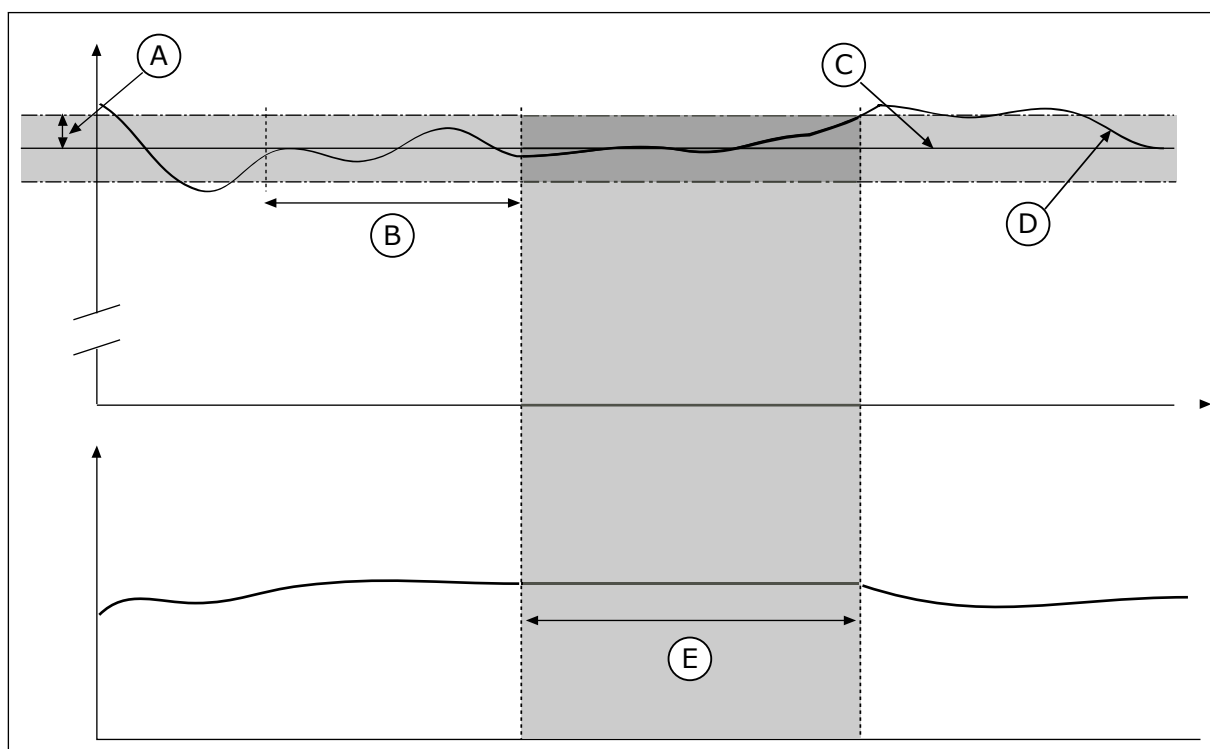
图 79: 死区功能
