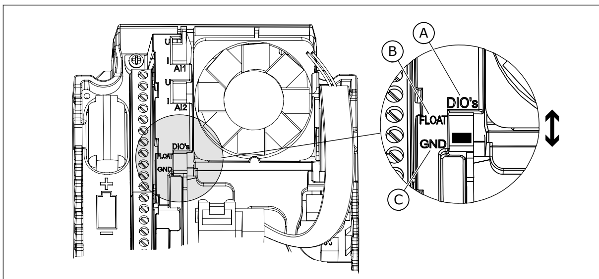
图 97: 隔离 DIP 开关
