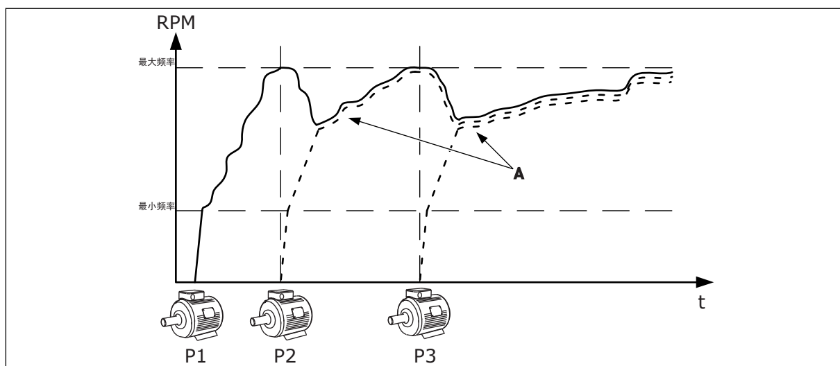
图 92: Multifollower 模式下的控制
