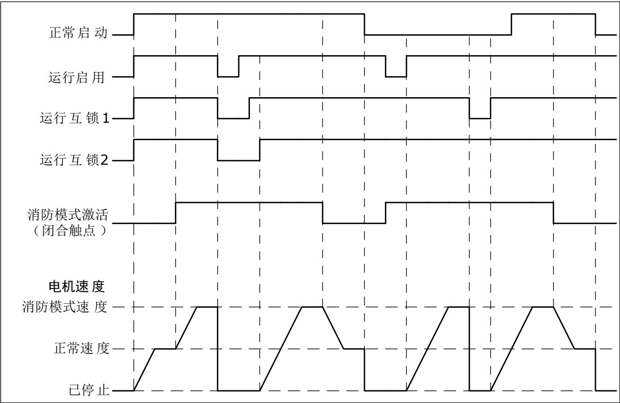
图 103: 消防模式功能
