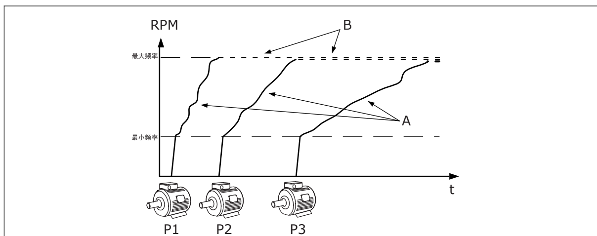
图 93: Multimaster 模式下的控制
