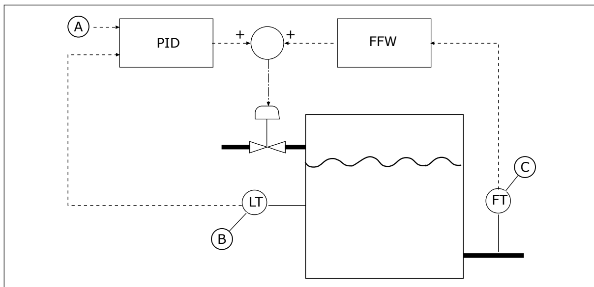
图 80: 前馈控制
