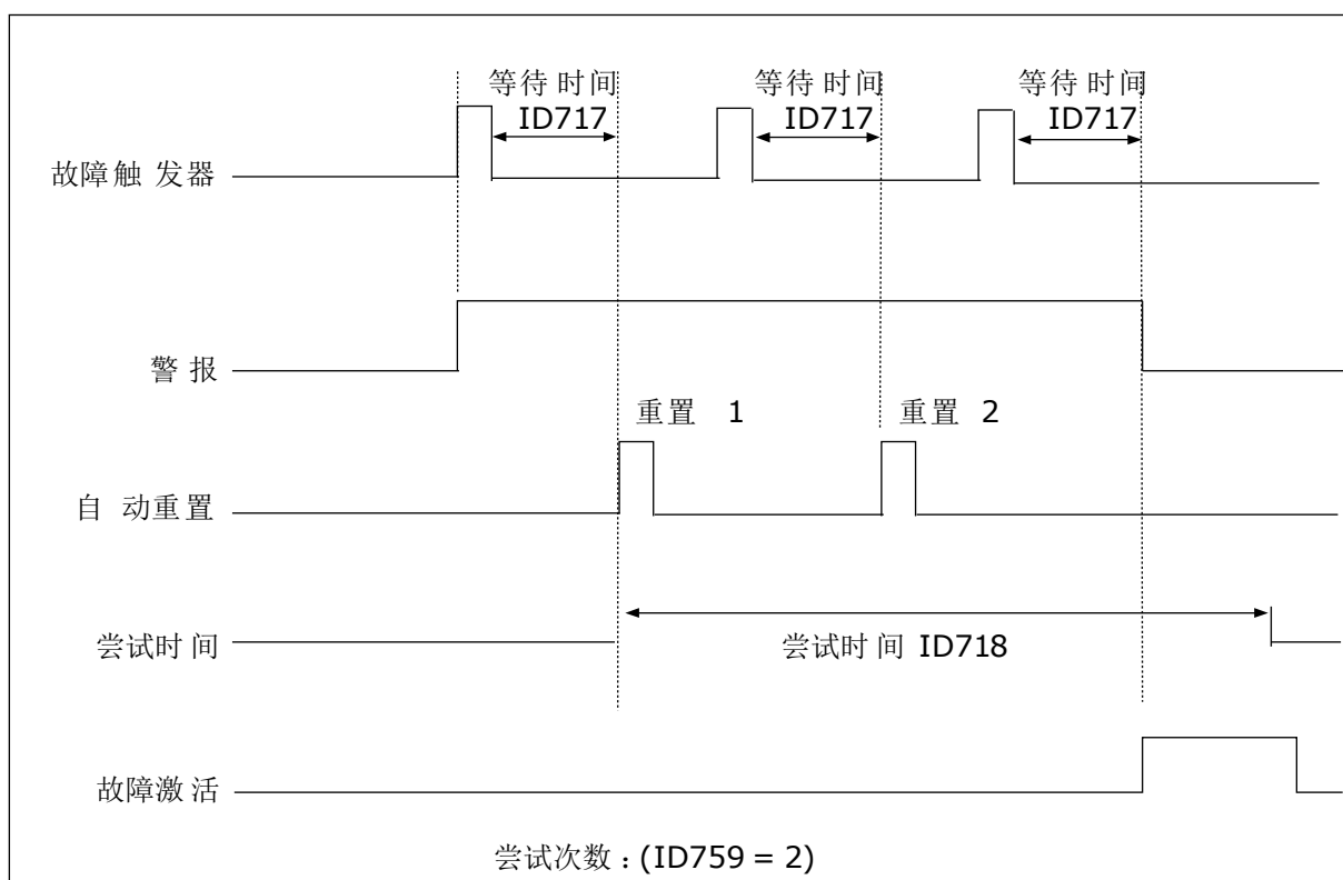
图 72: 自动重置功能
