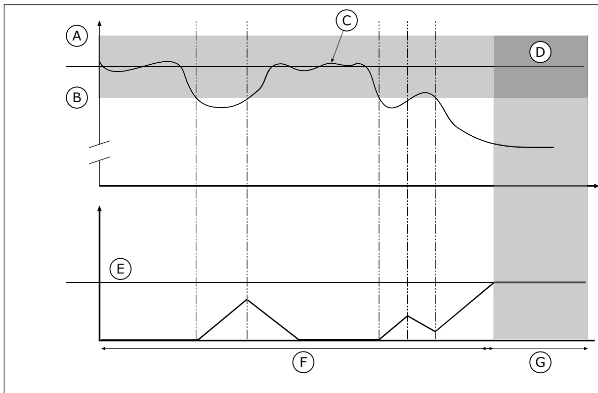
图 83: 反馈监控功能
