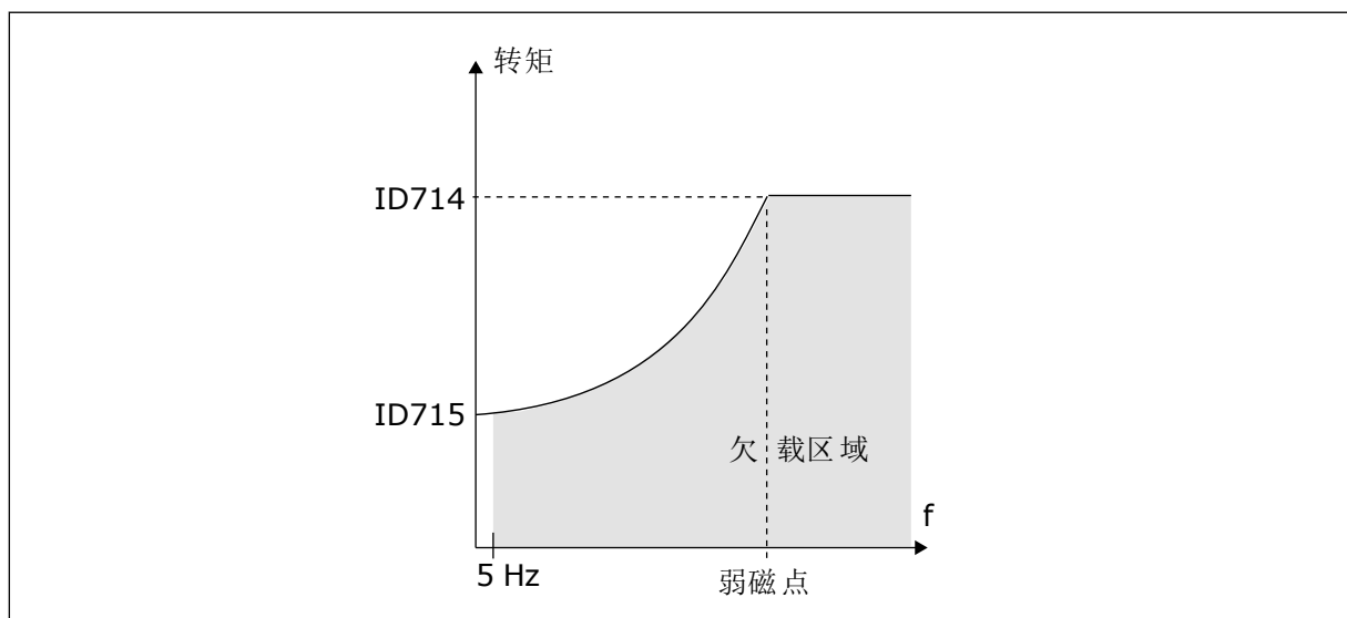
图 69: 设置最小负载
