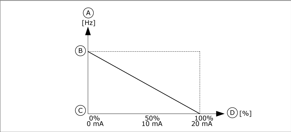
图 61: AI1 信号反演，选项 1
