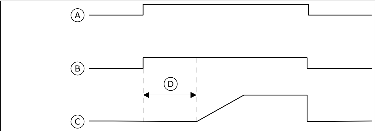
图 106: 注给泵功能
