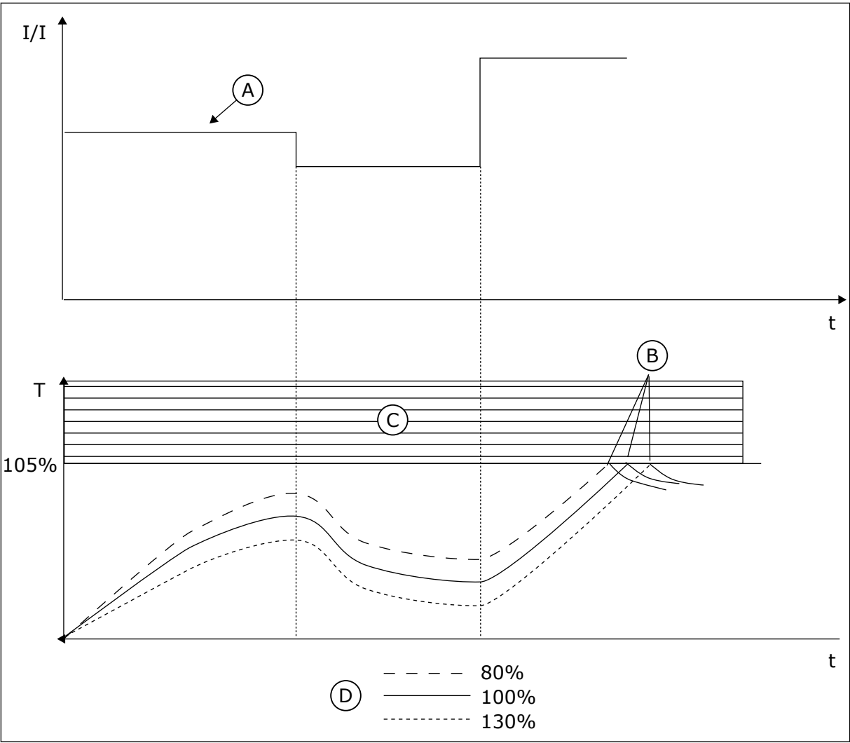
图 67: 电机温度的计算
