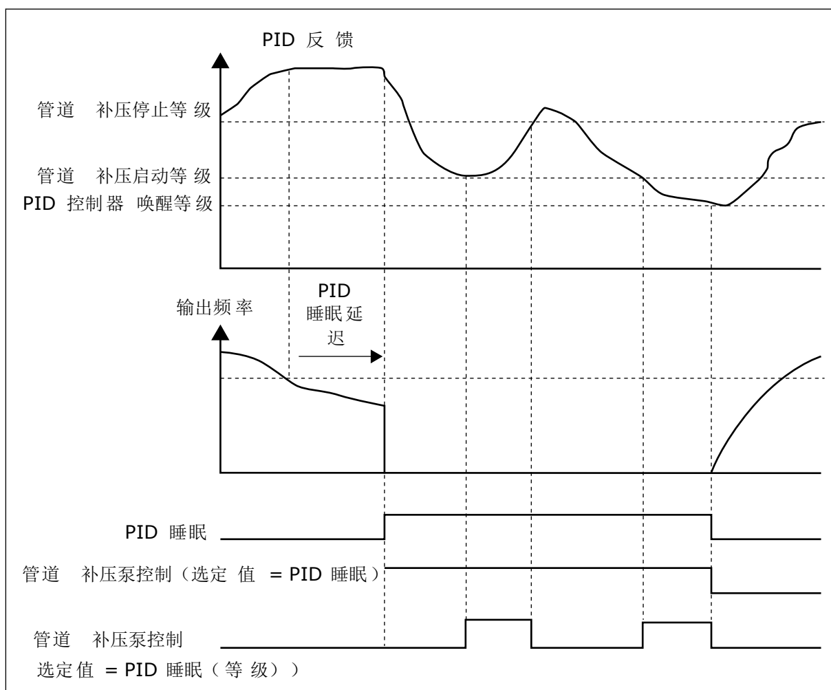
图 105: 管道补压泵功能
