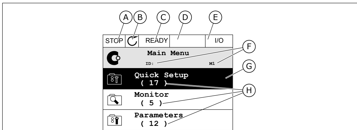
图 2: 图形显示屏
