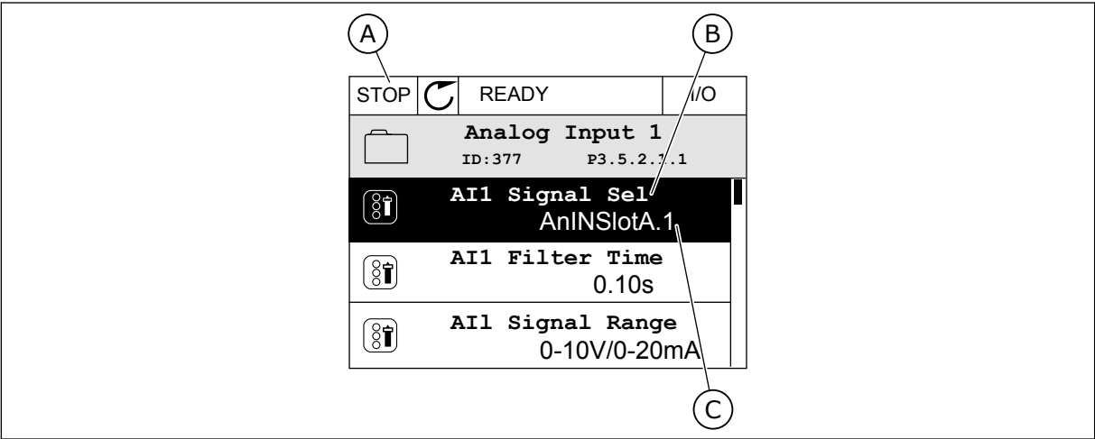
图 54: 图形显示屏中的“模拟输入”菜单
