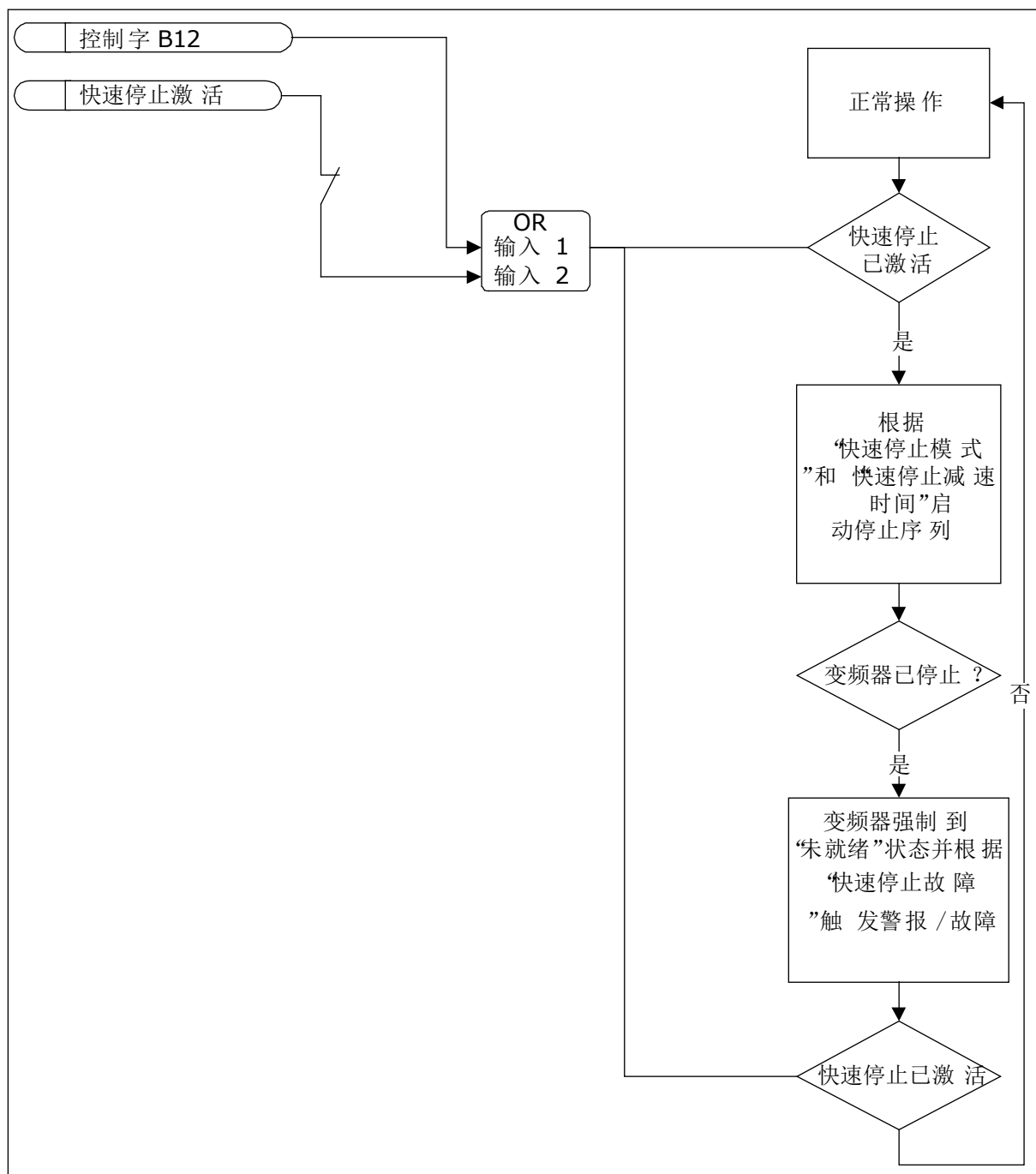
图 71: 快速停止逻辑
