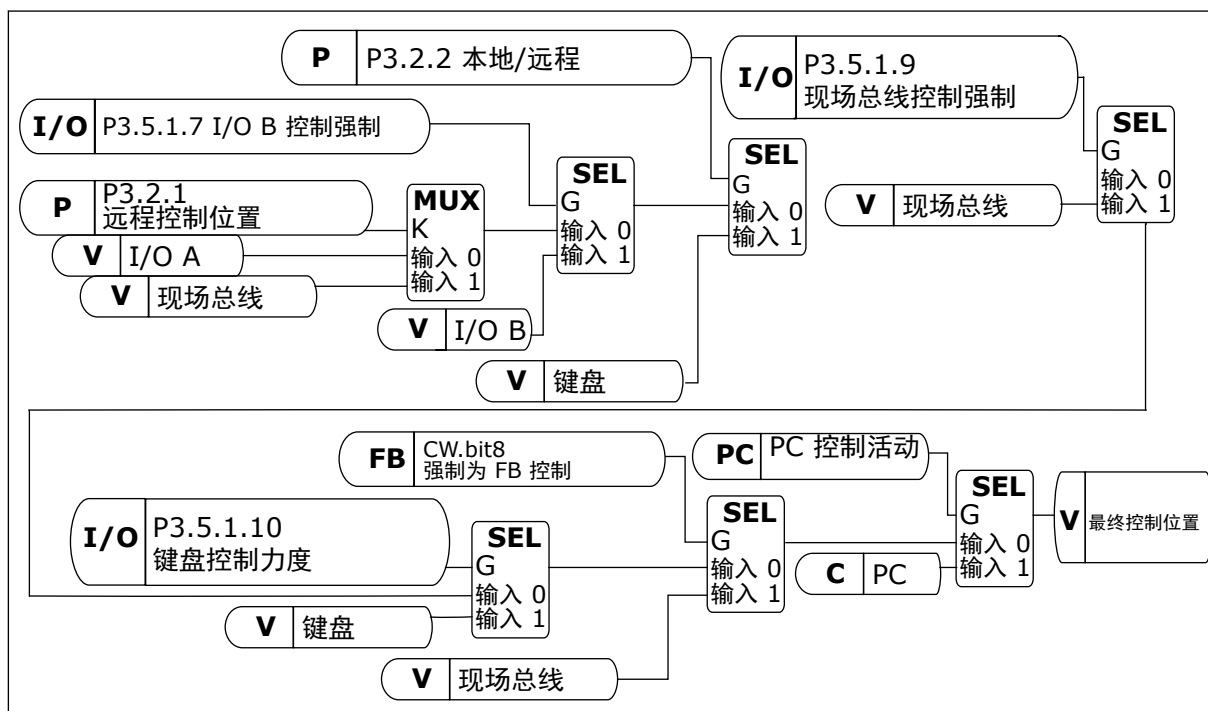
图 41: 控制位置
