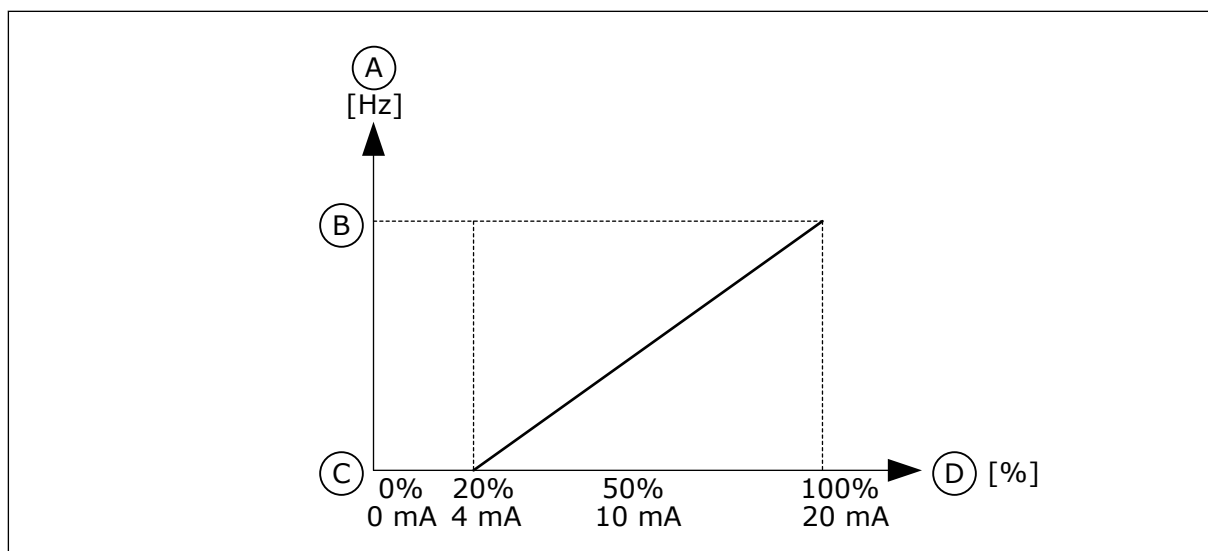
图 58: 模拟输入信号范围，选项 1
