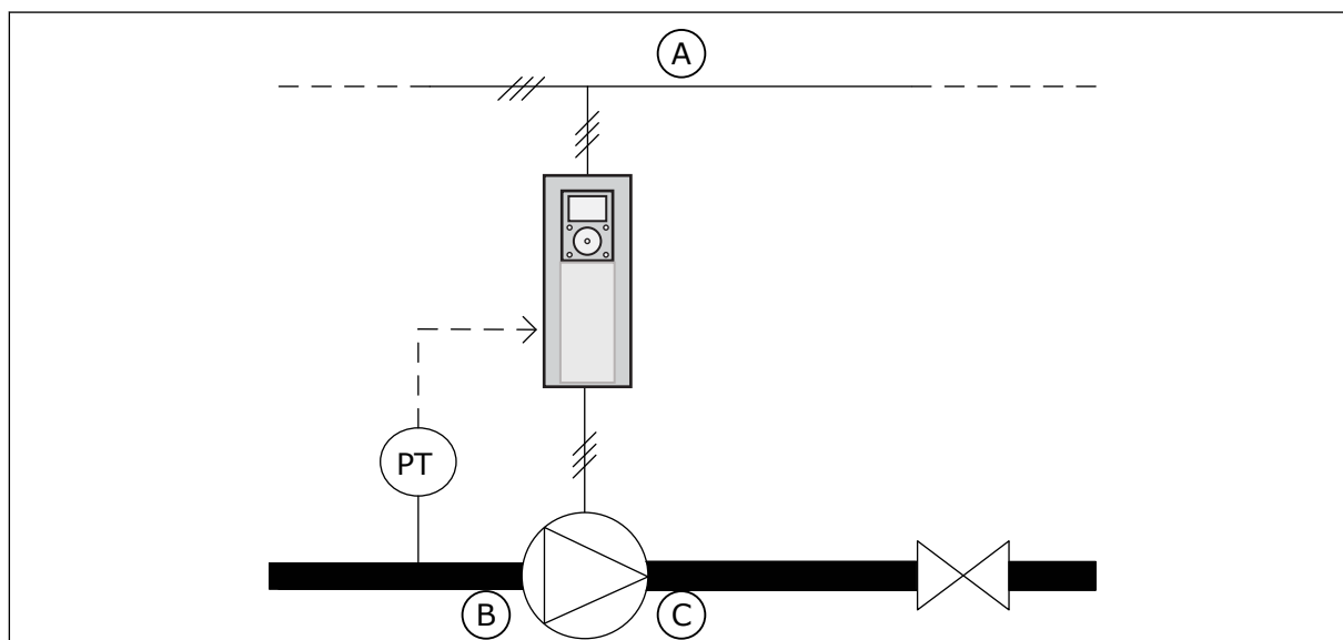
图 86: 压力传感器的位置
