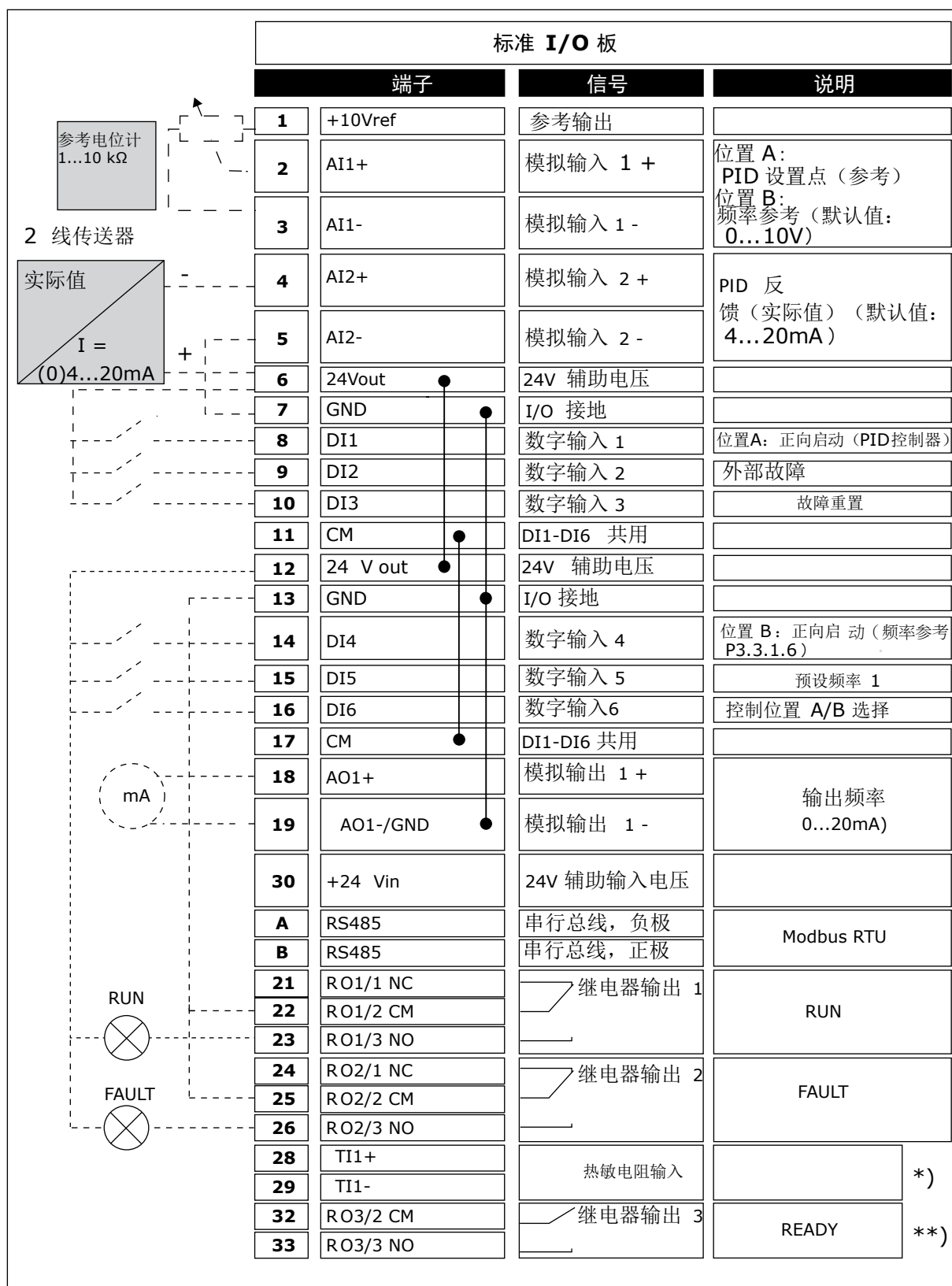
图 6: PID 控制应用程序的默认控制连接
