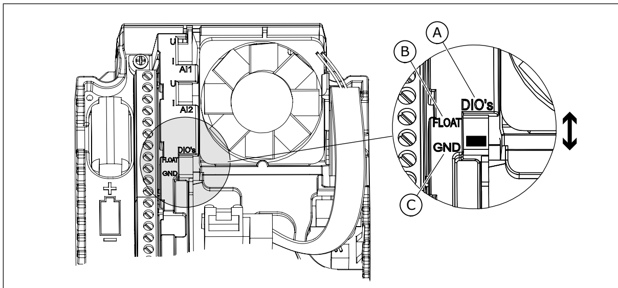
图 5: DIP 开关
