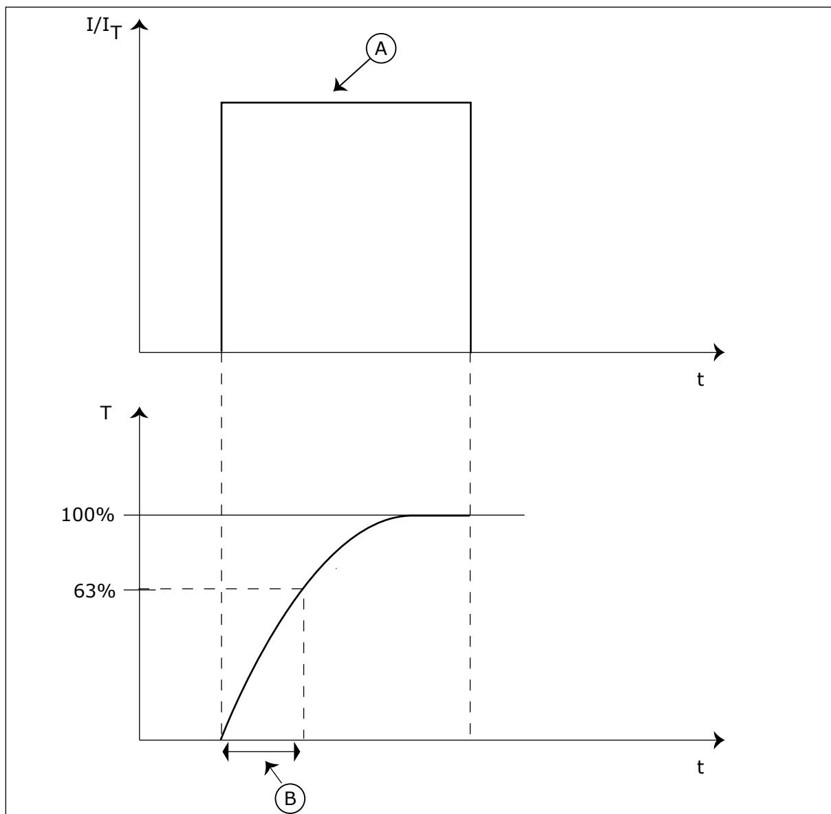
图 66: 电机热时间常数
