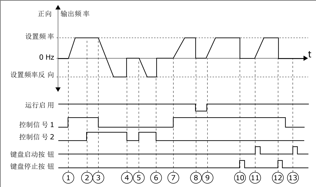
图 42: I/O A 启动/停止逻辑 = 0
