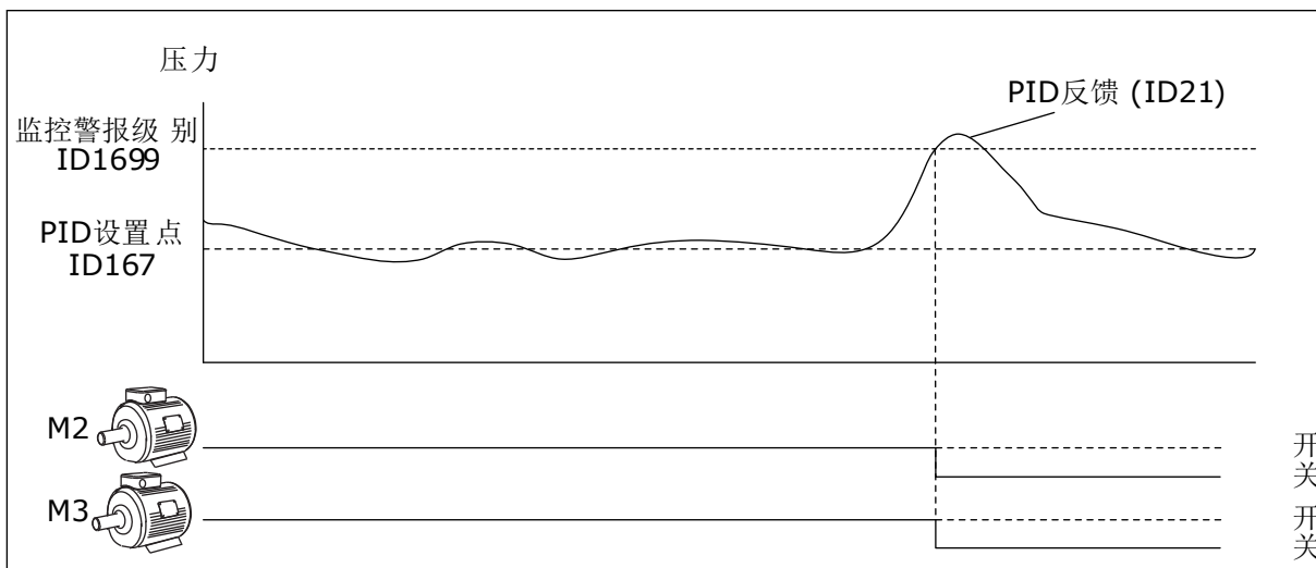
图 100: 过压监控功能
