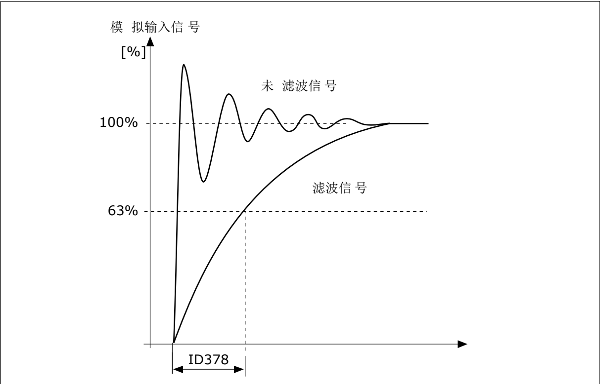
图 56: AI1 信号滤波
