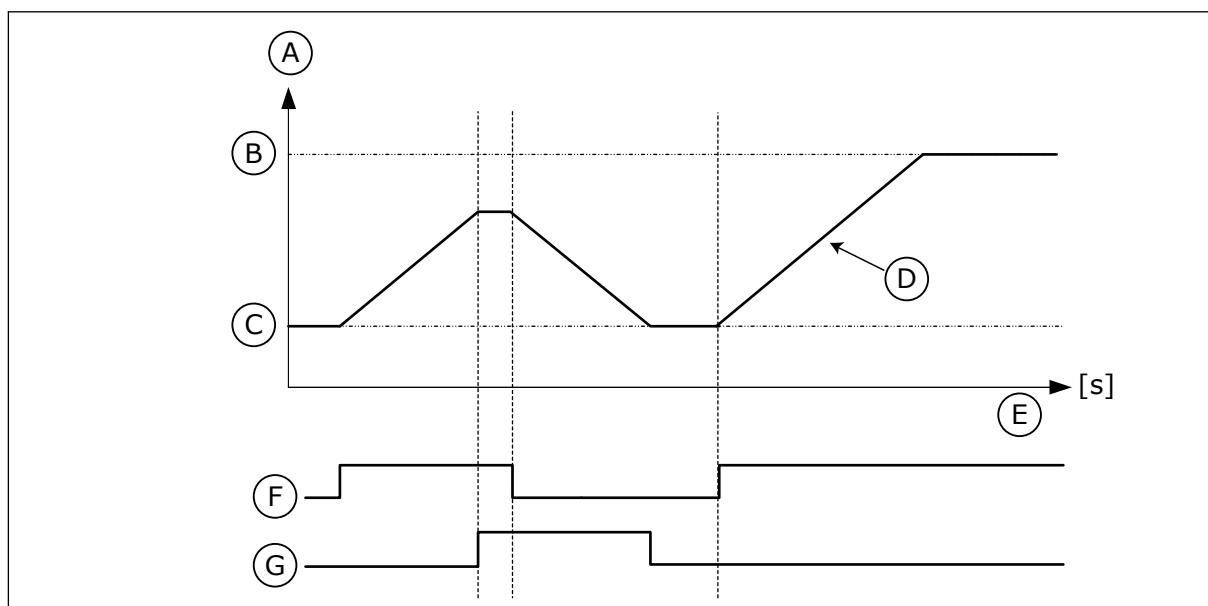
图 47: 电机电位计参数
