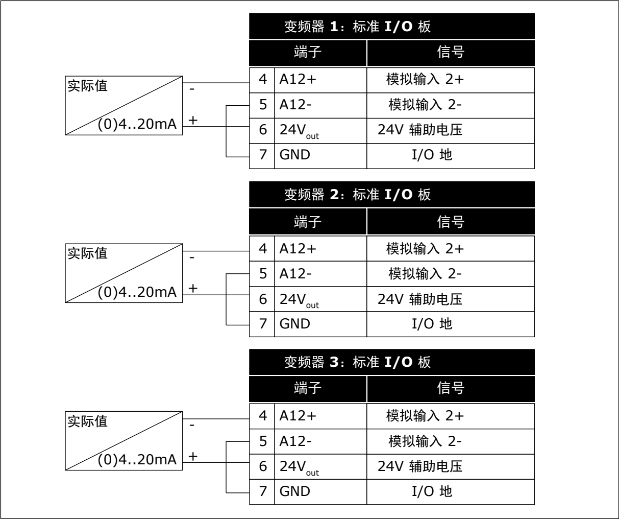
图 94: 每个变频器的反馈传感器的接线
