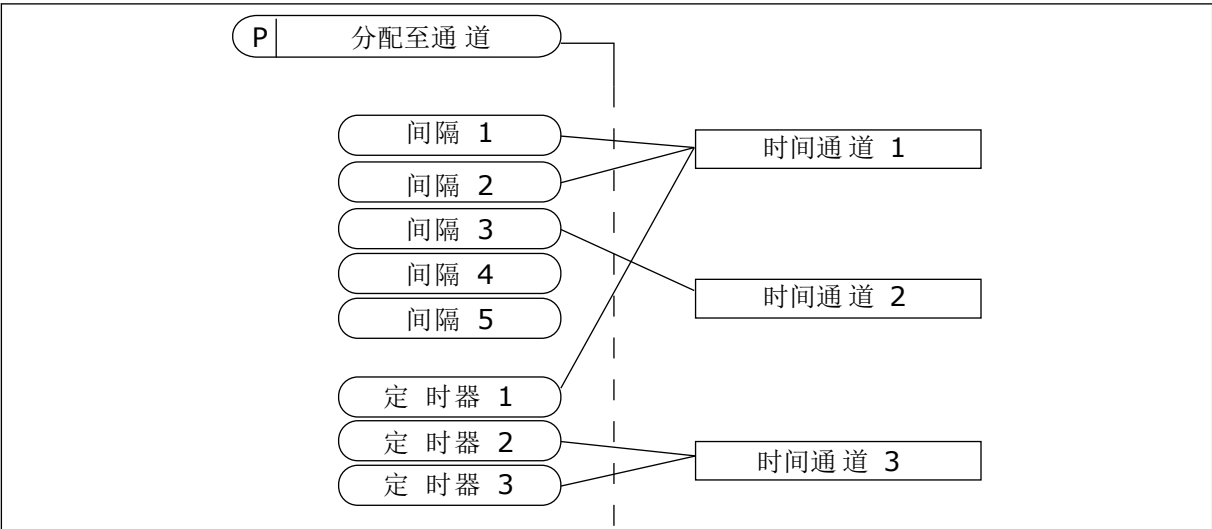
图 73: 将间隔和定时器分配至时间通道很灵活。每个间隔和定时器都有一个参数，可以使用此参数将其分配至某个时间通道。
