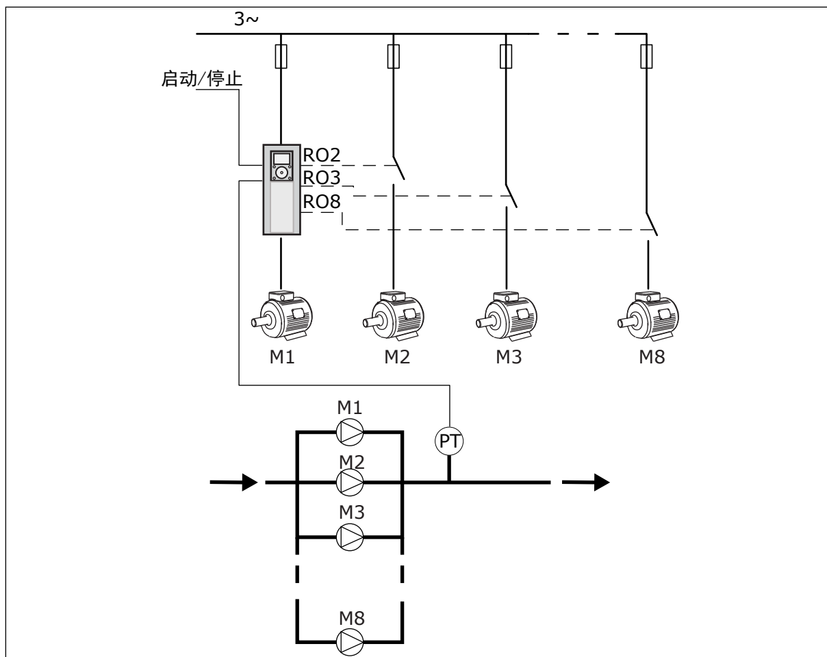
图 89: 单变频器配置 ( PT = 压力传感器 )
