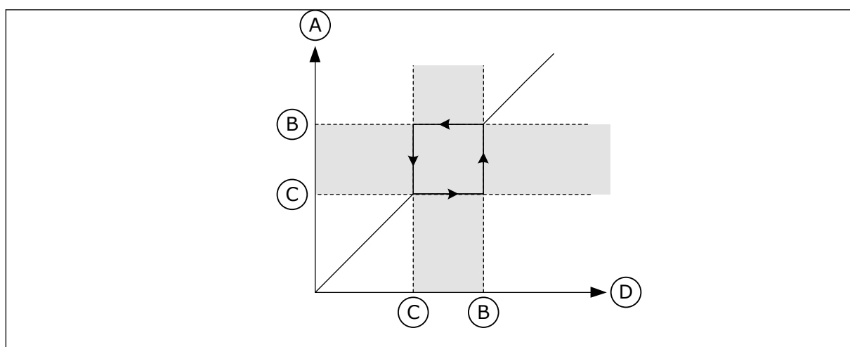
图 63: 禁止的频率
