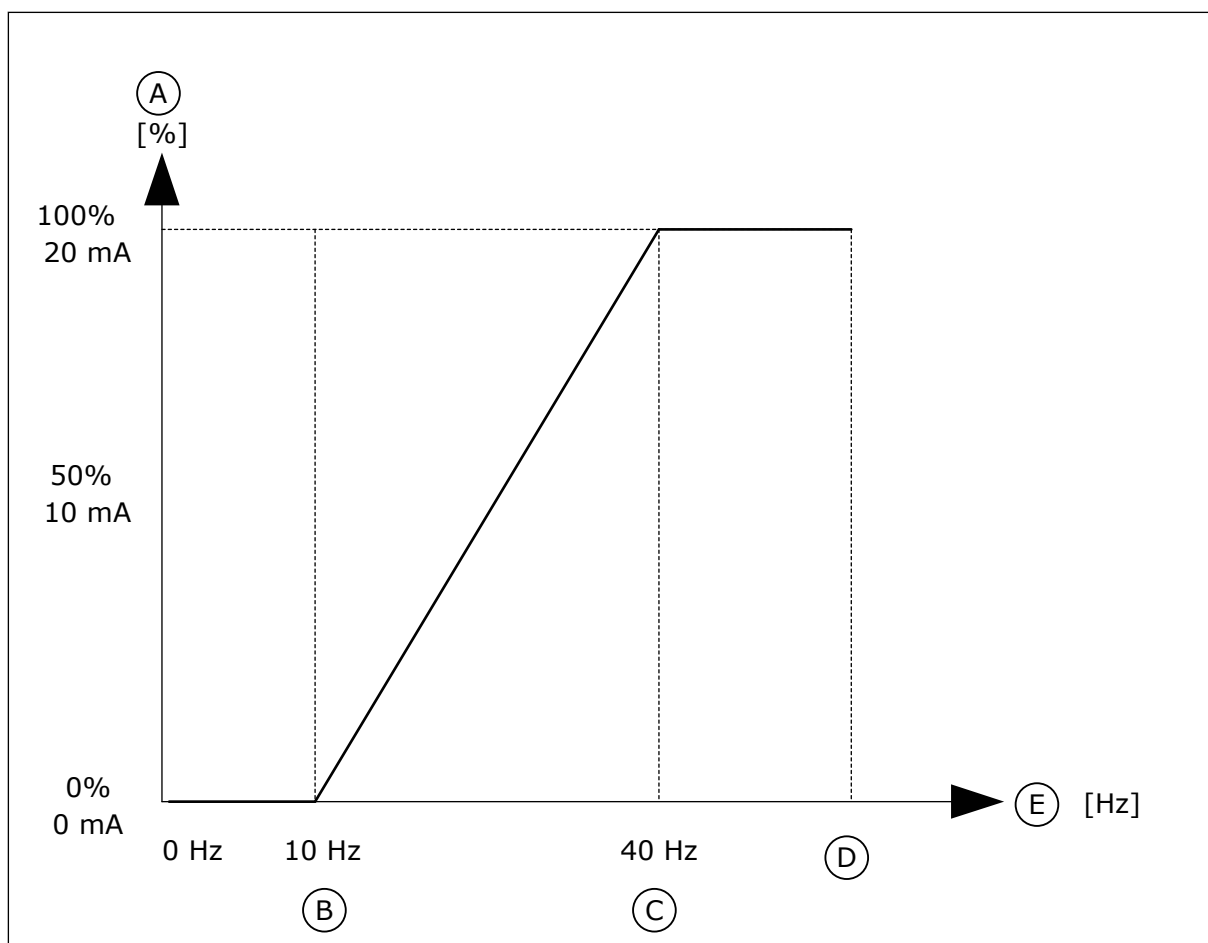
图 62: A01 信号的缩放
