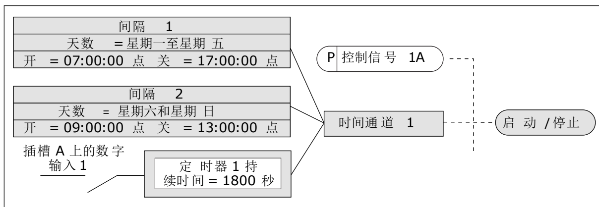
图 78: 时间通道 1 ( 而非数字输入 ) 用作启动命令的控制信号
