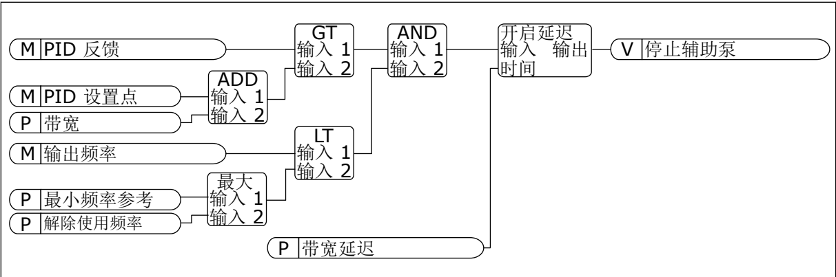
图 102: 降级频率
