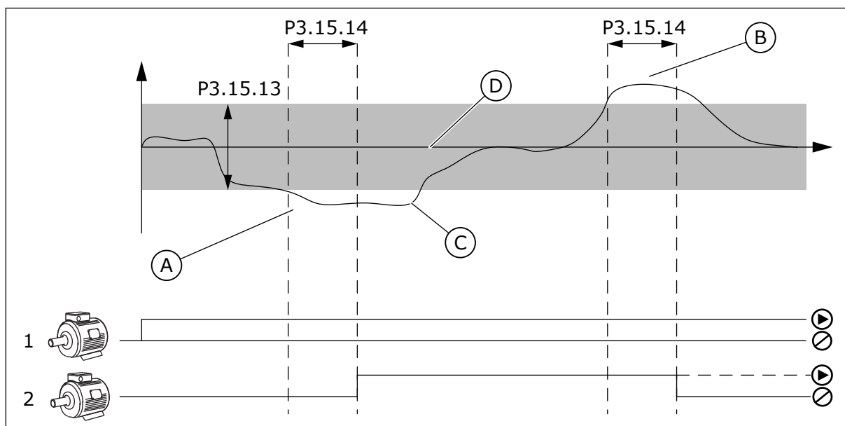
图 99: 辅助泵的启动/停止 ( P3.15.13 = 带宽 , P3.15.14 = 带宽延迟 )
