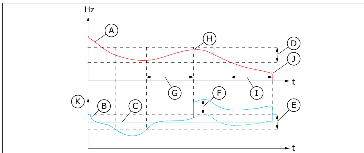
图 88: 睡眠，检测到无需求
