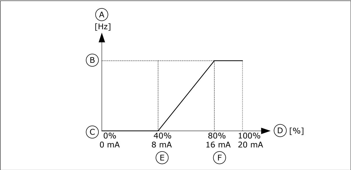
图 59: AI1 信号自定义最小值/最大值
