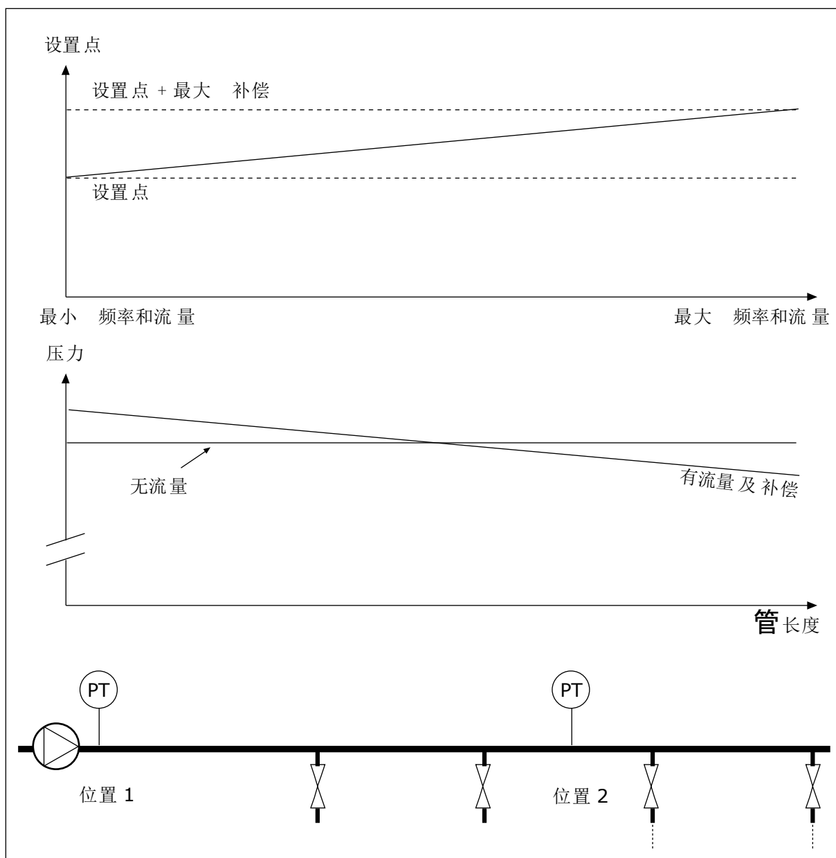
图 85: 压力损失补偿的启用设置点 1
