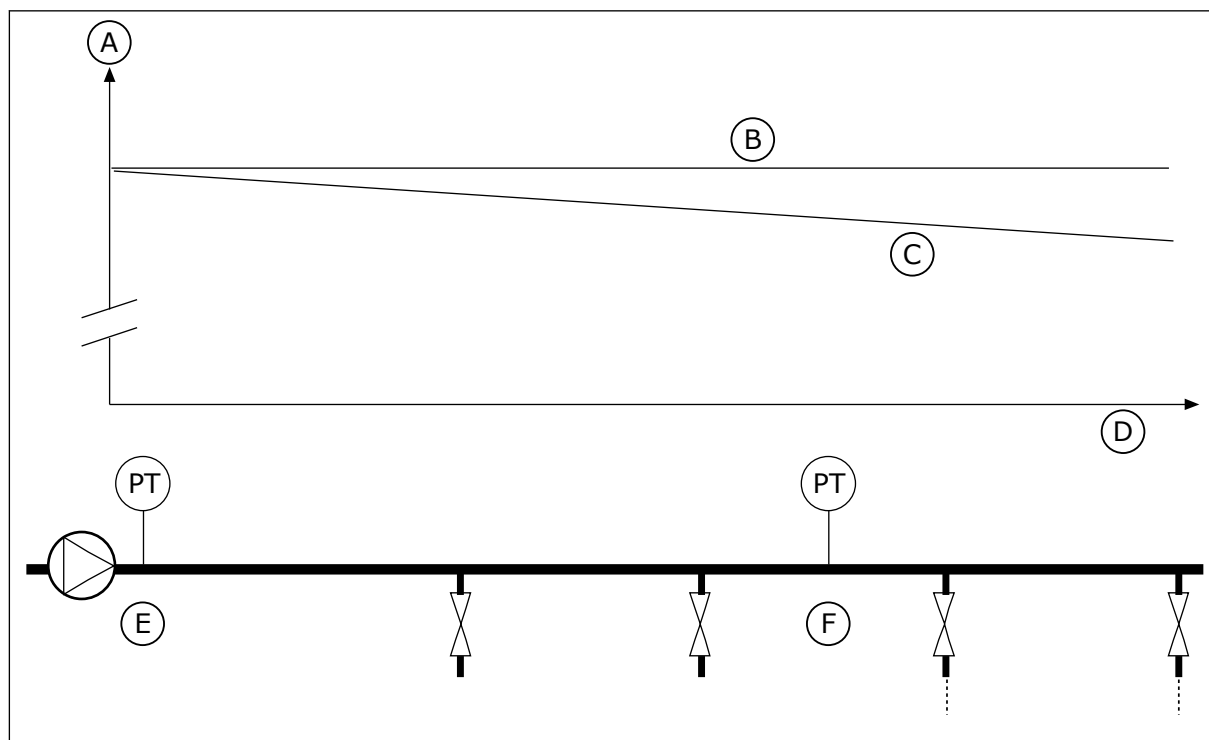
图 84: 压力传感器的位置
