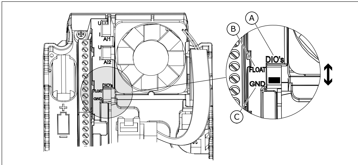
图 12: DIP 开关
