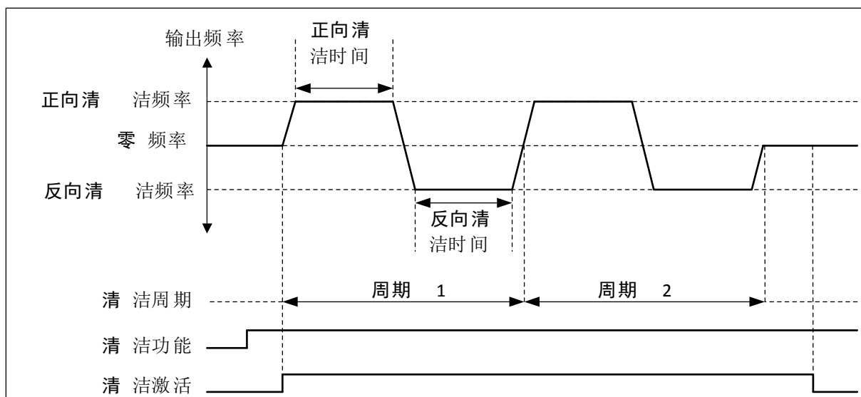
图 104: 自动清洁功能
