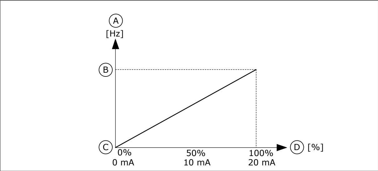
图 60: AI1 信号反演，选项 0
