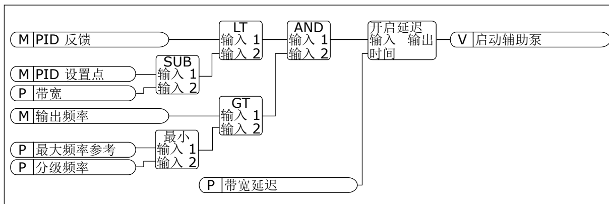
图 101: 分级频率
