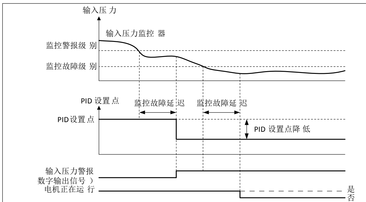
图 87: 输入压力监控功能
