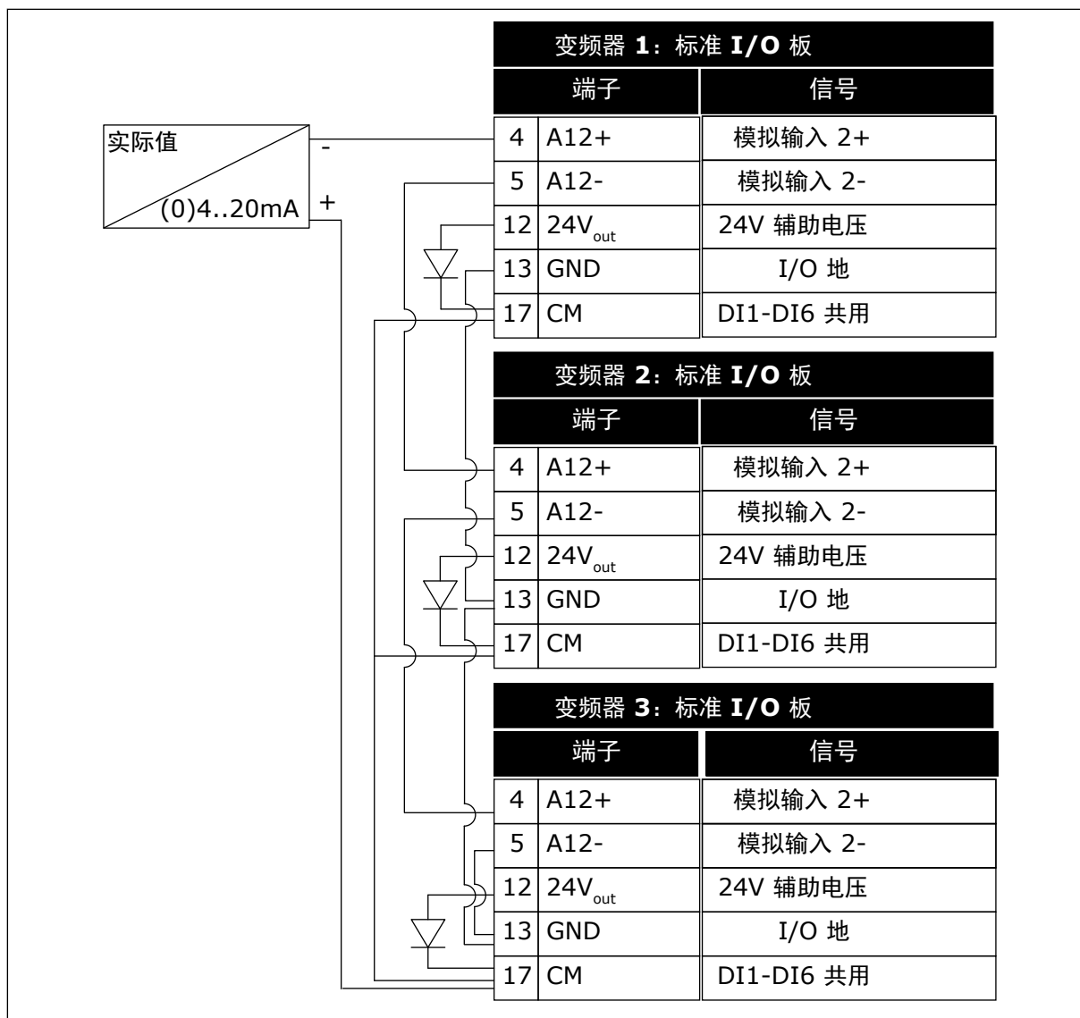
图 95: 所有变频器的相同传感器的接线 ( 从变频器的 I/O 板供电 )
