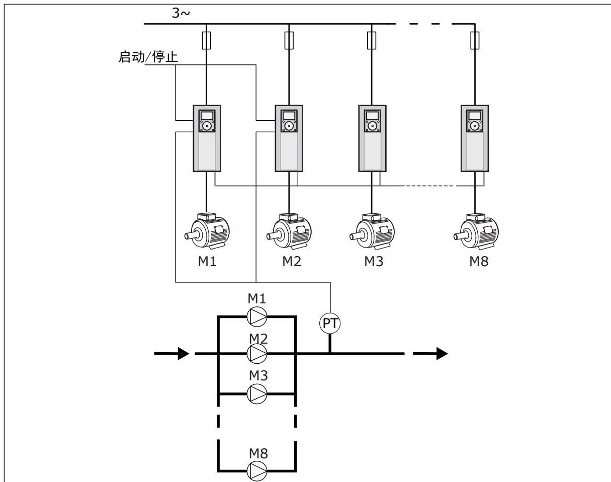
图 90: 多变频器配置 (PT = 压力传感器)
