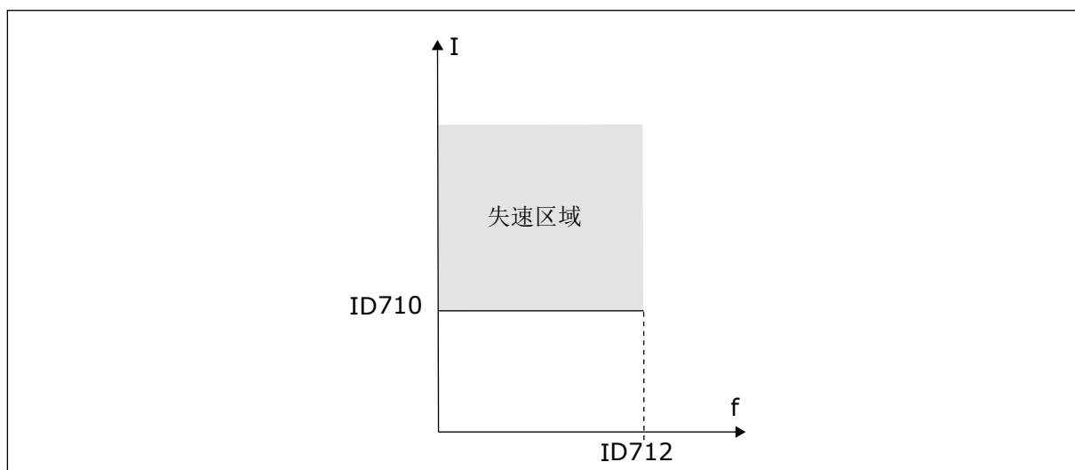
图 68: 失速特征设置
