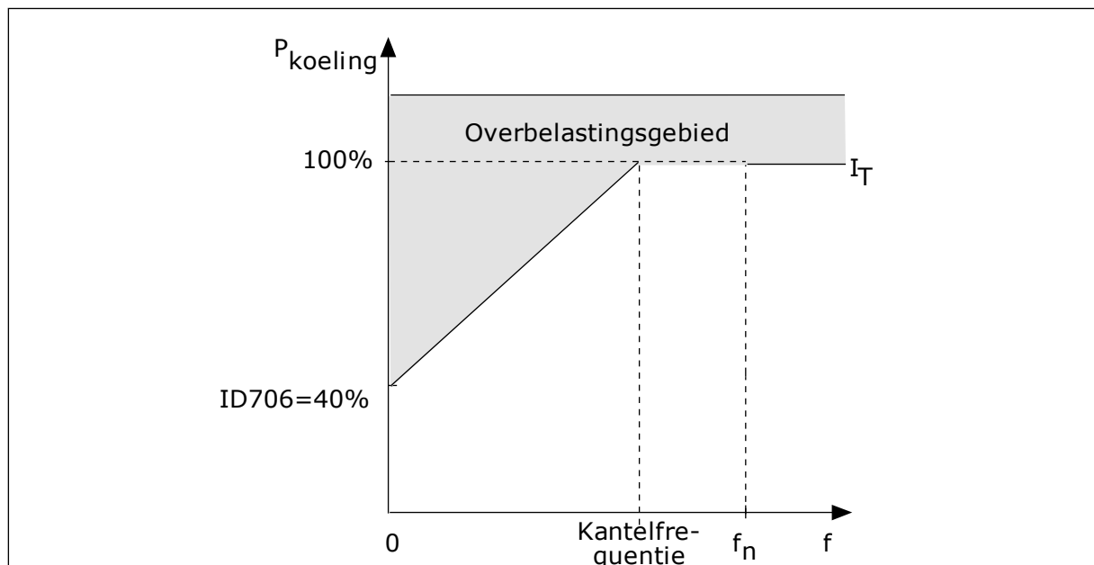
Afb. 72: De motor thermische stroom I_T -curve
