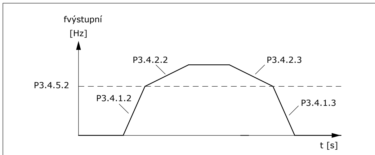
Obr. 50: Rampa 2 se aktivuje tehdy, jestliže výstupní frekvence překročí prahovou úroveň. (P. 3.4.5.2 = Prahová frekvence rampy, P3.4.1.2 = Doba rozběhu 1, P3.4.2.2 = Doba rozběhu 2, P3.4.1.3 = Doba doběhu 1, P3.4.2.3 = Doba doběhu 2)
