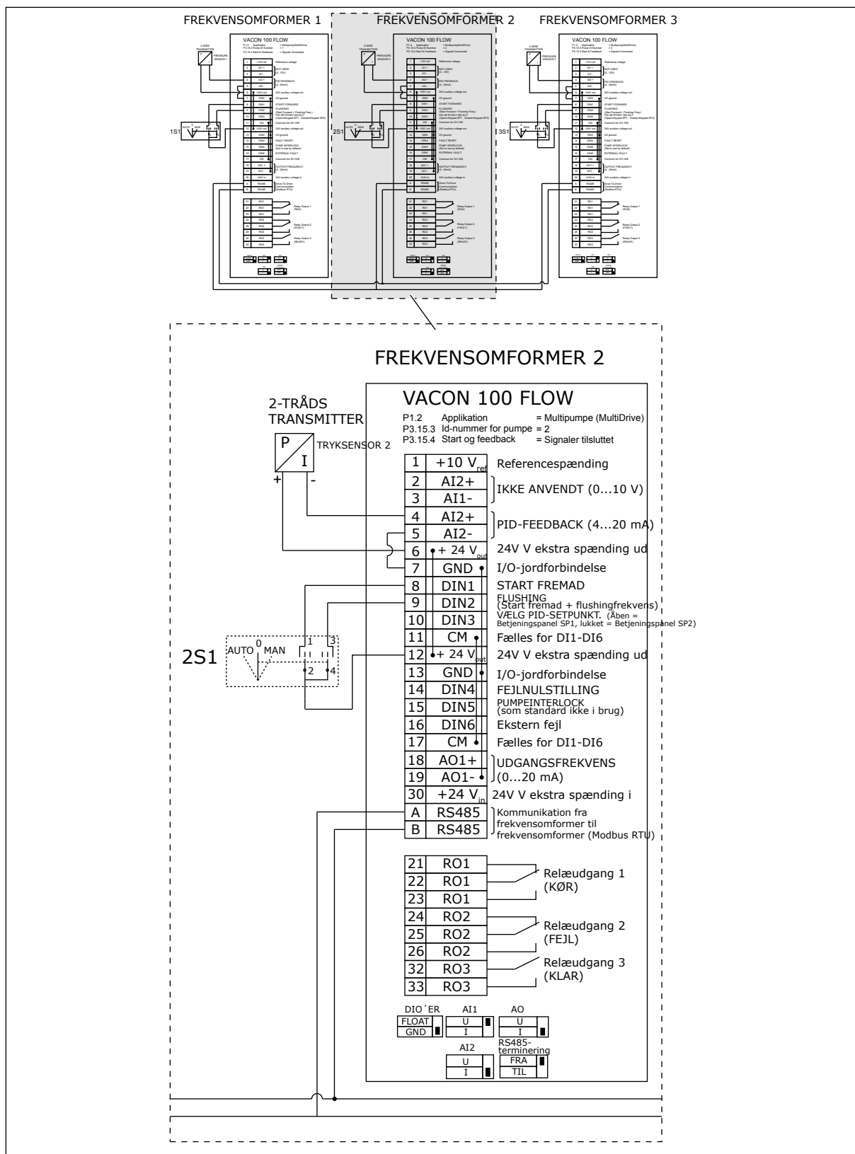
Fig. 19: Eldiagram til multipumpesystem (flere frekvensomformere), eksempel 1B
