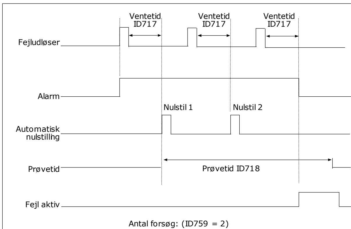
Fig. 72: Automatisk nulstillingsfunktion
