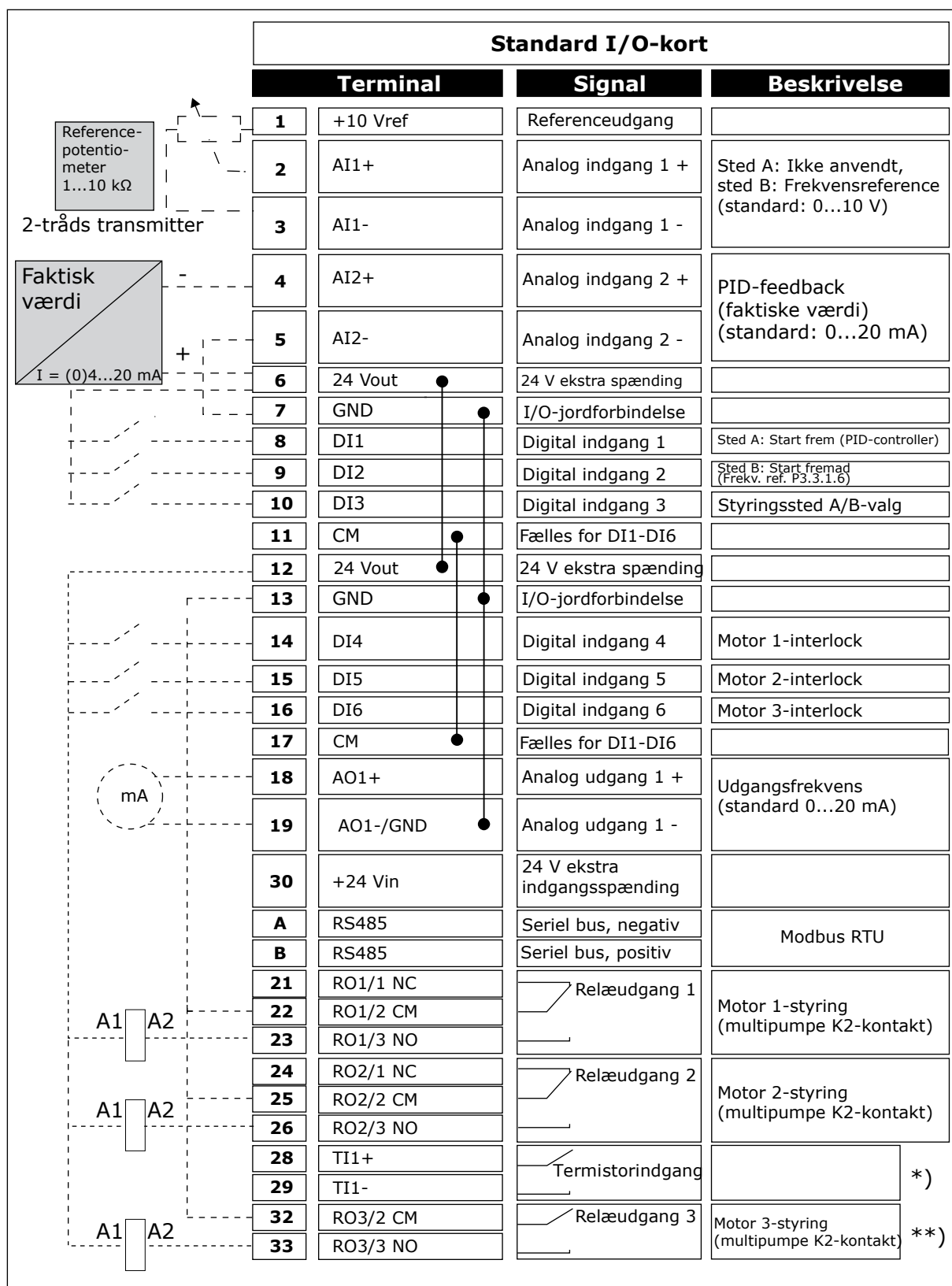
Fig. 11: Standardkontrolforbindelser til multipumpeapplikation (enkelt frekvensomformer)
