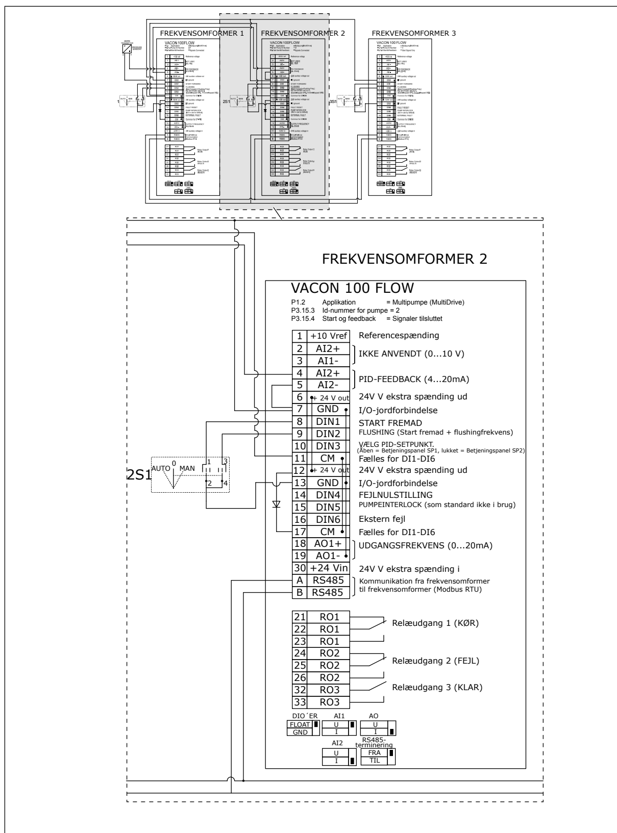
Fig. 28: Eldiagram til multipumpesystem (flere frekvensomformere), eksempel 4B
