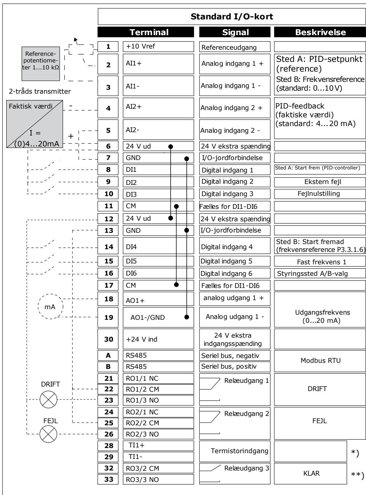
Fig. 6: Standardstyringsforbindelser for PID-styringsapplikationen
