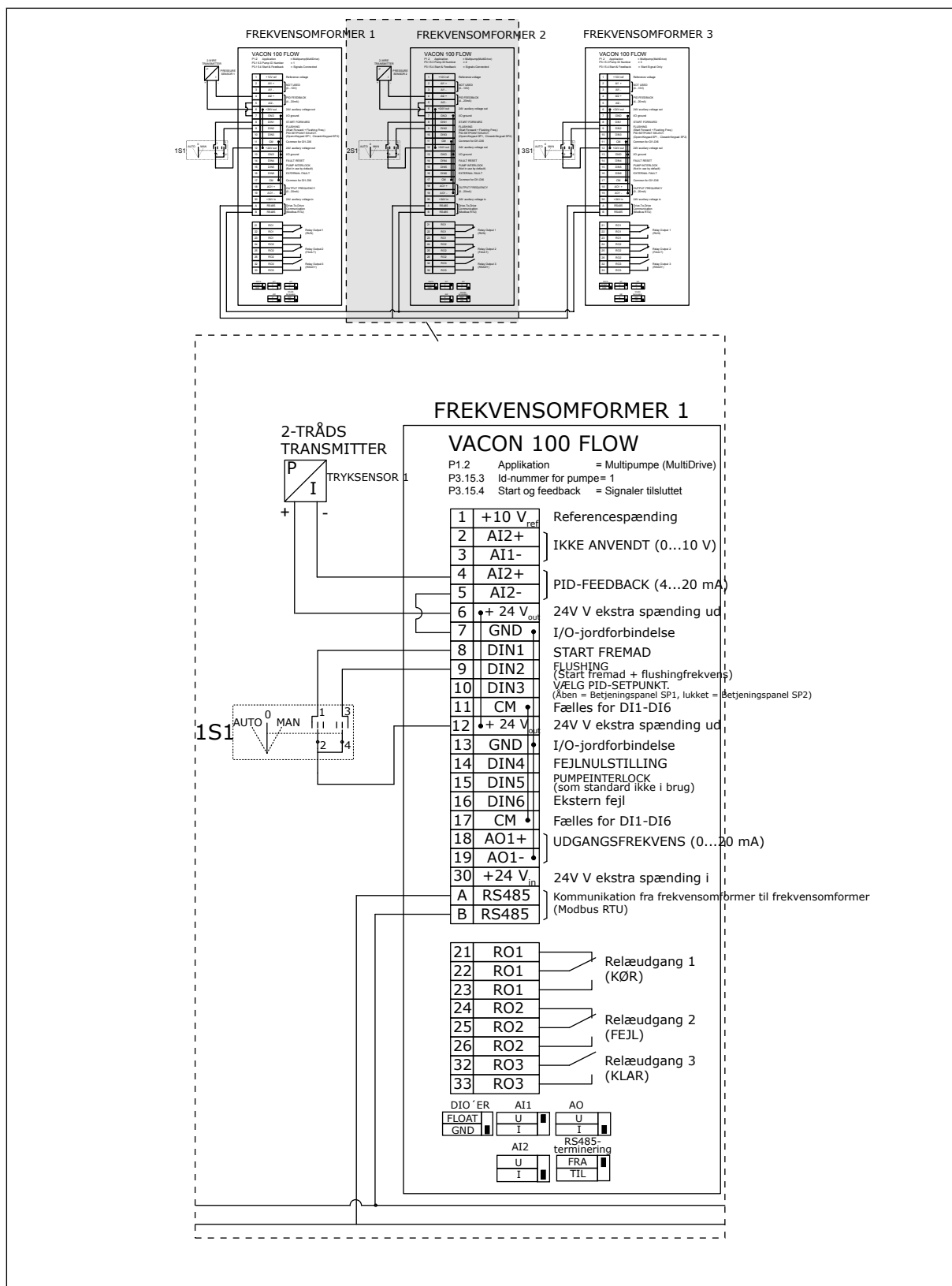
Fig. 25: Eldiagram til multipumpesystem (flere frekvensomformere), eksempel 3B
