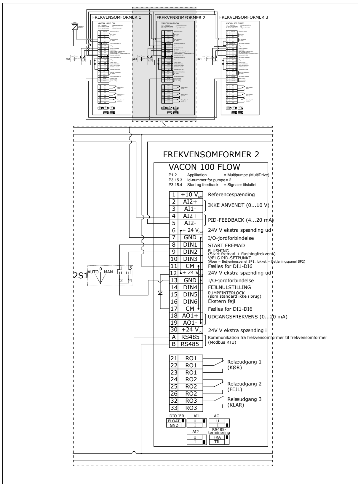
Fig. 22: Eldiagram til multipumpesystem (flere frekvensomformere), eksempel 2B
