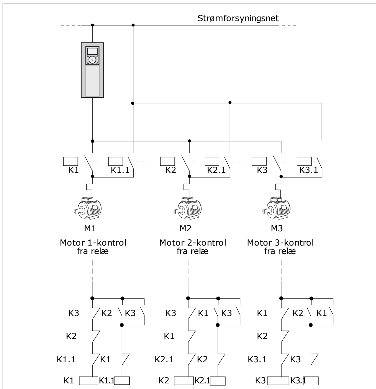
Fig. 98: Valg 1
