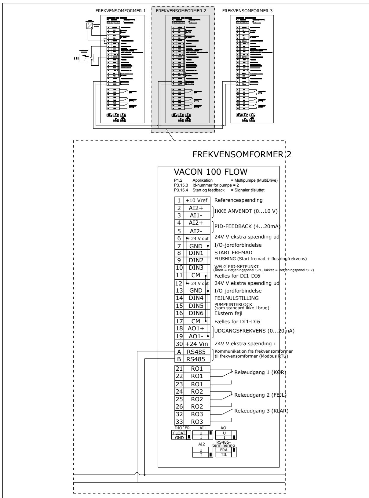
Fig. 31: Eldiagram til multipumpesystem (flere frekvensomformere), eksempel 5B
