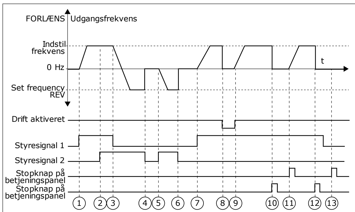
Fig. 42: I/O A-start/stop-logik = 0
