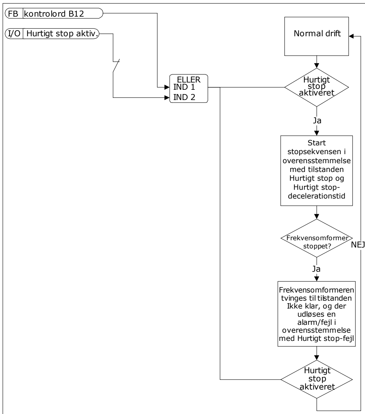
Fig. 71: Hurtigt stop-tilstand
