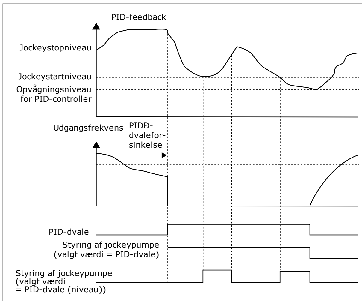
Fig. 105: Jockeypumpefunktionen
