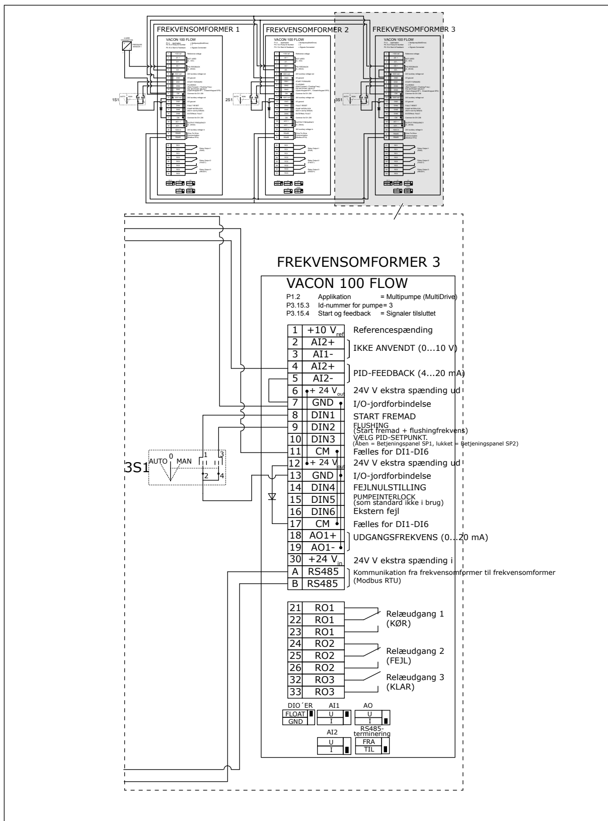
Fig. 23: Eldiagram til multipumpesystem (flere frekvensomformere), eksempel 2C
