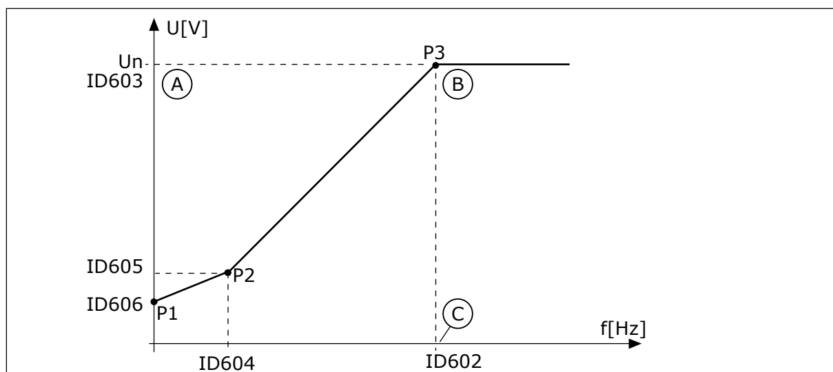
Fig. 39: Programmerbar U/f-kurve
