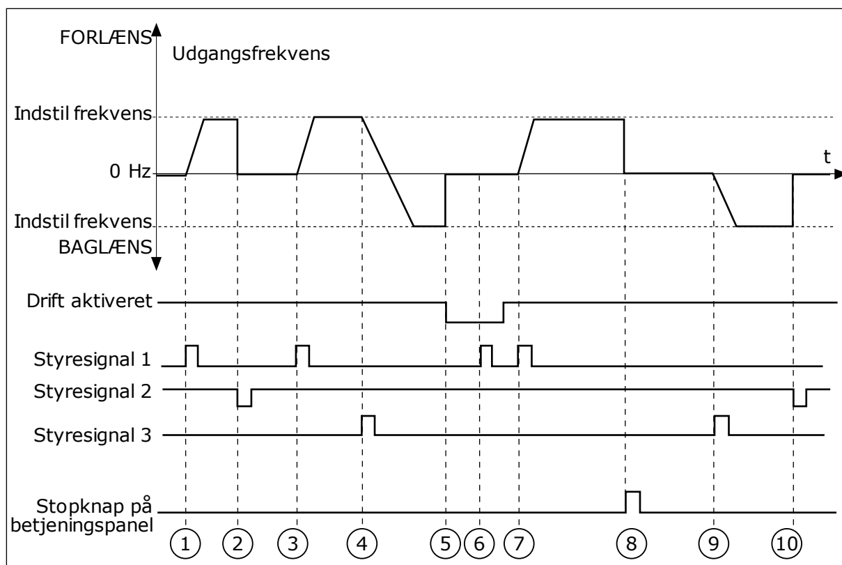
Fig. 43: I/O A-start/stop-logik = 1
