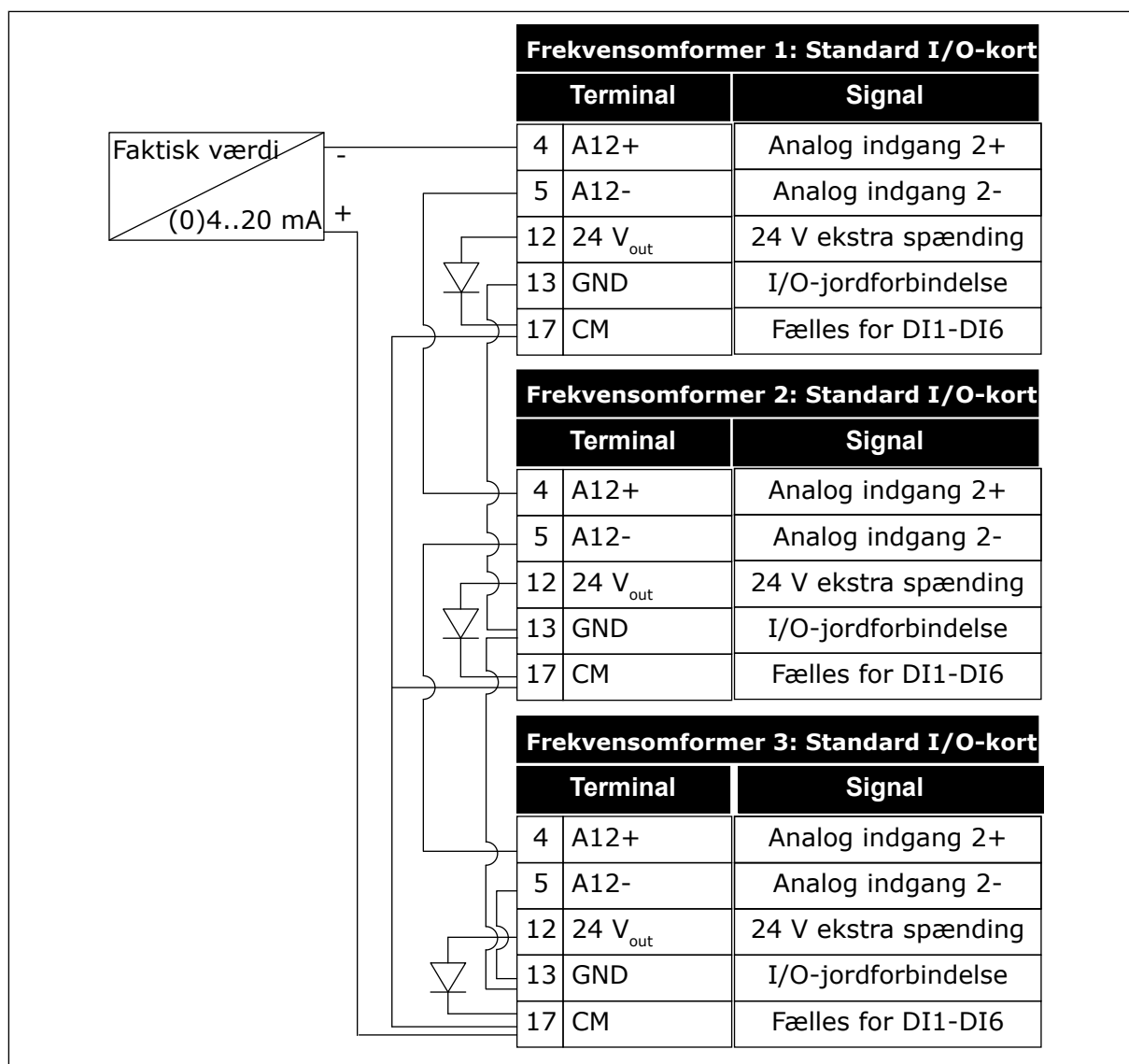
Fig. 95: Kabling af den samme sensor for alle frekvensomformere (tilvejebringes fra frekvensomformerens I/O-kort)
