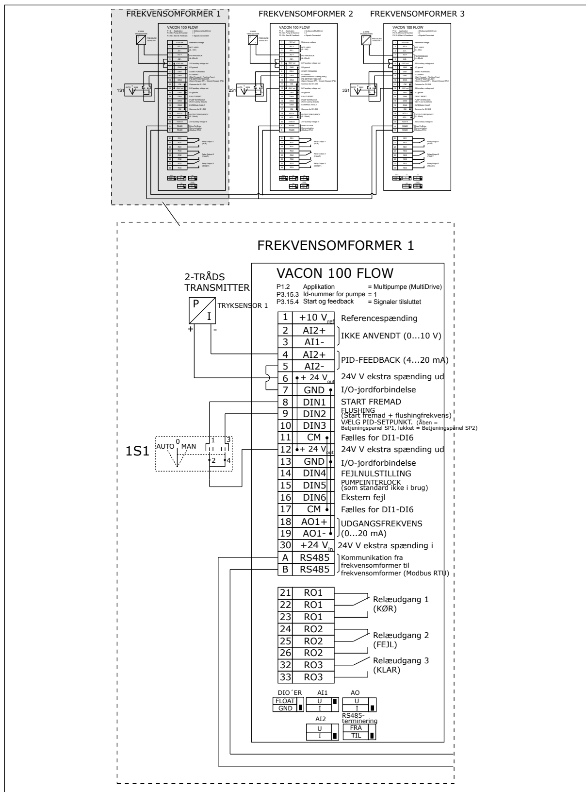
Fig. 18: Eldiagram til multipumpesystem (flere frekvensomformere), eksempel 1A
