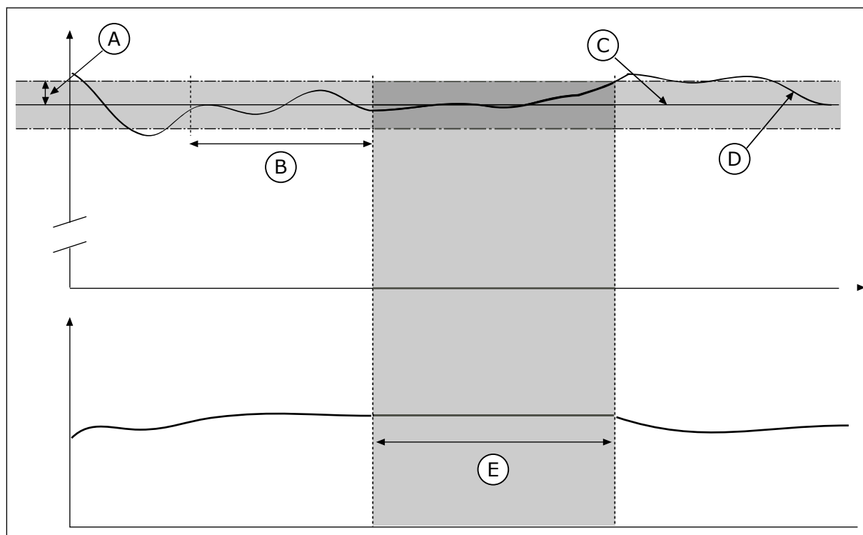
Fig. 79: Dødzonefunktion
