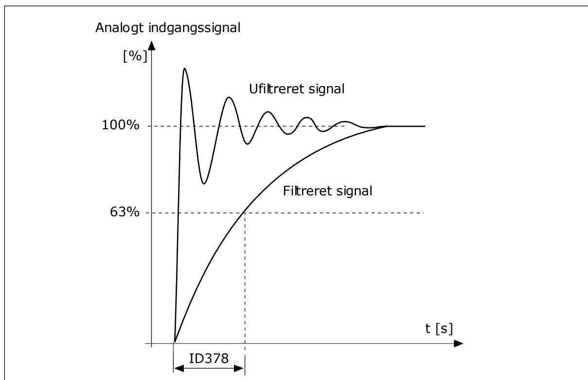
Fig. 56: AI1-signalfiltrering
