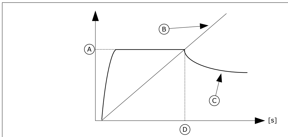
Fig. 40: I/f-startparametrene
