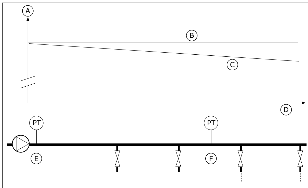
Fig. 84: Tryksensorens position
