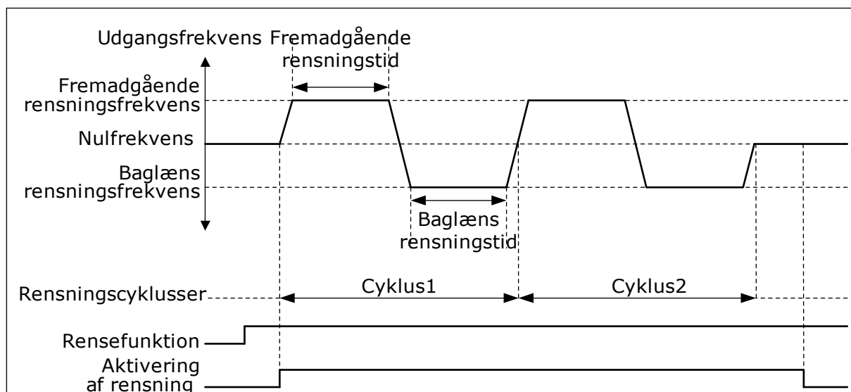
Fig. 104: Autorensningsfunktionen
