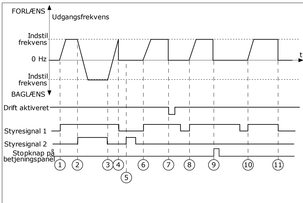
Fig. 46: I/O A-start/stop-logik = 4
