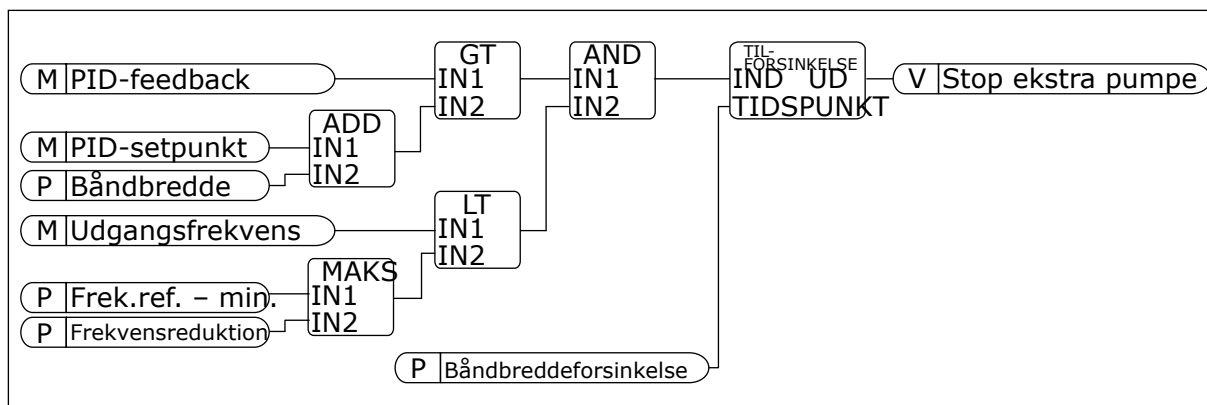
Fig. 102: Frekvensreduktion
