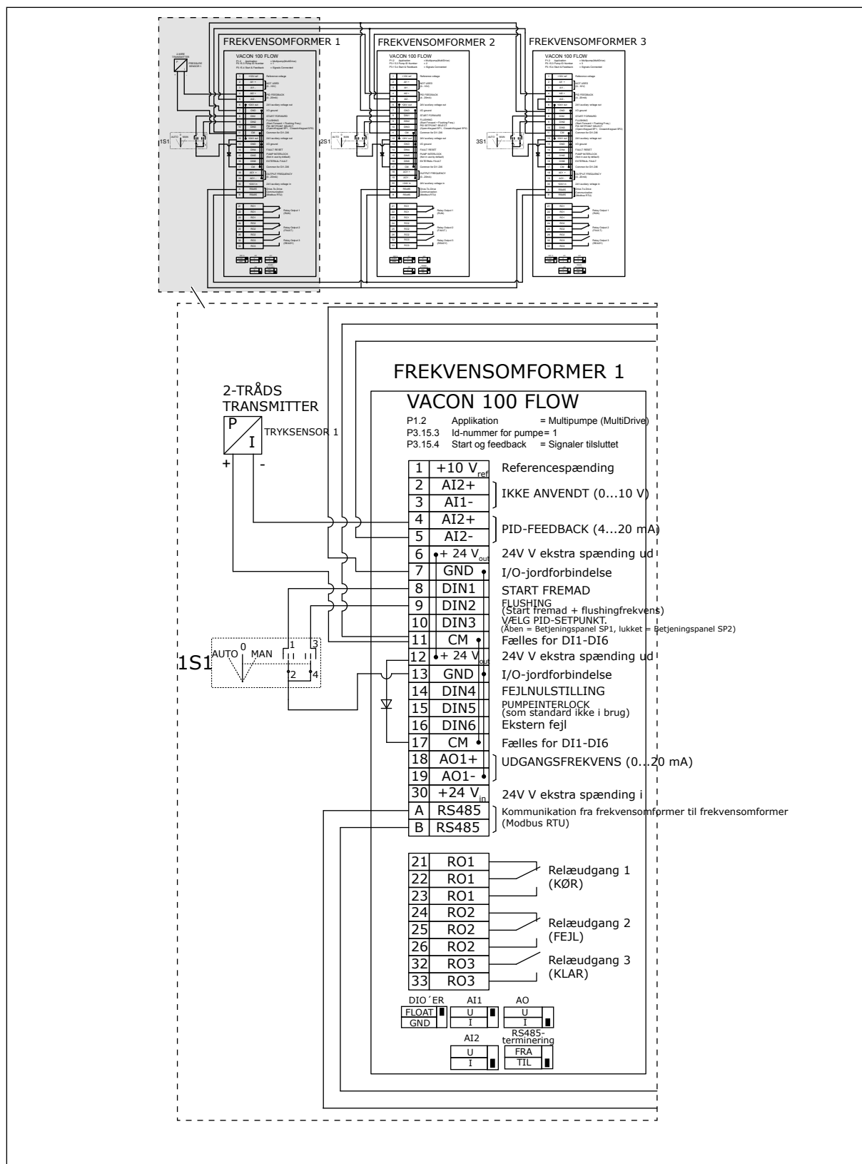
Fig. 21: Eldiagram til multipumpesystem (flere frekvensomformere), eksempel 2A
