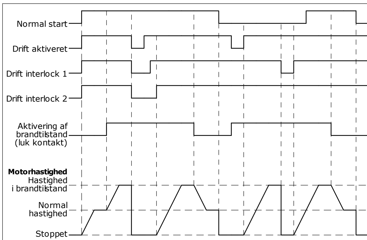
Fig. 103: Brandtilstandsfunktionen
