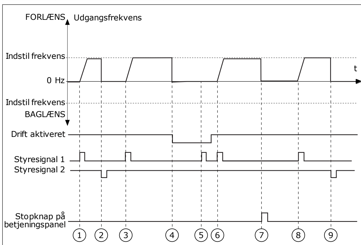
Fig. 16: I/O A-start/stop-logik = 1
