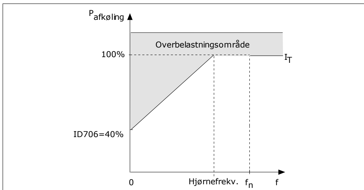
Fig. 28: Kurve for motorvarmestrom I_T
