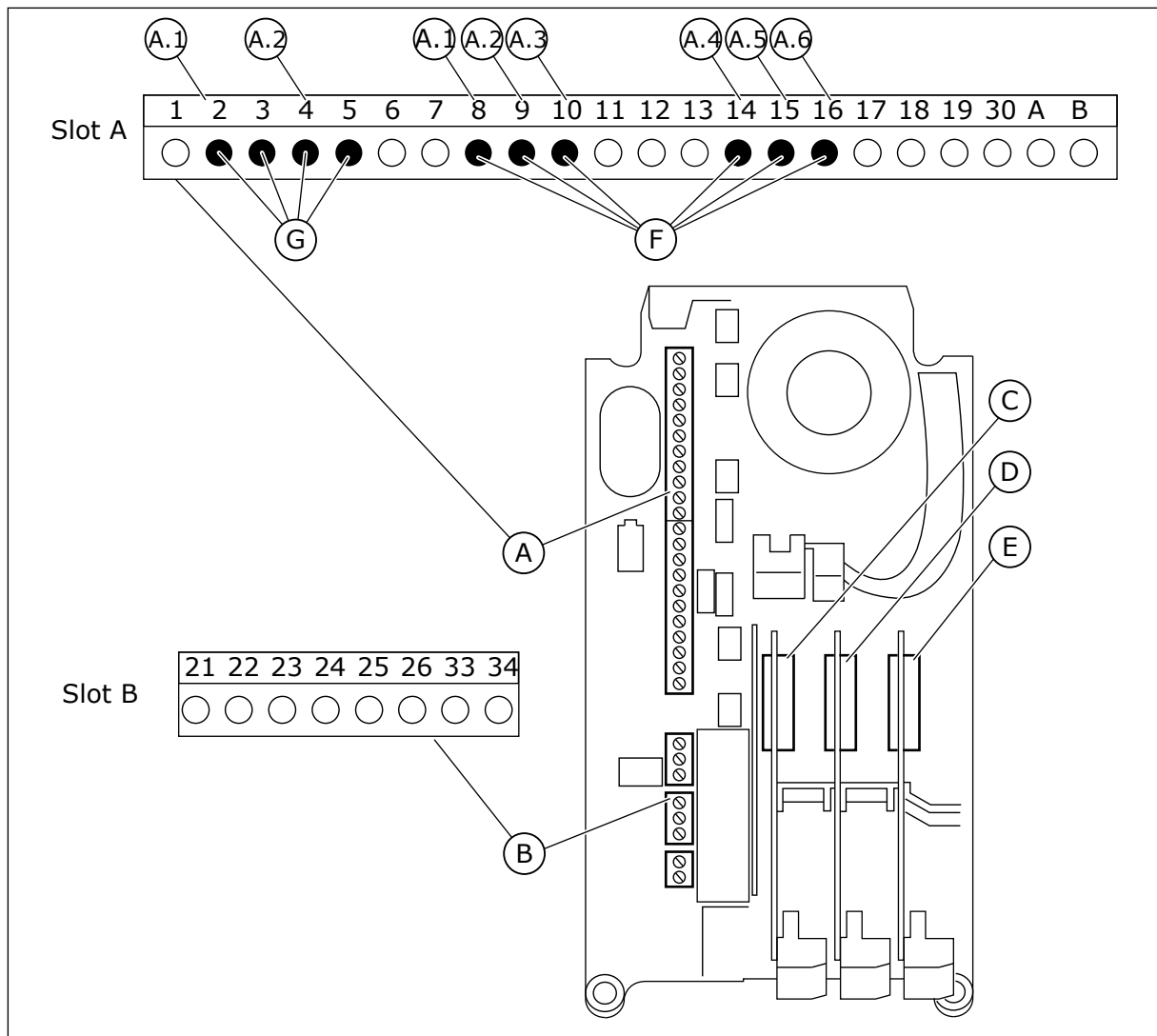
Σχ. 22: Οι υποδοχές προαιρετικής κάρτας και οι προγραμματιζόμενες εισοδοί
