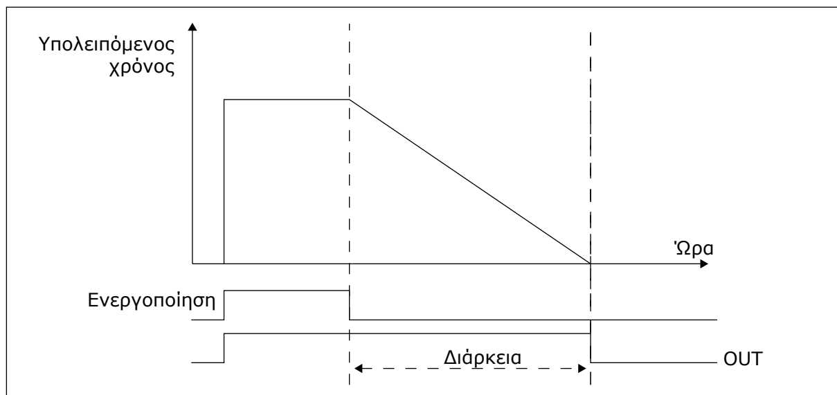
Σχ. 35: Το σήμα ενεργοποίησης προέρχεται από ψηφιακή είσοδο ή από εικονική ψηφιακή είσοδο, όπως ένα κανάλι χρόνου. Ο χρονοδιακόπτης μετρά αντίστροφα από το κατερχόμενο μέτωπο.
