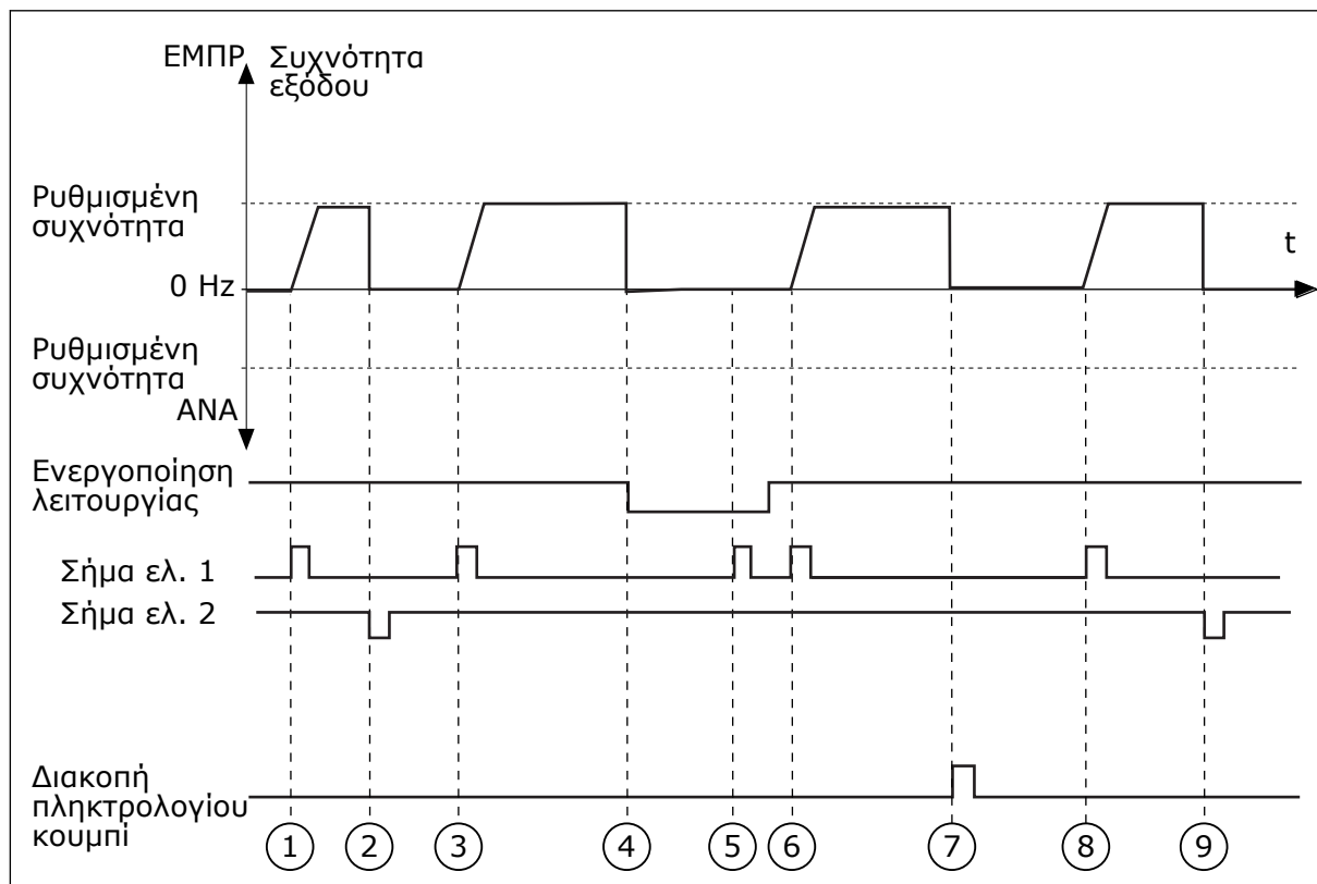
Σχ. 16: Λογική έναρξης/στάσης I / O A = 1
