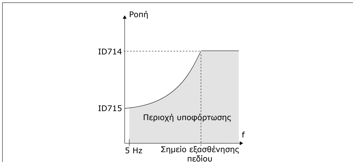
Σχ. 31: Ορισμός του ελάχιστου φορτίου
