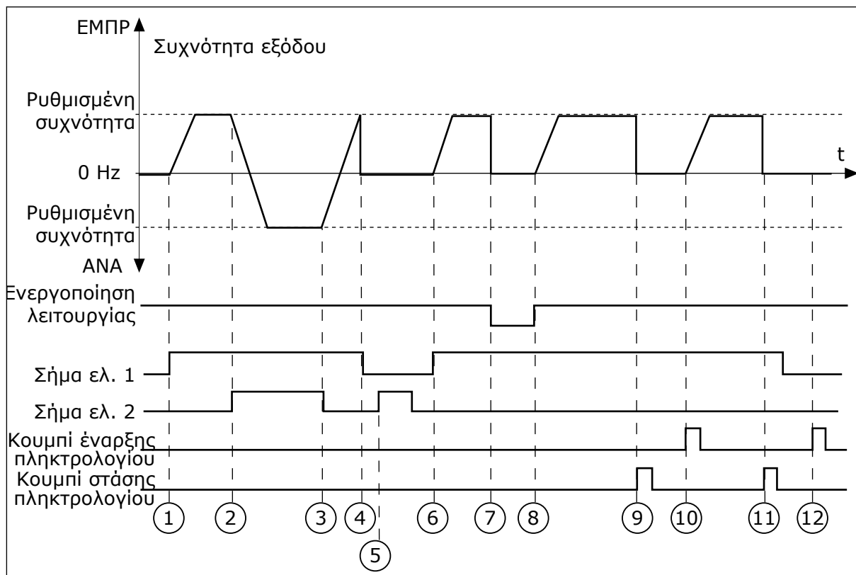
Σχ. 18: Λογική έναρξης/στάσης / t = 3
