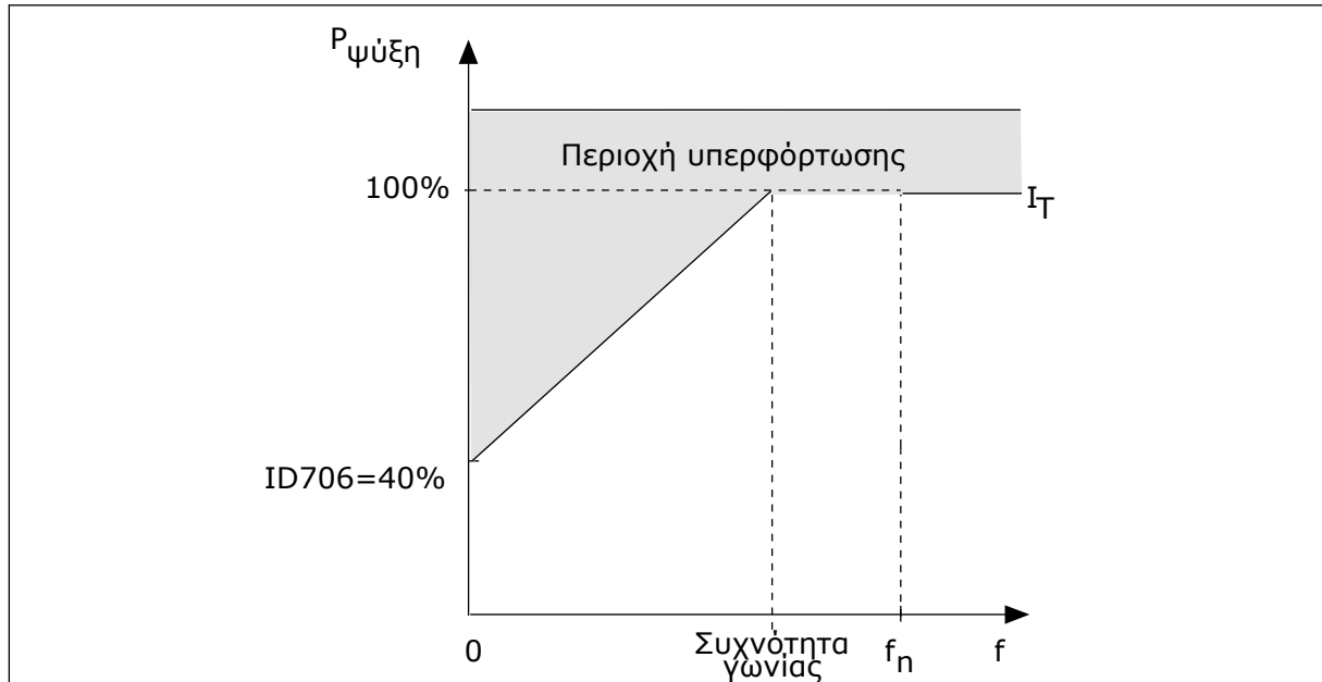
Σχ. 28: Η καμπύλη θερμικού ρεύματος κινητήρα I_T
