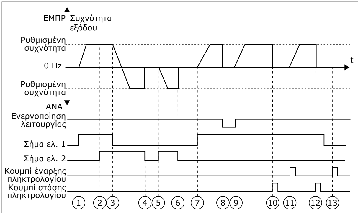
Σχ. 15: Λογική έναρξης/στάσης / O A = 0
