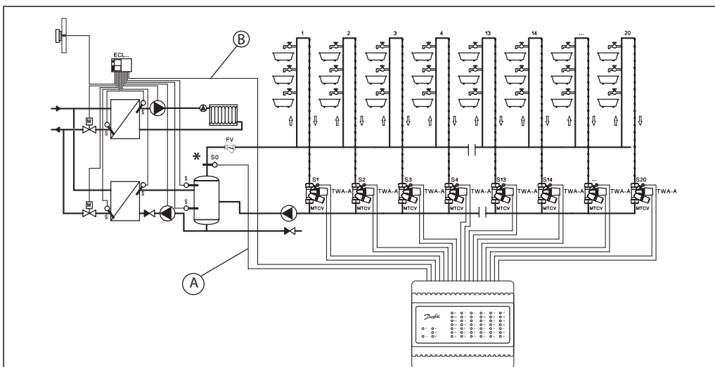
Фиг. 11. – схема на монтаж за дезинфекция и температурата на регистрация
