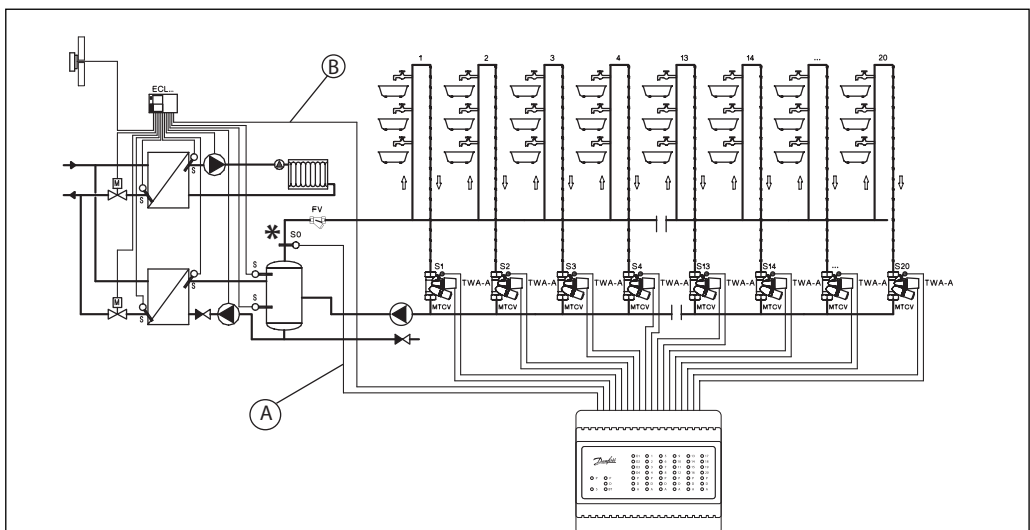
Fig. 11 – installatieschema voor desinfectie- en registratietemperatuur
