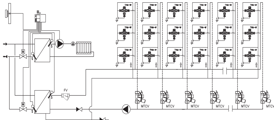
Fig. 8 Schema instalației de apă caldă cu recirculare - versiunea automată.
