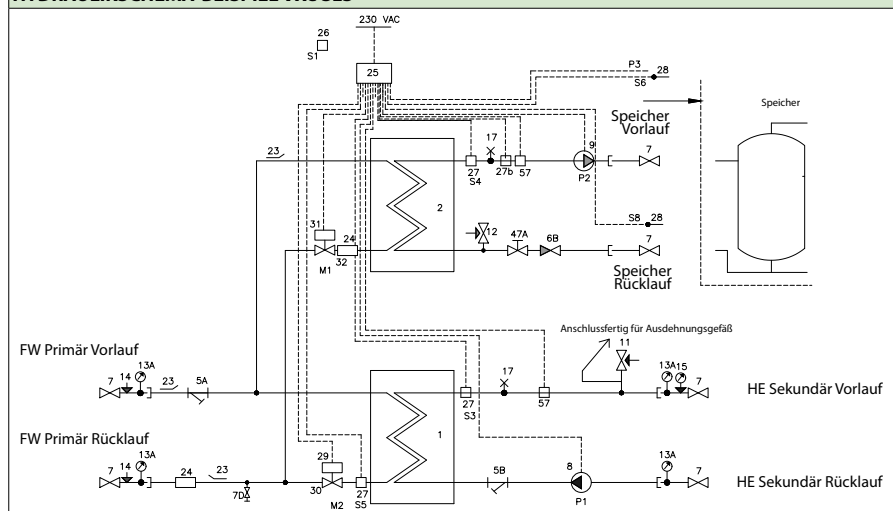
HYDRAULIKSCHEMA-BEISPIEL VXe SLS
