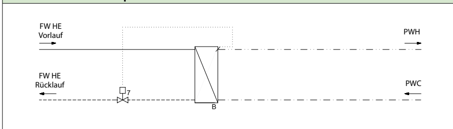
Termix One-B mit Sicherheitsventil
