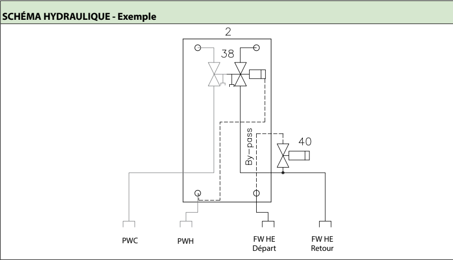
2 Échangeur de chaleur à plaques XB06H-1 ... 38 Redan PTC2+P-Régulateur 40 Danfoss F JVR pour bypass/PWH-C.
