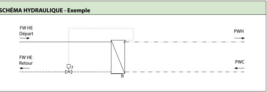
Termix One avec soupape de sécurité B Échangeur de chaleur à plaques PWH 7 Régulateur de température thermostatique
